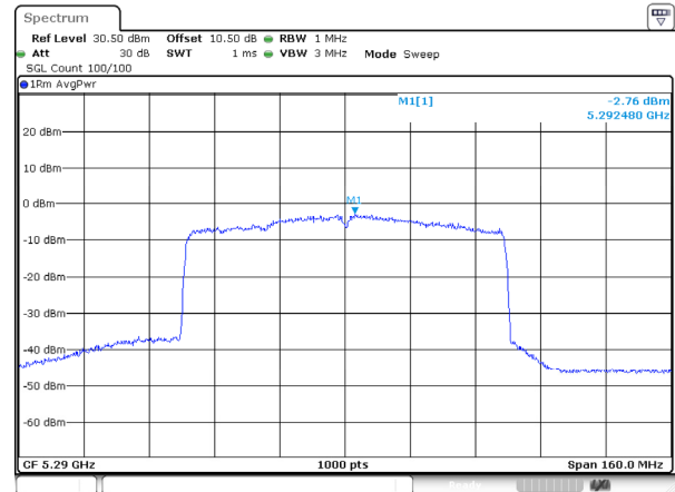
802.11ax80_5290MHz_RU_FULL_Ant 1
