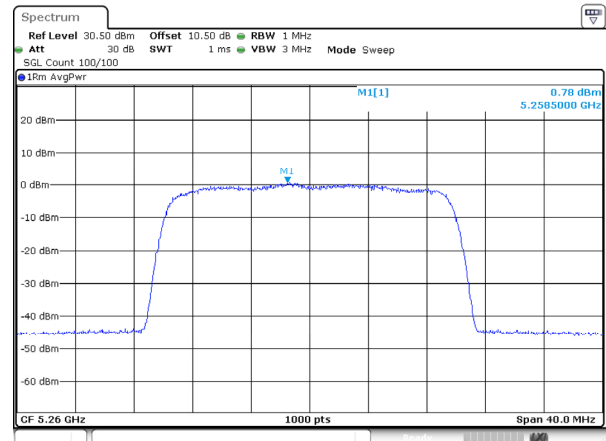
802.11be20_5260MHz_RU_FULL_Ant 1
