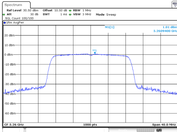
802.11ac20_5260MHz_Ant 2
