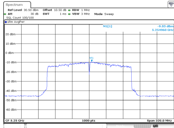
802.11be160_5250MHz_RU_FULL_Ant 1
