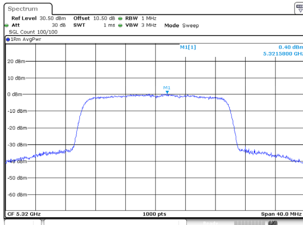
802.11be20_5320MHz_RU_FULL_Ant 0
