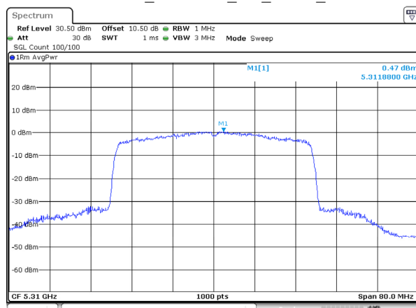
802.11be40_5310MHz_RU_FULL_Ant 0
