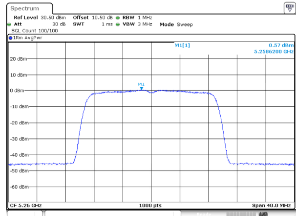
802.11ac20_5260MHz_Ant 1
