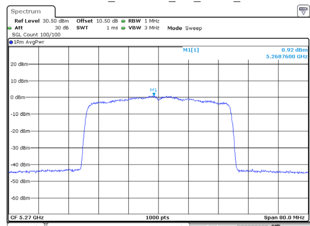
802.11be40_5270MHz_RU_FULL_Ant 1
