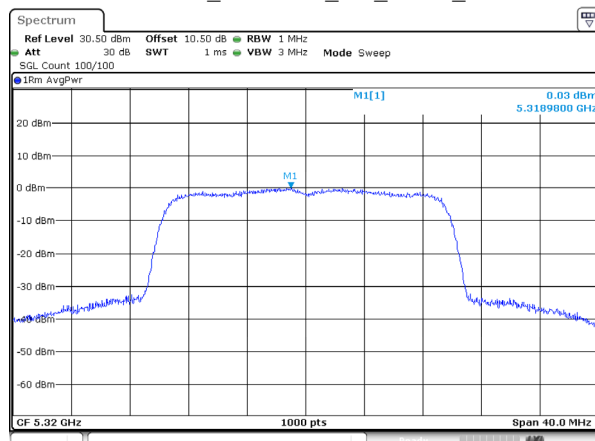
802.11be20_5320MHz_RU_FULL_Ant 2
