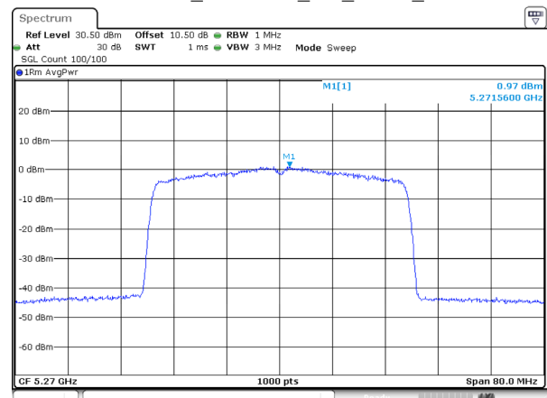
802.11be40_5270MHz_RU_FULL_Ant 0
