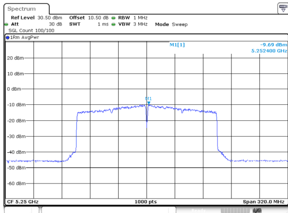
802.11be160_5250MHz_RU_FULL_Ant 2
