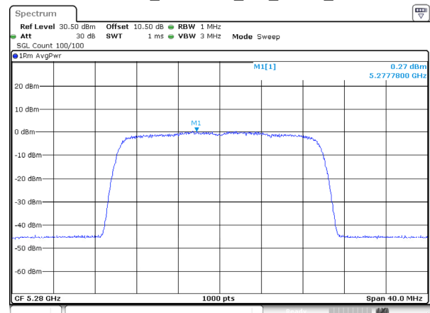
802.11be20_5280MHz_RU_FULL_Ant 2
