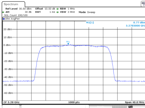
802.11be20_5280MHz_RU_FULL_Ant 1
