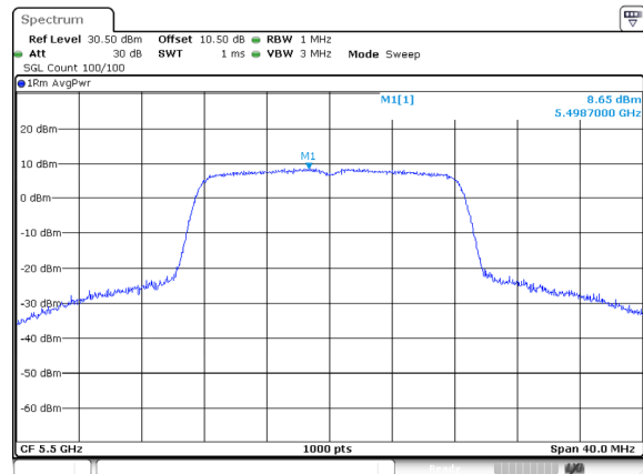
802.11a_5500MHz_Ant 0
