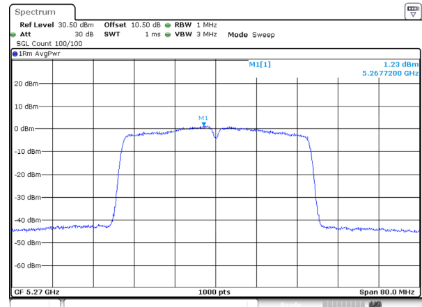
802.11ac40_5270MHz_Ant 0
