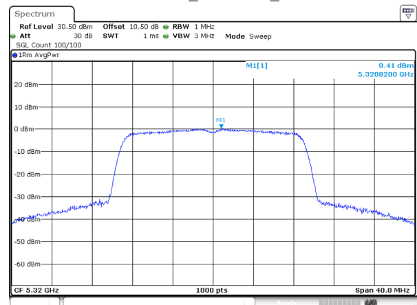
802.11ac20_5320MHz_Ant 1
