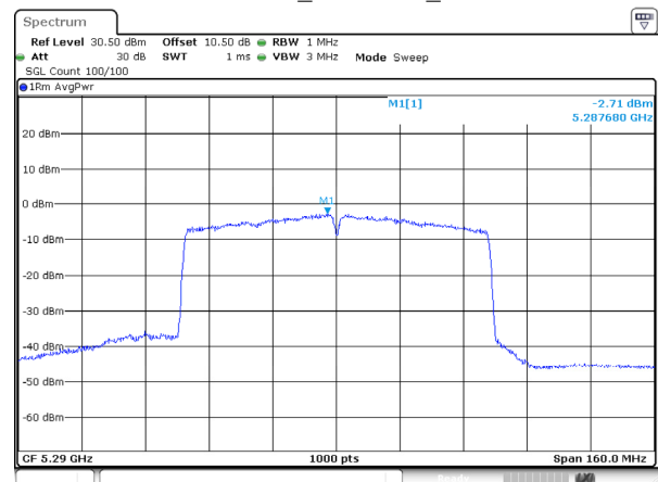
802.11ac80_5290MHz_Ant 2
