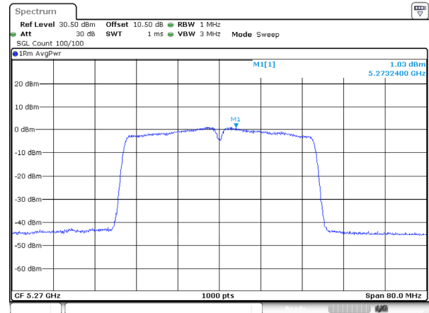
802.11ac40_5270MHz_Ant 2
