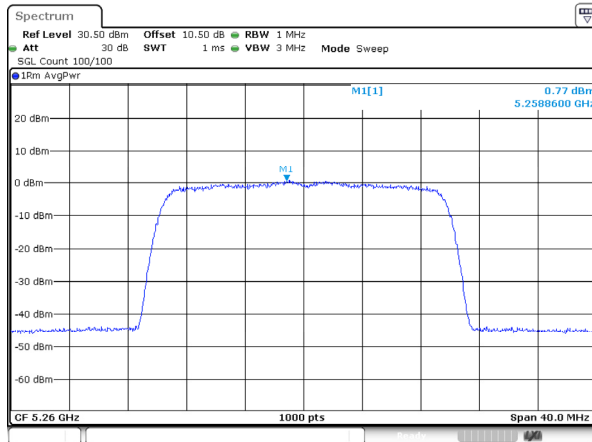
802.11be20_5260MHz_RU_FULL_Ant 0
