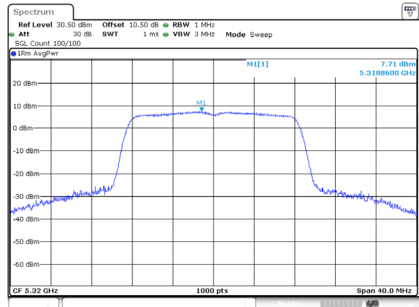
802.11a_5320MHz_Ant 2
