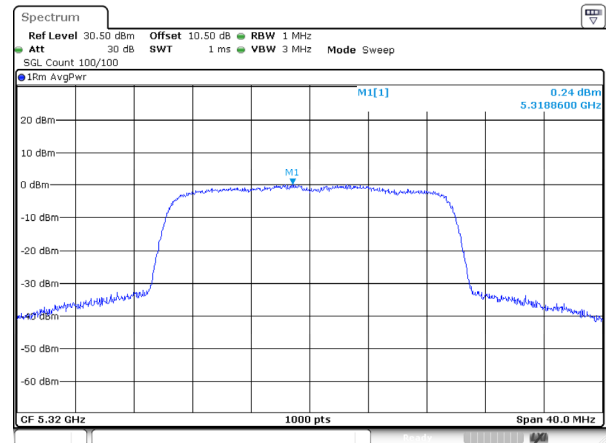
802.11be20_5320MHz_RU_FULL_Ant 1
