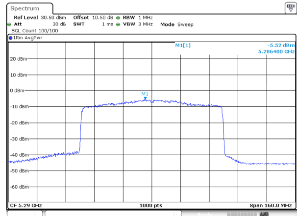
802.11be80_5290MHz_RU_FULL_Ant 0
