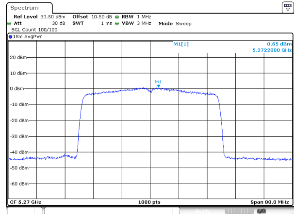
802.11be40_5270MHz_RU_FULL_Ant 2
