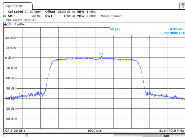
802.11be20_5260MHz_RU_FULL_Ant 2
