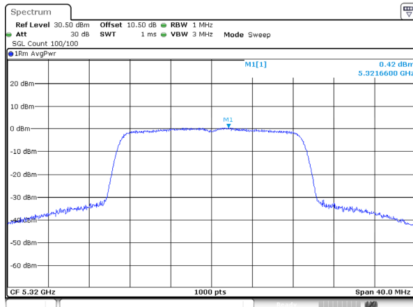
802.11ac20_5320MHz_Ant 2
