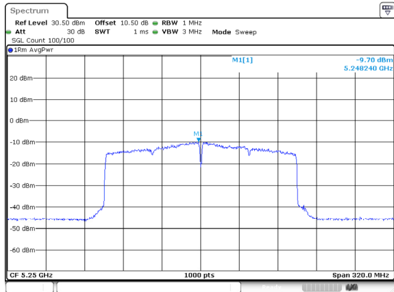
802.11be160_5250MHz_RU_FULL_Ant 0
