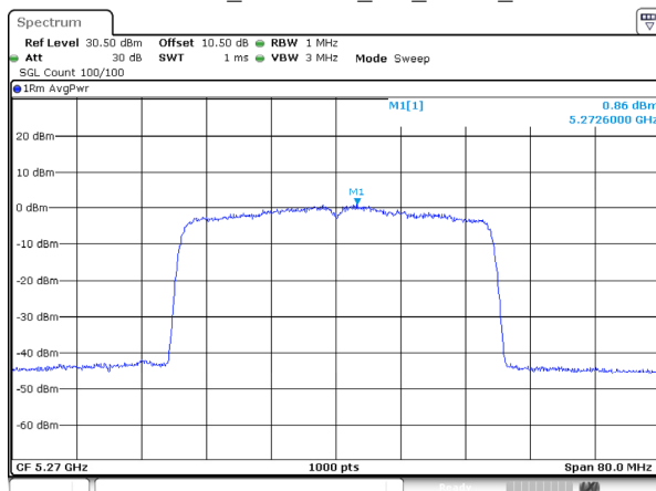
802.11ax40_5270MHz_RU_FULL_Ant 2
