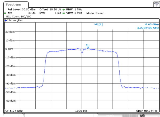
802.11ac40_5270MHz_Ant 1
