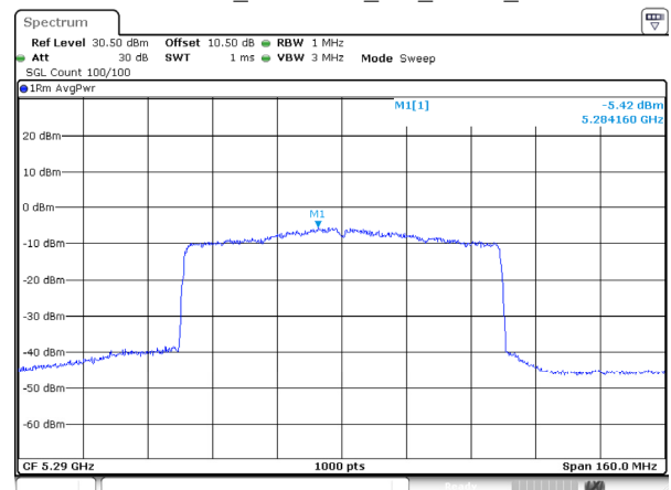
802.11be80_5290MHz_RU_FULL_Ant 2
