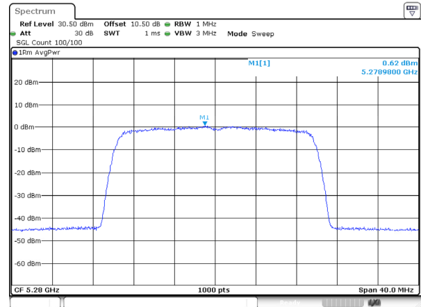
802.11be20_5280MHz_RU_FULL_Ant 0
