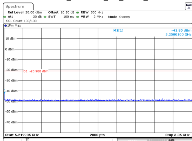
802.11be20_5240MHz_RU_FULL_Ant 2
