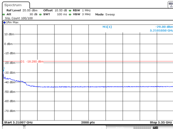
802.11be40_5190MHz_RU_FULL_Ant 1
