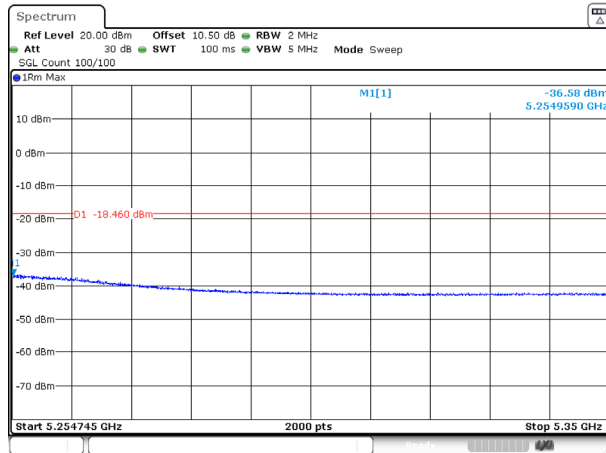
802.11ac80_5210MHz_Ant 0
