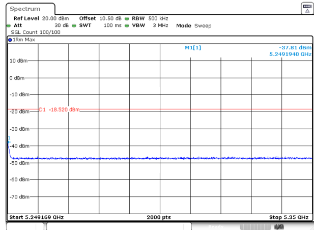
802.11ac40_5230MHz_Ant 1
