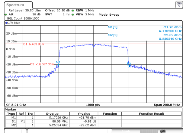
802.11ac80_5210MHz_Ant 1
