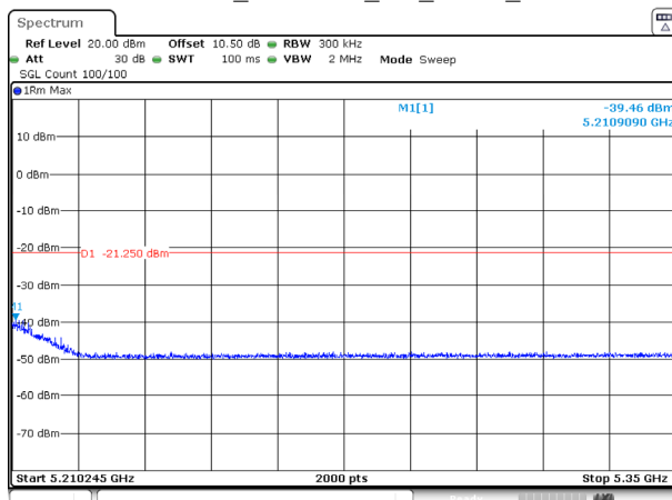
802.11be20_5200MHz_RU_FULL_Ant 2
