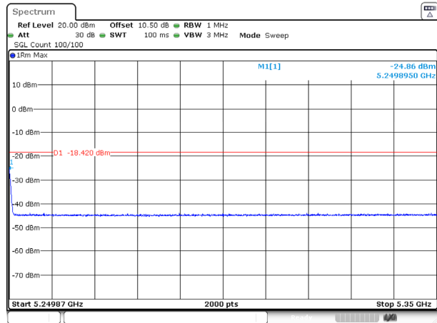
802.11ax40_5230MHz_RU_FULL_Ant 0
