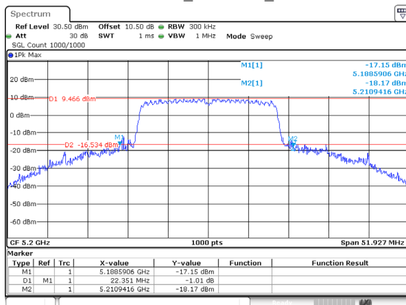
802.11ac20_5200MHz_Ant 2
