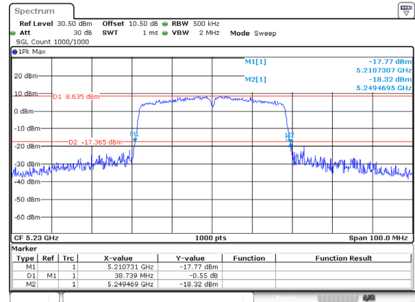
802.11ac40_5230MHz_Ant 0
