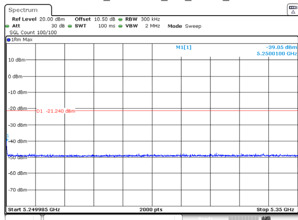
802.11be20_5240MHz_RU_FULL_Ant 0
