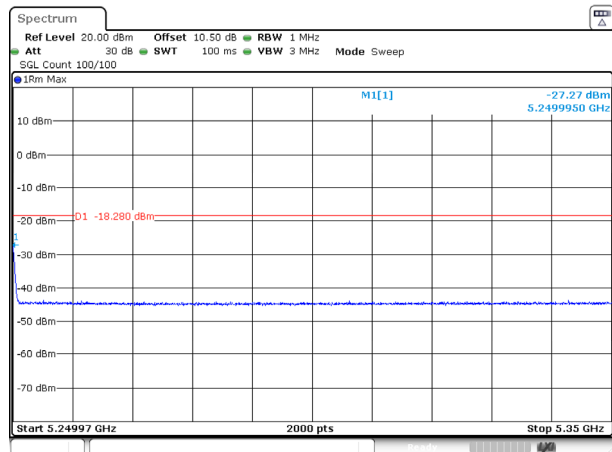
802.11ax40_5230MHz_RU_FULL_Ant 2
