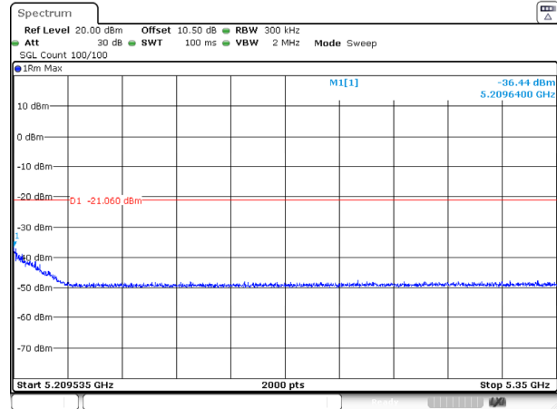
802.11ac20_5200MHz_Ant 1
