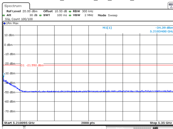
802.11be20_5200MHz_RU_FULL_Ant 0
