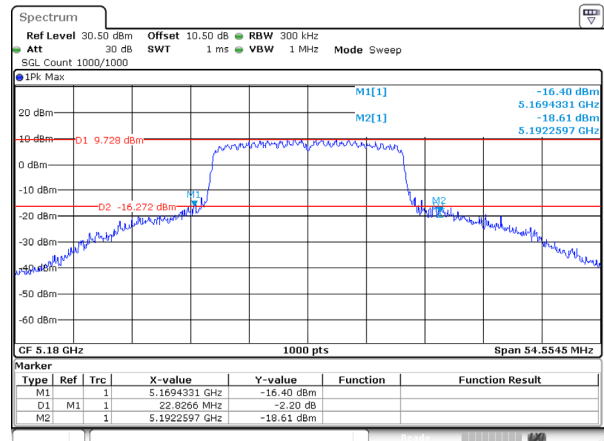
802.11ac20_5180MHz_Ant 2
