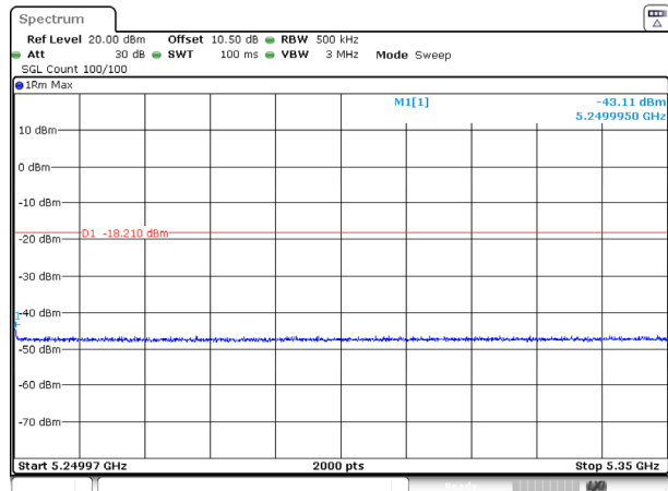
802.11be40_5230MHz_RU_FULL_Ant 1
