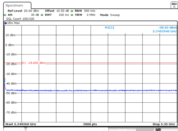
802.11ac40_5230MHz_Ant 2
