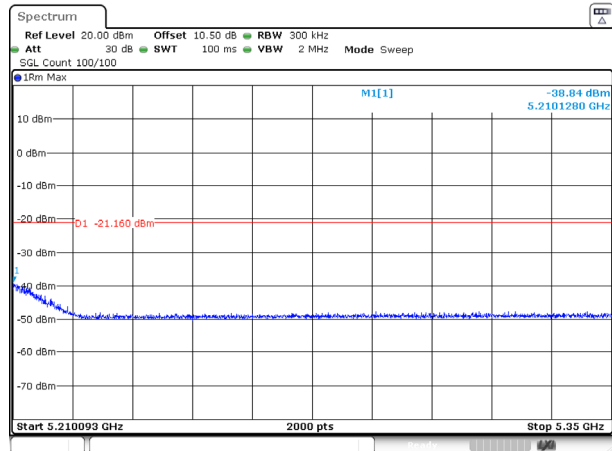
802.11be20_5200MHz_RU_FULL_Ant 1
