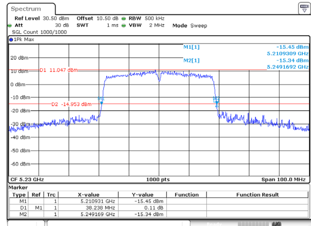
802.11ac40_5230MHz_Ant 1
