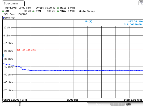
802.11be40_5190MHz_RU_FULL_Ant 0
