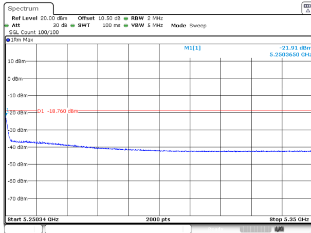
802.11ax80_5210MHz_RU_FULL_Ant 0
