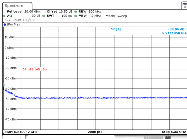
802.11ac20_5200MHz_Ant 2
