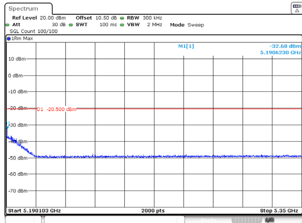
802.11be20_5180MHz_RU_FULL_Ant 0
