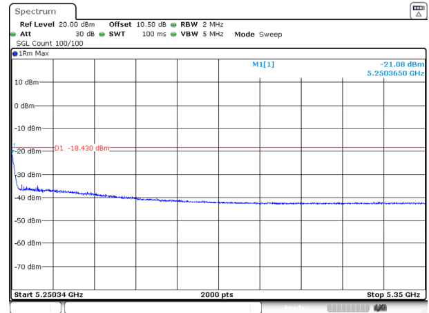
802.11be80_5210MHz_RU_FULL_Ant 1
