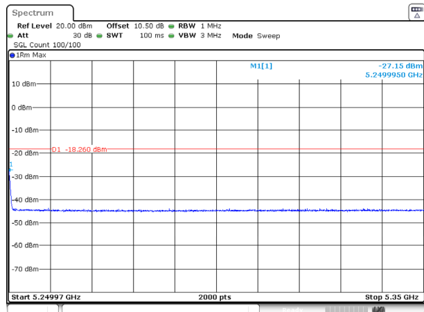
802.11be40_5230MHz_RU_FULL_Ant 2
