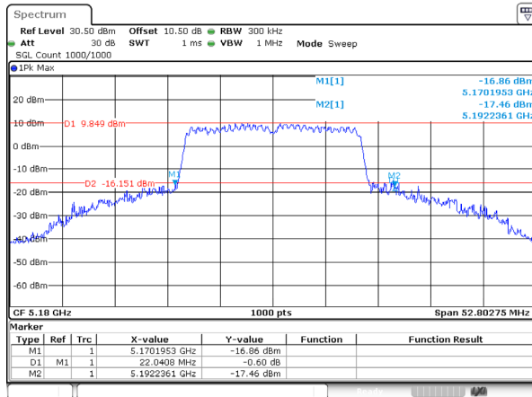
802.11ac20_5180MHz_Ant 1
