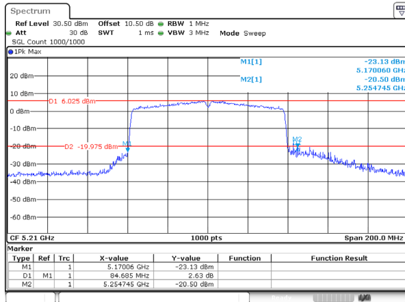
802.11ac80_5210MHz_Ant 0
