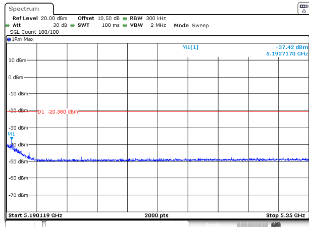
802.11be20_5180MHz_RU_FULL_Ant 2
