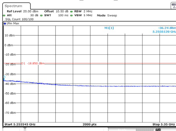
802.11ac80_5210MHz_Ant 2
