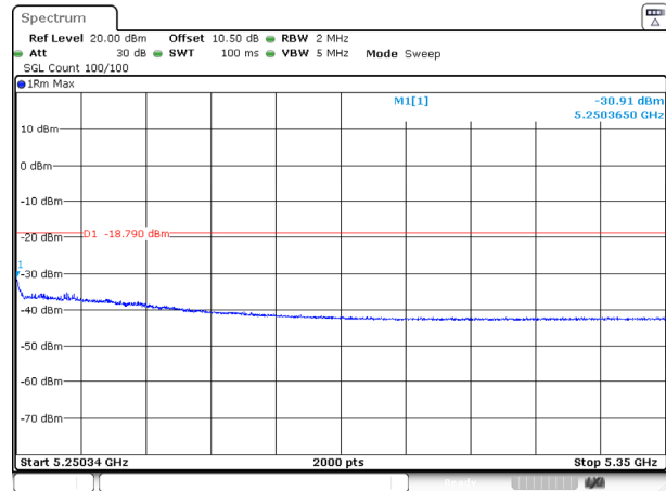
802.11ac80_5210MHz_Ant 1
