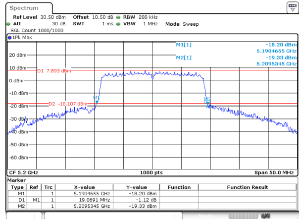
802.11ac20_5200MHz_Ant 1
