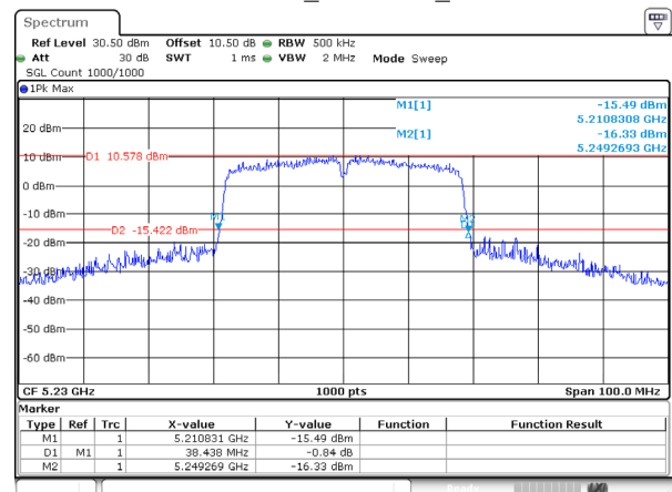
802.11ac40_5230MHz_Ant 2
