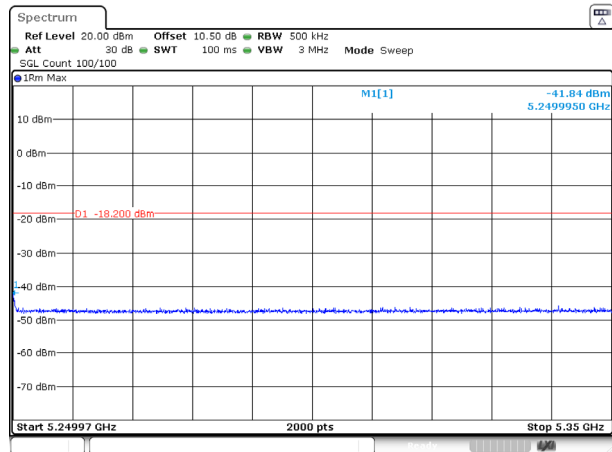
802.11ax40_5230MHz_RU_FULL_Ant 1
