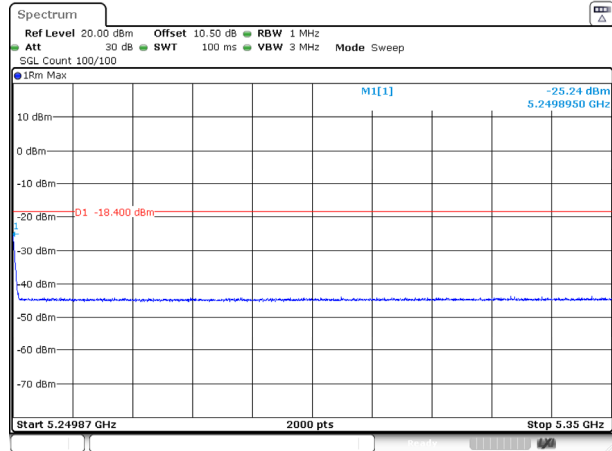
802.11be40_5230MHz_RU_FULL_Ant 0
