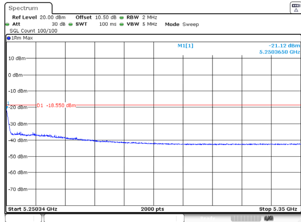
802.11ax80_5210MHz_RU_FULL_Ant 1
