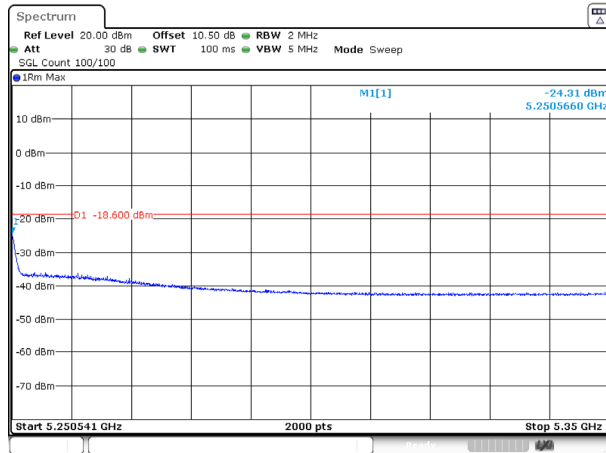
802.11be80_5210MHz_RU_FULL_Ant 0
