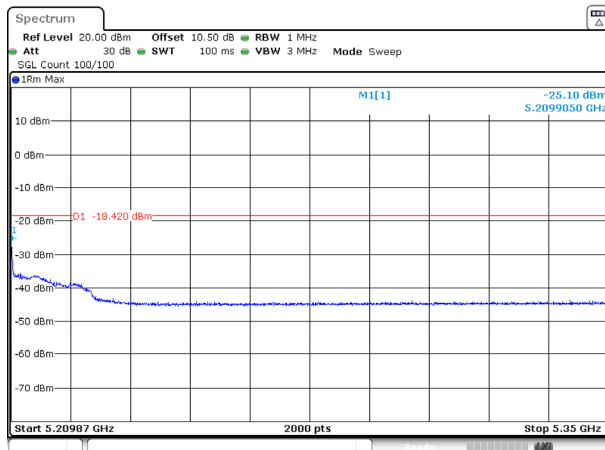
802.11be40_5190MHz_RU_FULL_Ant 2
