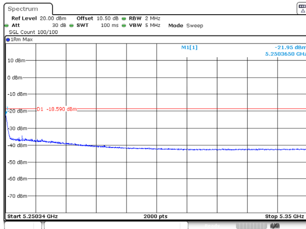
802.11ax80_5210MHz_RU_FULL_Ant 2
