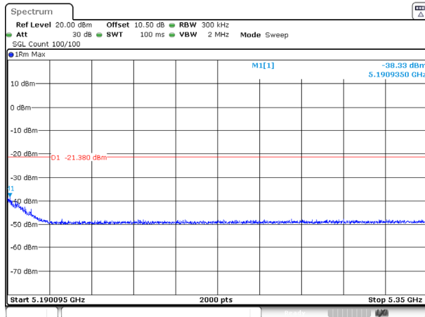
802.11be20_5180MHz_RU_FULL_Ant 1
