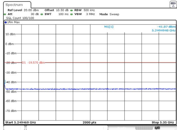
802.11ac40_5230MHz_Ant 0
