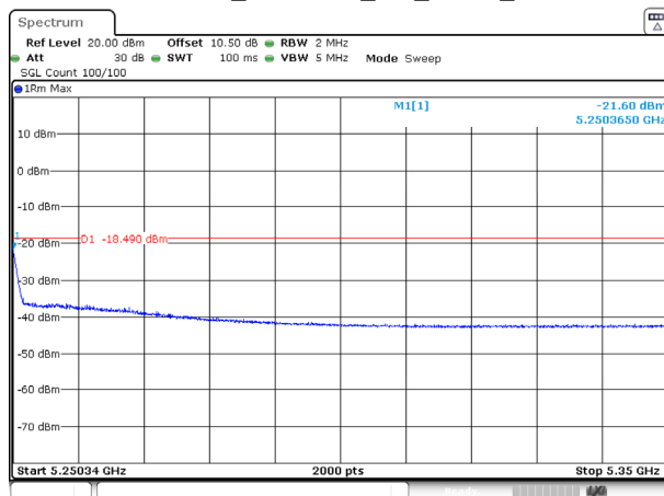
802.11be80_5210MHz_RU_FULL_Ant 2
