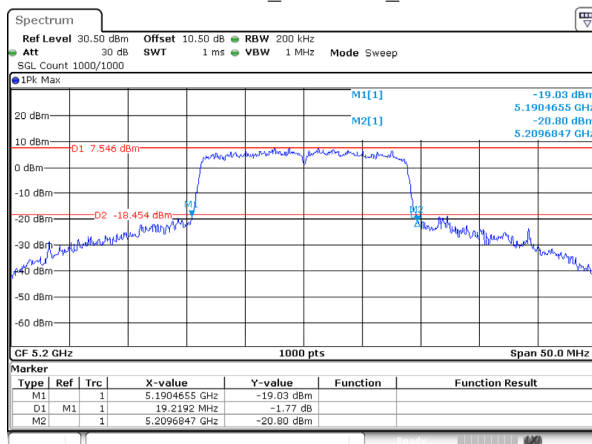
802.11ac20_5200MHz_Ant 0
