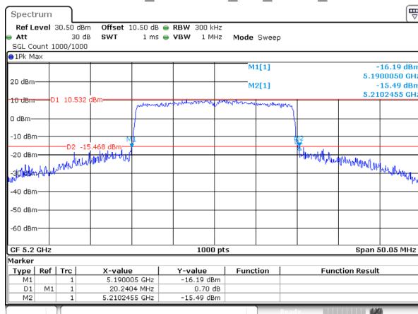
802.11be20_5200MHz_RU_FULL_Ant 2
