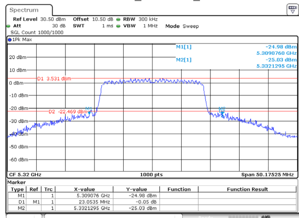
802.11ac20_5320MHz_Ant 1
