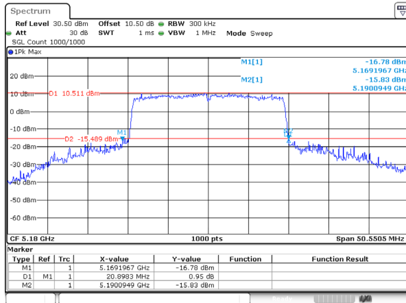
802.11be20_5180MHz_RU_FULL_Ant 1
