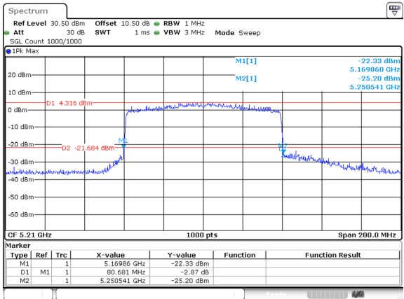
802.11be80_5210MHz_RU_FULL_Ant 0
