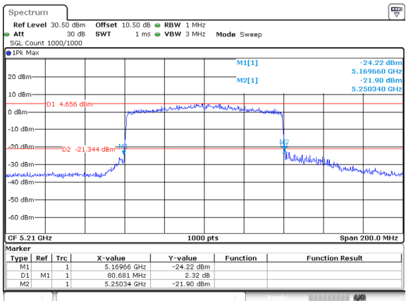
802.11be80_5210MHz_RU_FULL_Ant 2
