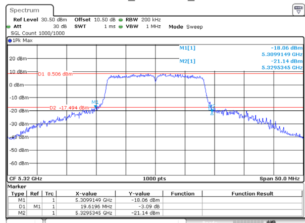
802.11a_5320MHz_Ant 2
