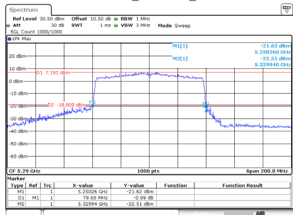
802.11ac80_5290MHz_Ant 2
