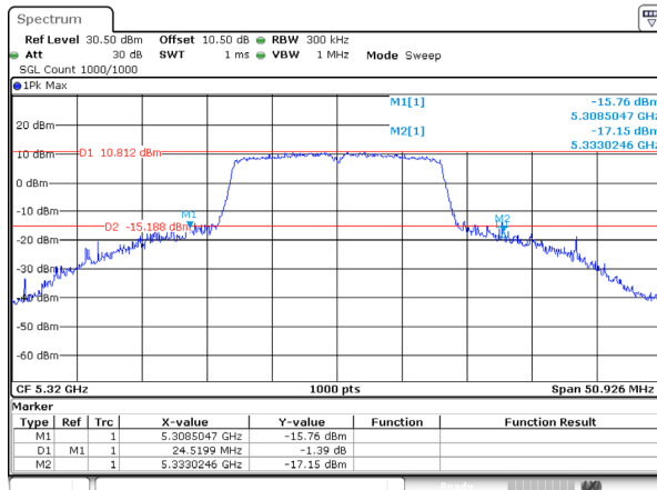
802.11a_5320MHz_Ant 1
