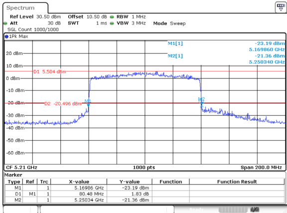
802.11be80_5210MHz_RU_FULL_Ant 1
