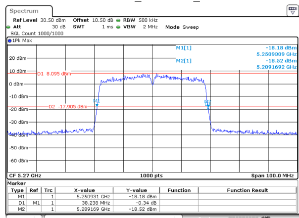
802.11ac40_5270MHz_Ant 1
