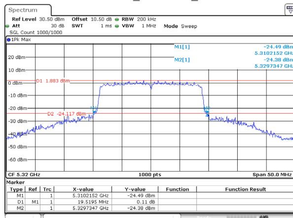
802.11ac20_5320MHz_Ant 2
