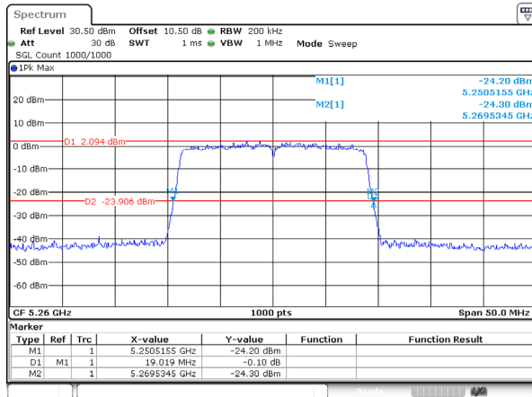
802.11ac20_5260MHz_Ant 0
