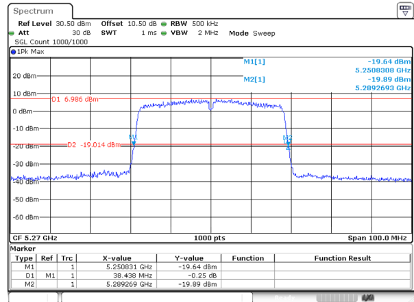
802.11ac40_5270MHz_Ant 2
