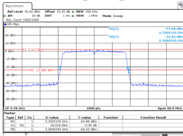
802.11ac20_5260MHz_Ant 2
