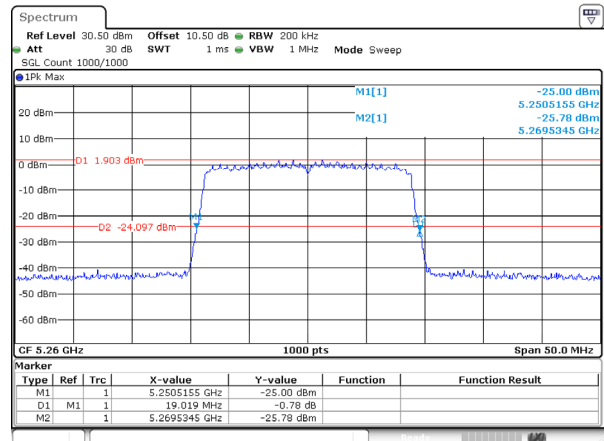
802.11ac20_5260MHz_Ant 1
