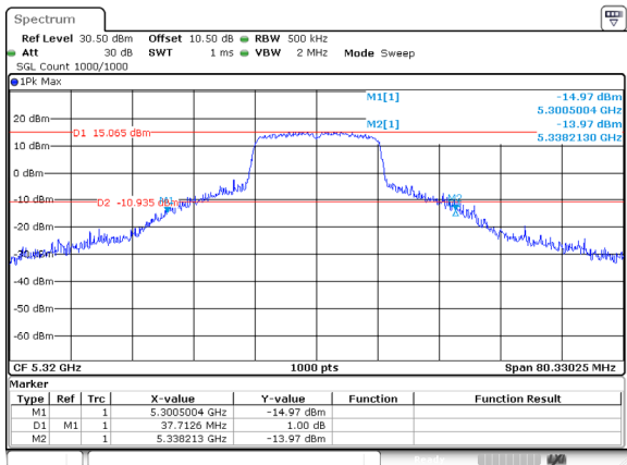
802.11a_5320MHz_Ant 0
