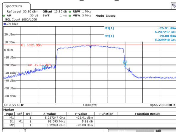
802.11ac80_5290MHz_Ant 1
