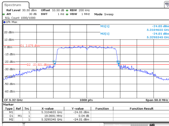
802.11ac20_5320MHz_Ant 0
