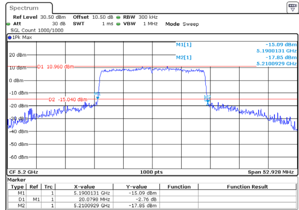
802.11be20_5200MHz_RU_FULL_Ant 1
