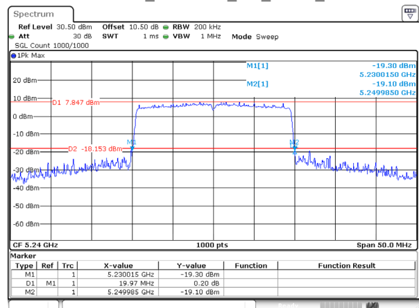
802.11be20_5240MHz_RU_FULL_Ant 2
