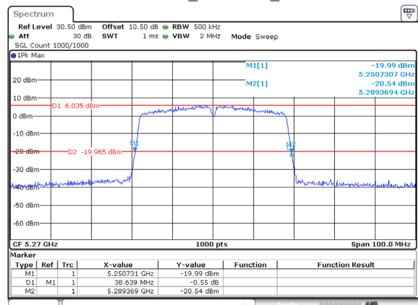
802.11ac40_5270MHz_Ant 0
