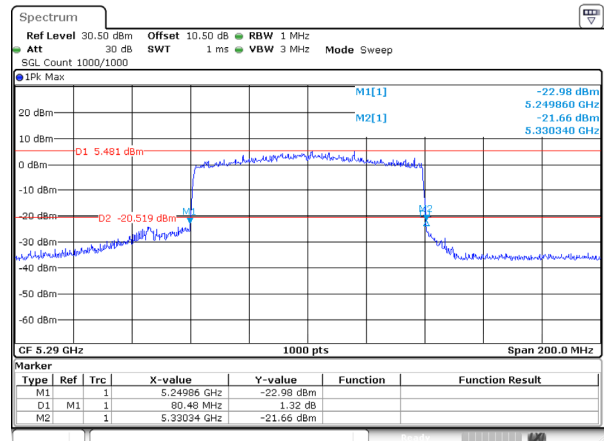
802.11be80_5290MHz_RU_FULL_Ant 0
