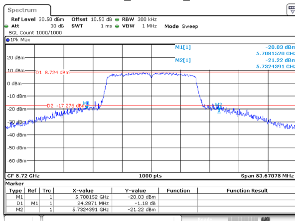
802.11a_5720MHz_Ant 1
