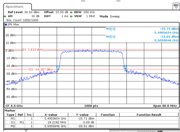
802.11ac20_5500MHz_Ant 2
