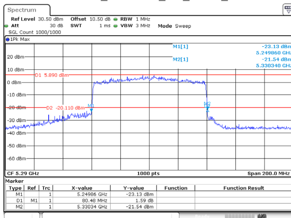
802.11be80_5290MHz_RU_FULL_Ant 1
