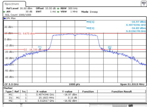
802.11a_5500MHz_Ant 1
