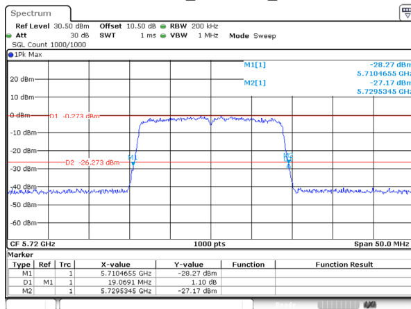
802.11ac20_5720MHz_Ant 0
