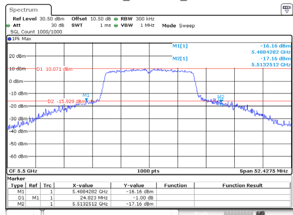
802.11a_5500MHz_Ant 2
