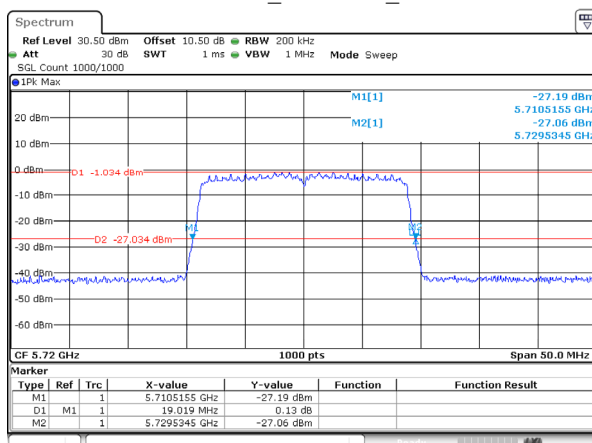
802.11ac20_5720MHz_Ant 1
