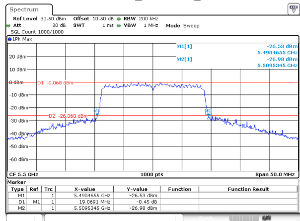
802.11ac20_5500MHz_Ant 1
