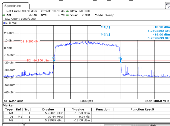
802.11ax40_5270MHz_RU_FULL_Ant 2
