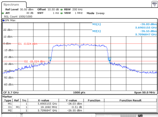
802.11ac20_5700MHz_Ant 0
