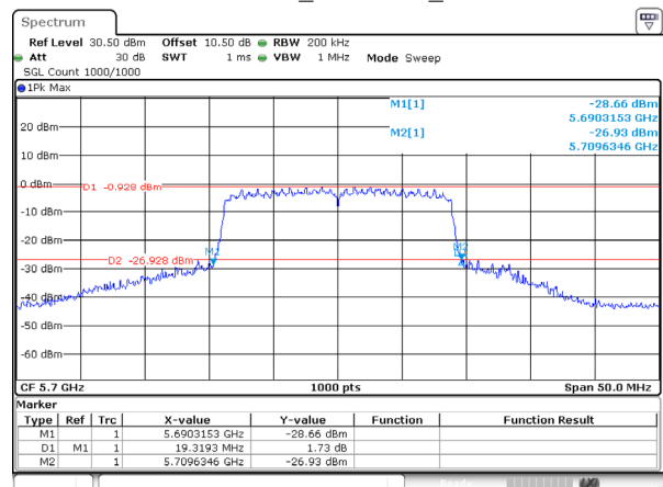
802.11ac20_5700MHz_Ant 1
