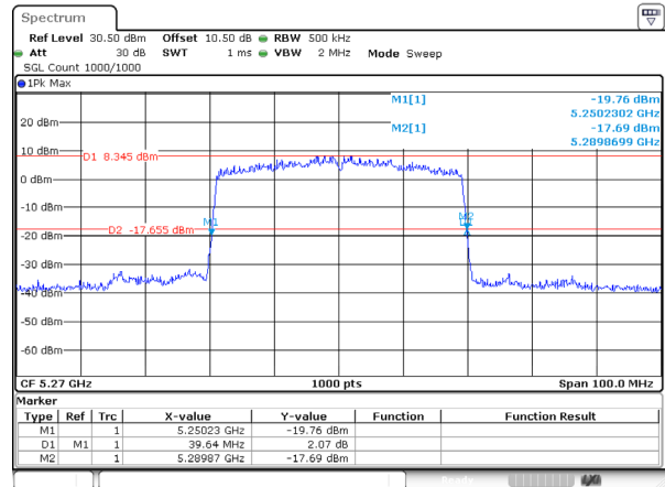
802.11be40_5270MHz_RU_FULL_Ant 2
