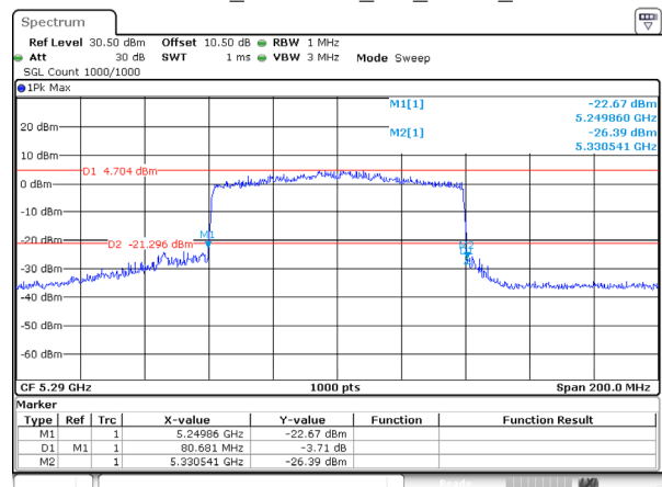
802.11be80_5290MHz_RU_FULL_Ant 2
