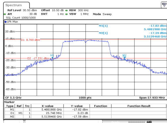
802.11a_5500MHz_Ant 0
