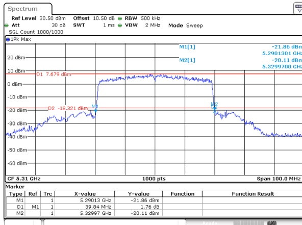
802.11be40_5310MHz_RU_FULL_Ant 2
