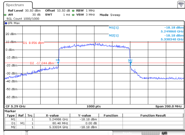
802.11ax80_5290MHz_RU_FULL_Ant 1
