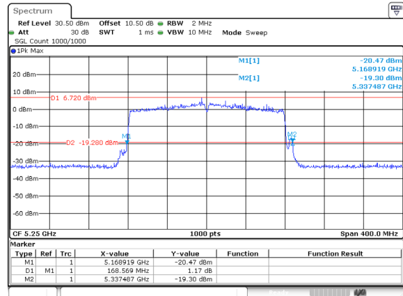
802.11be160_5250MHz_RU_FULL_Ant 1
