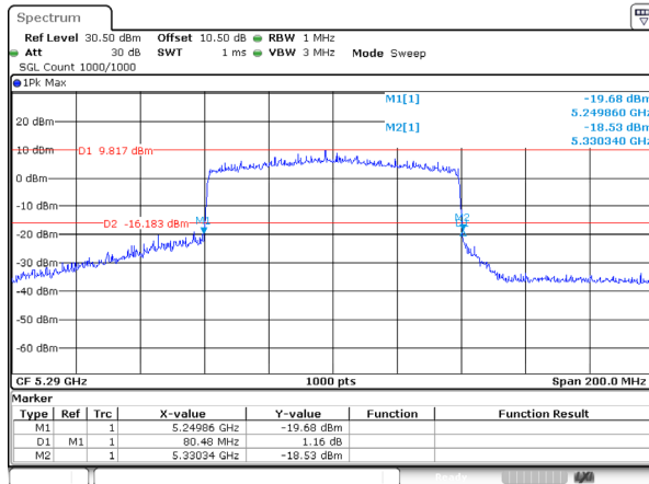
802.11ax80_5290MHz_RU_FULL_Ant 0
