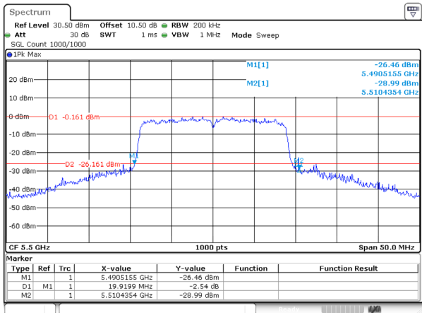
802.11ac20_5500MHz_Ant 0
