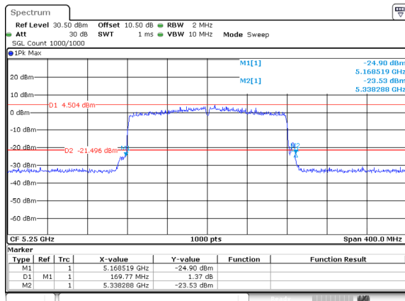
802.11be160_5250MHz_RU_FULL_Ant 2
