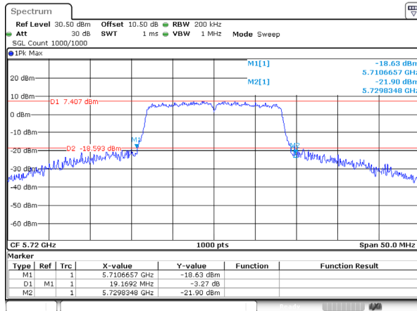
802.11a_5720MHz_Ant 0
