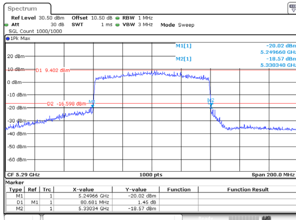
802.11ax80_5290MHz_RU_FULL_Ant 2
