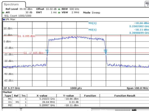
802.11ax40_5270MHz_RU_FULL_Ant 1
