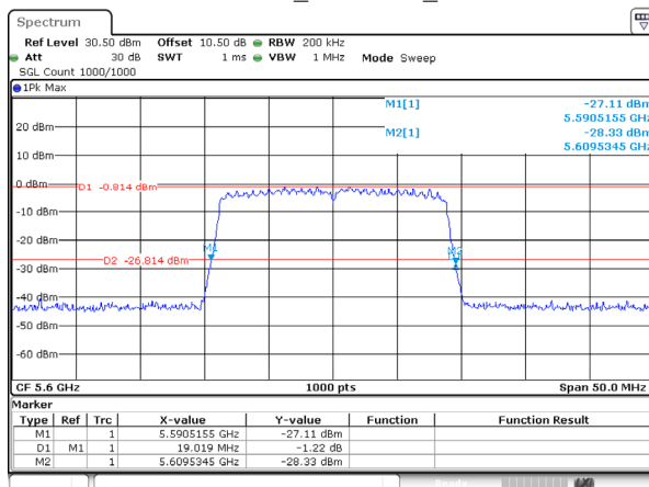
802.11ac20_5600MHz_Ant 1
