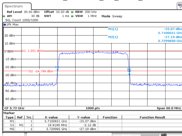
802.11ax20_5720MHz_RU_FULL_Ant 1
