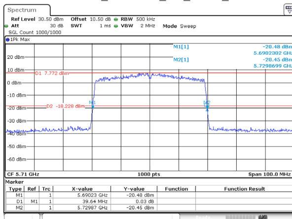
802.11be40_5710MHz_RU_FULL_Ant 1
