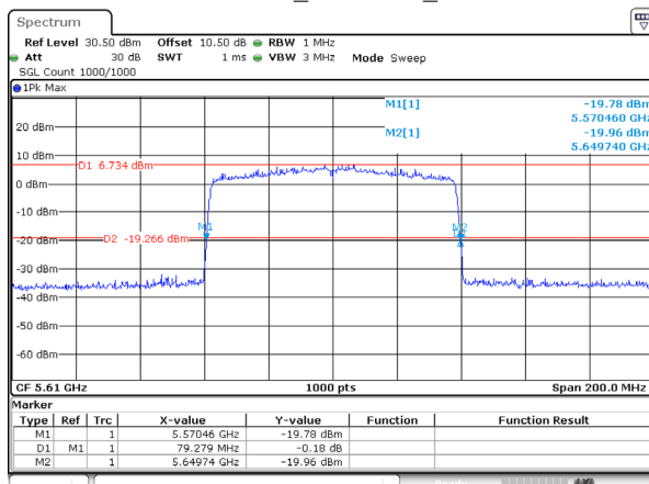
802.11ac80_5610MHz_Ant 2
