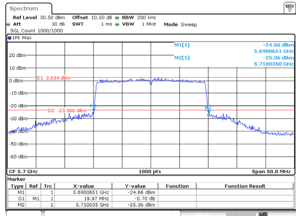
802.11be20_5700MHz_RU_FULL_Ant 1
