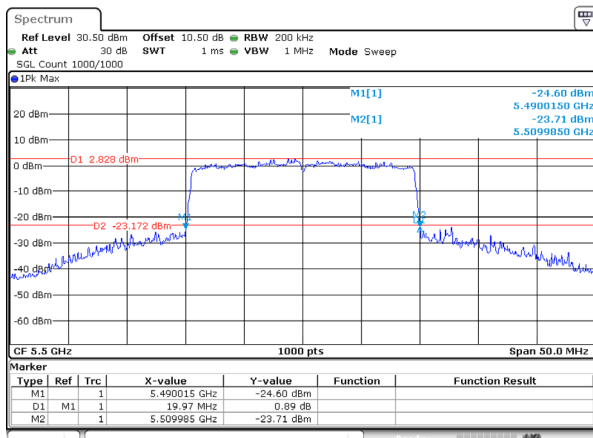
802.11be20_5500MHz_RU_FULL_Ant 0
