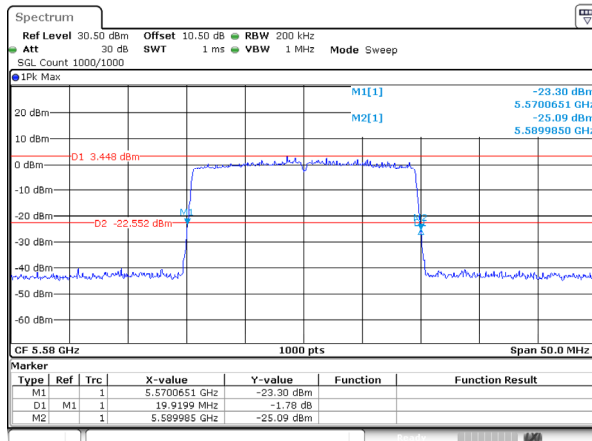
802.11be20_5580MHz_RU_FULL_Ant 1
