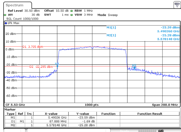
802.11ac80_5530MHz_Ant 0
