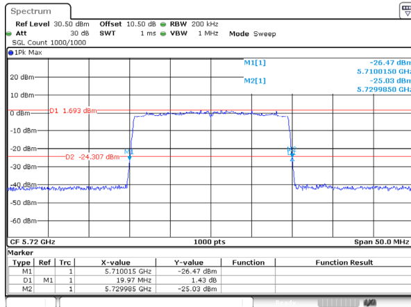
802.11be20_5720MHz_RU_FULL_Ant 0
