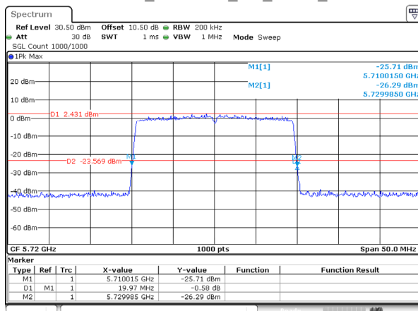
802.11be20_5720MHz_RU_FULL_Ant 1
