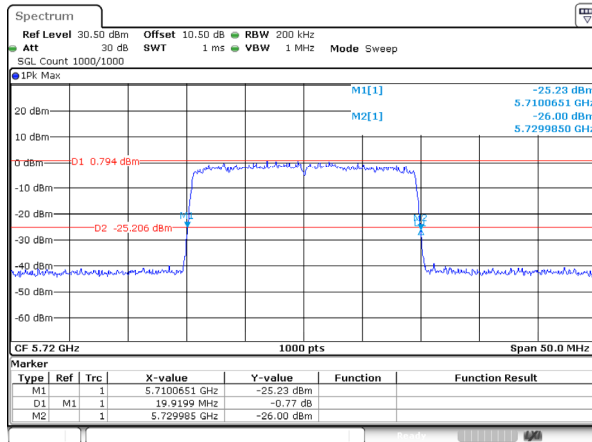
802.11ax20_5720MHz_RU_FULL_Ant 0
