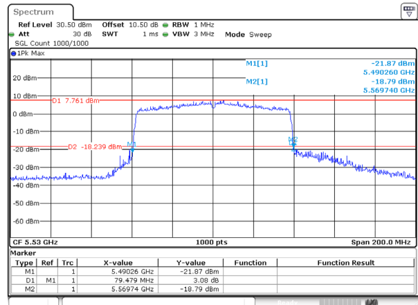
802.11ac80_5530MHz_Ant 2
