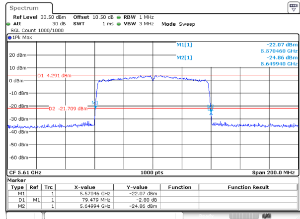
802.11ac80_5610MHz_Ant 1
