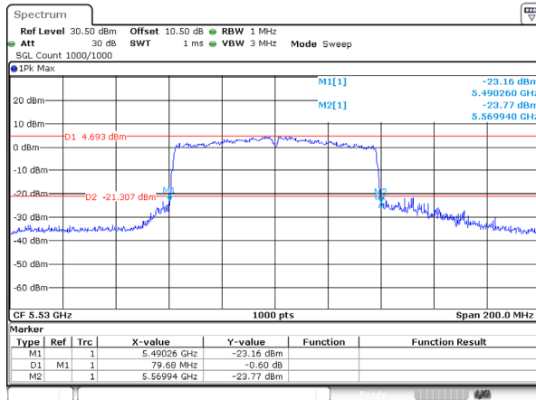
802.11ac80_5530MHz_Ant 1
