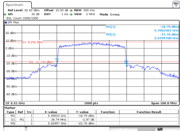
802.11be40_5510MHz_RU_FULL_Ant 1
