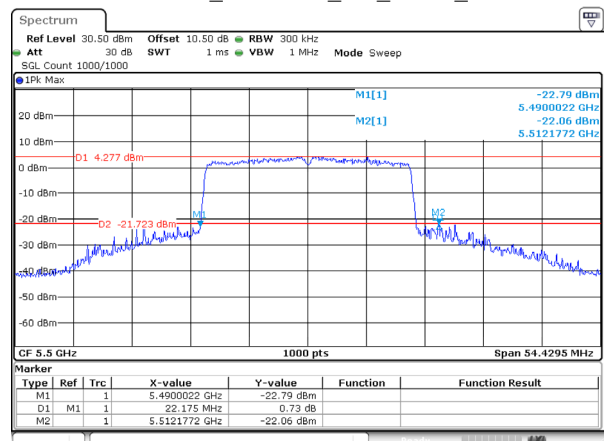
802.11be20_5500MHz_RU_FULL_Ant 2
