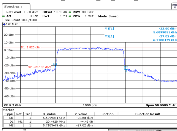
802.11be20_5700MHz_RU_FULL_Ant 0
