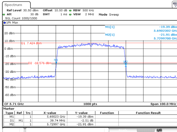
802.11be40_5710MHz_RU_FULL_Ant 0
