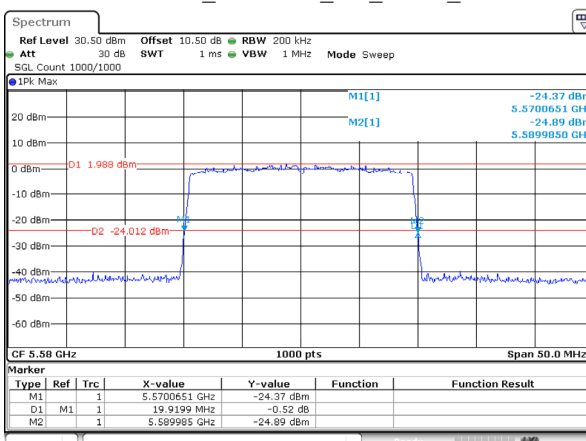
802.11be20_5580MHz_RU_FULL_Ant 0
