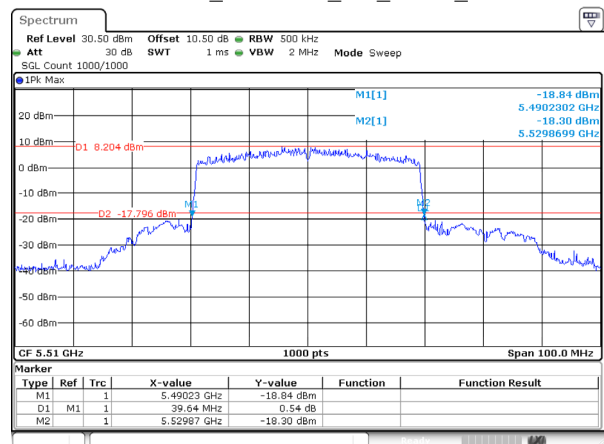
802.11be40_5510MHz_RU_FULL_Ant 2
