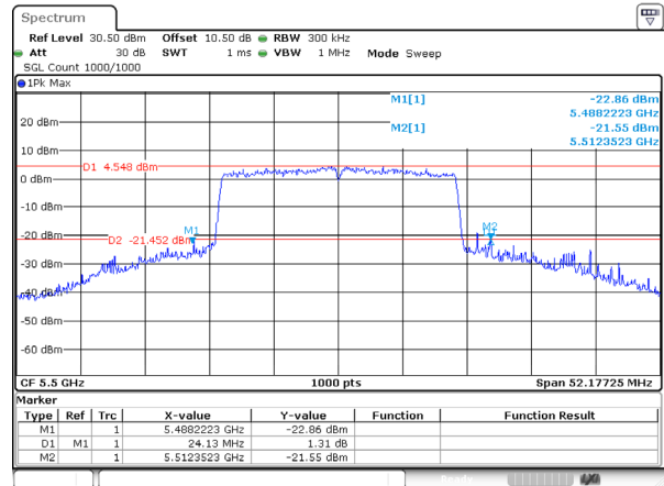
802.11be20_5500MHz_RU_FULL_Ant 1
