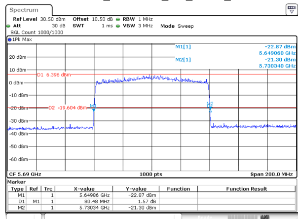
802.11be80_5690MHz_RU_FULL_Ant 2
