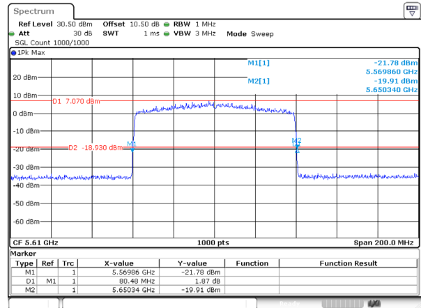
802.11be80_5610MHz_RU_FULL_Ant 1
