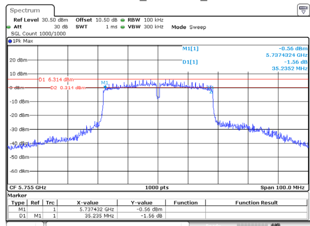
802.11ac40_5755MHz_Ant 1
