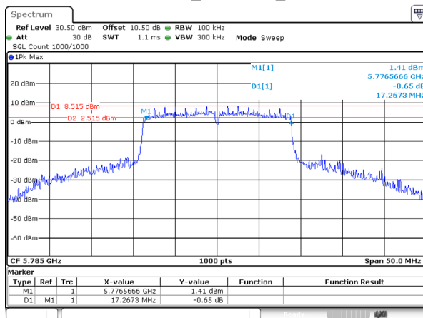
802.11ac20_5785MHz_Ant 1
