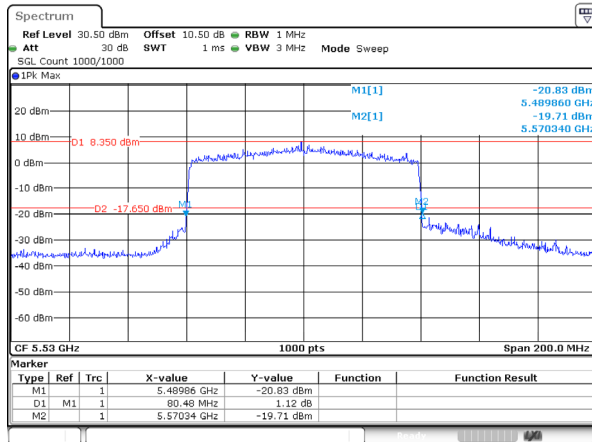
802.11be80_5530MHz_RU_FULL_Ant 1
