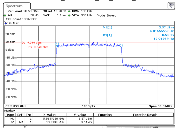
802.11be20_5825MHz_RU_FULL_Ant 1
