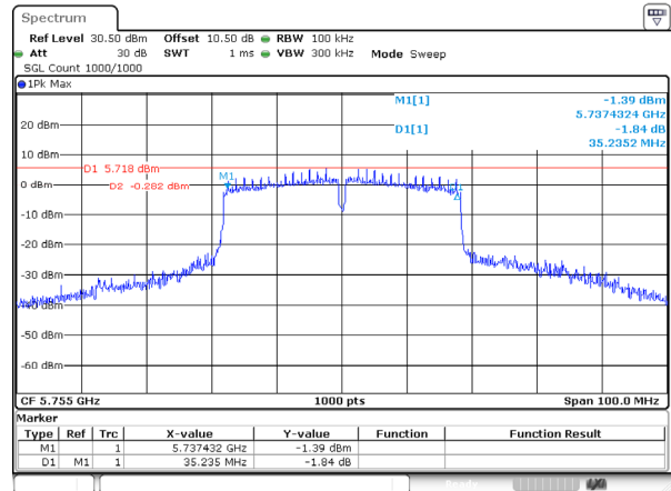
802.11ac40_5755MHz_Ant 2
