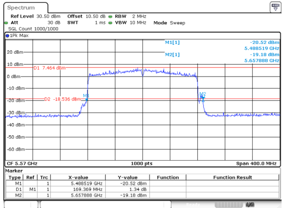
802.11be160_5570MHz_RU_FULL_Ant 0
