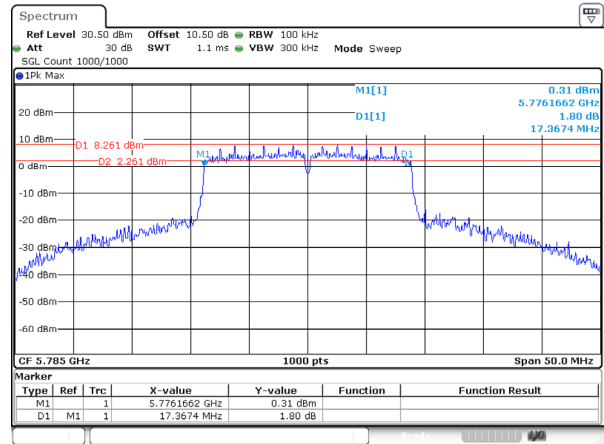
802.11ac20_5785MHz_Ant 0
