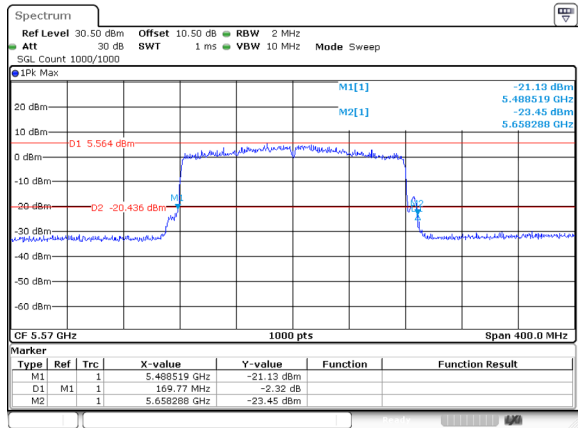
802.11be160_5570MHz_RU_FULL_Ant 2
