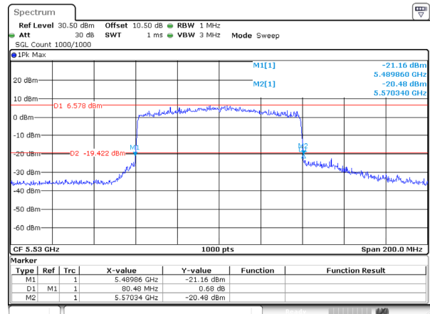
802.11be80_5530MHz_RU_FULL_Ant 2
