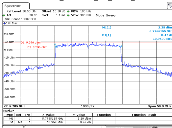
802.11be20_5785MHz_RU_FULL_Ant 1
