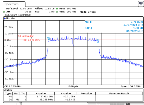
802.11ac40_5755MHz_Ant 0
