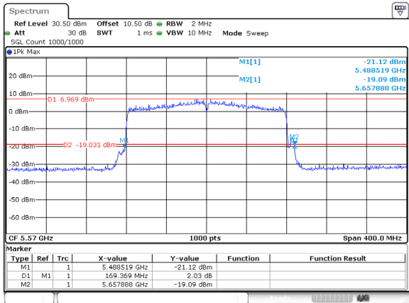
802.11be160_5570MHz_RU_FULL_Ant 1
