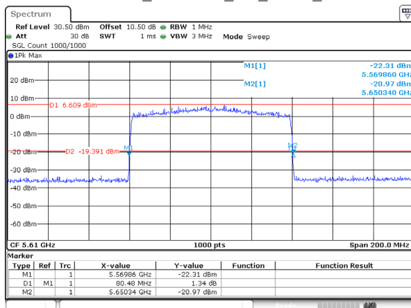
802.11be80_5610MHz_RU_FULL_Ant 2
