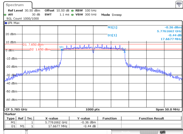
802.11ac20_5785MHz_Ant 2
