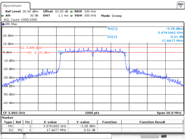
802.11ac20_5885MHz_Ant 2
