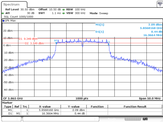
802.11a_5865MHz_Ant 0
