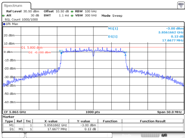
802.11ac20_5865MHz_Ant 2
