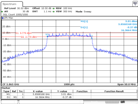
802.11a_5865MHz_Ant 1
