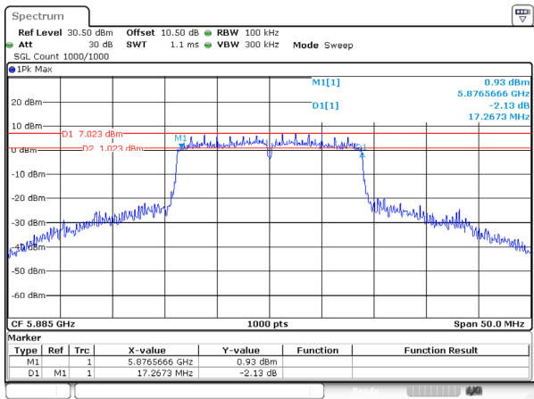
802.11ac20_5885MHz_Ant 1
