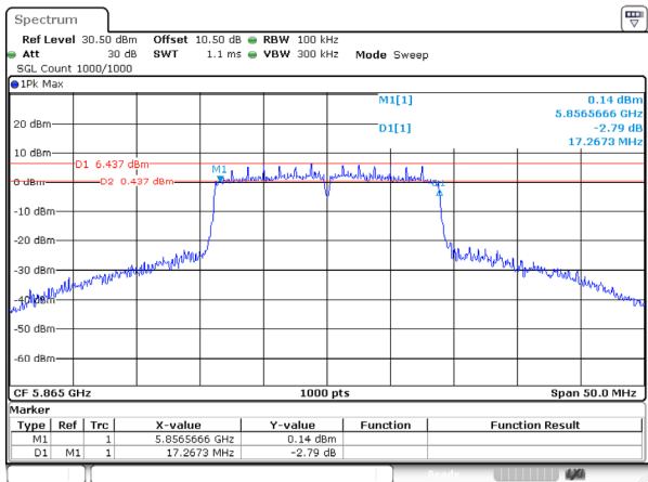
802.11ac20_5865MHz_Ant 0
