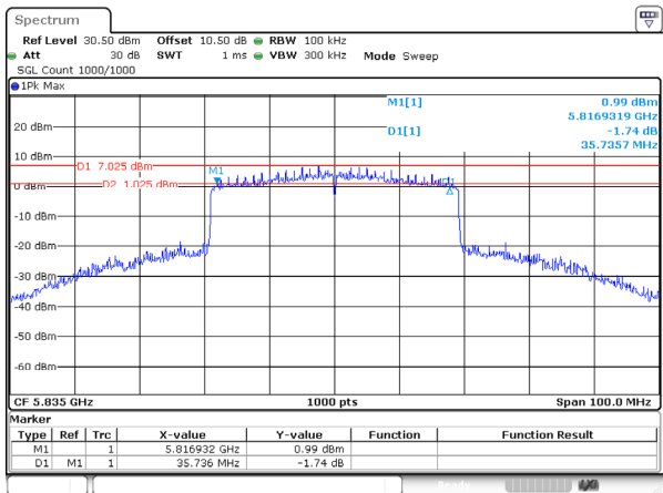
802.11be40_5835MHz_RU_Full_Ant 2
