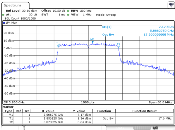
802.11ac20_5865MHz_Ant 2
