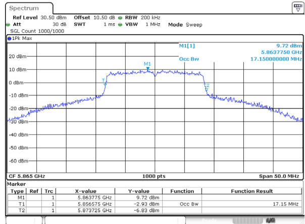
802.11a_5865MHz_Ant 2
