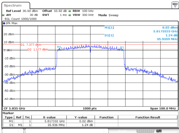
802.11be40_5835MHz_RU_Full_Ant 1
