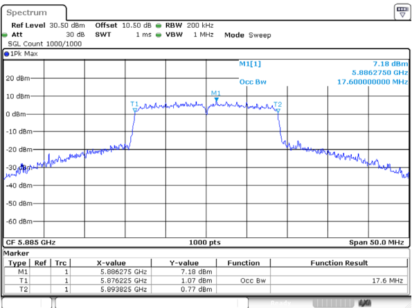
802.11ac20_5885MHz_Ant 2
