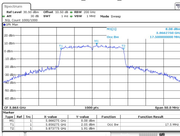
802.11ac20_5865MHz_Ant 0
