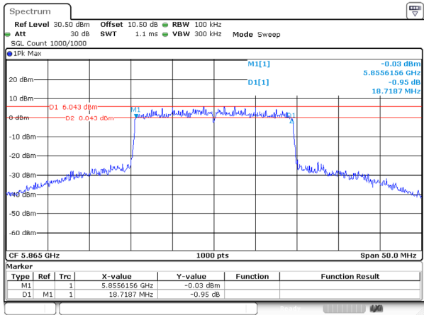
802.11be20_5865MHz_RU_Full_Ant 0
