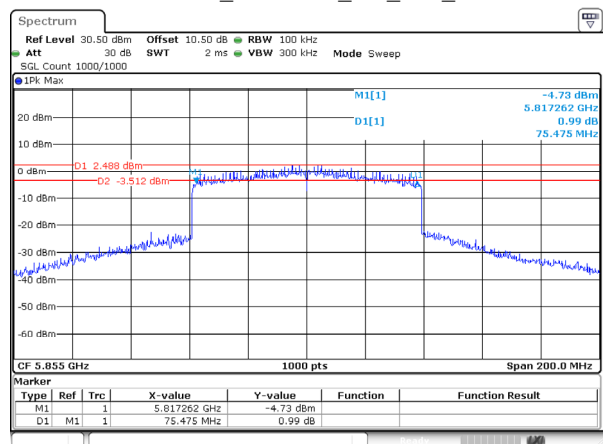
802.11ax80_5855MHz_RU_Full_Ant 2
