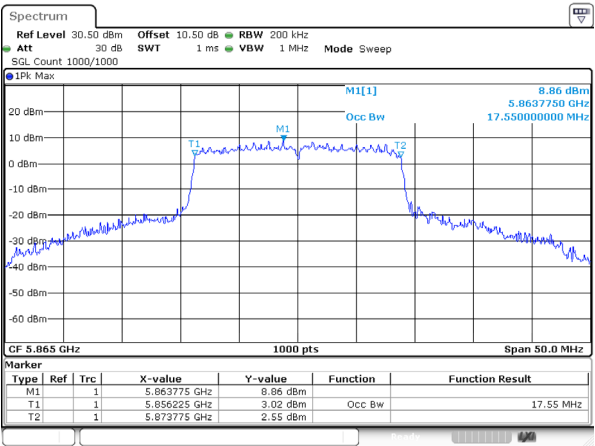
802.11ac20_5865MHz_Ant 1
