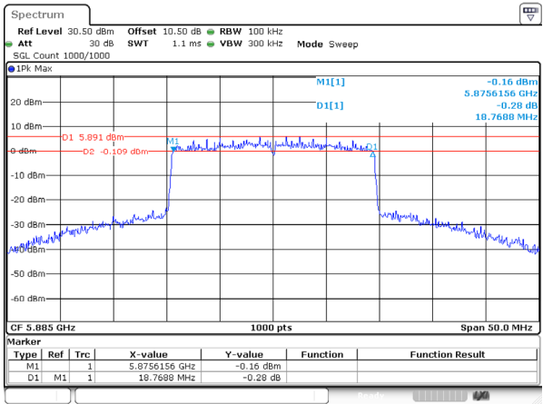
802.11be20_5885MHz_RU_Full_Ant 0
