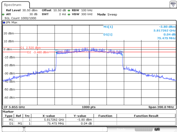
802.11ac80_5855MHz_Ant 2
