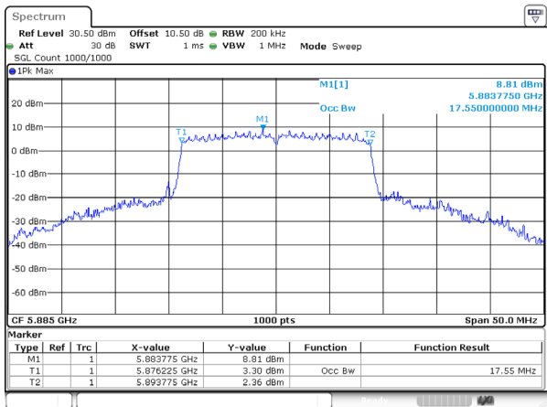
802.11ac20_5885MHz_Ant 1
