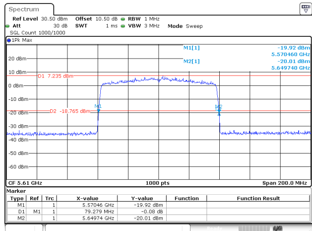
802.11ac80_5610MHz_Chain 2
