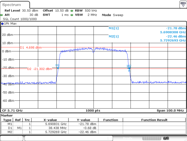
802.11ac40_5710MHz_Chain 2
