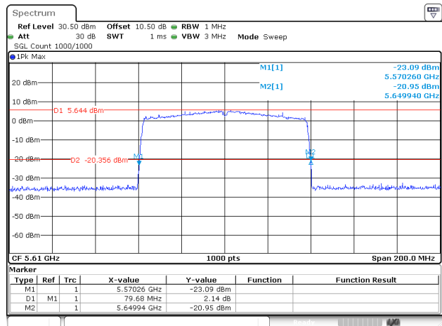
802.11ac80_5610MHz_Chain 0
