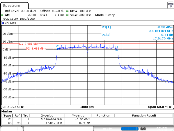
802.11ac20_5825MHz_Chain 0
