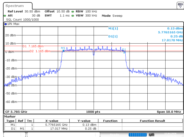
802.11ac20_5785MHz_Chain 0
