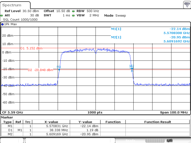
802.11ac40_5590MHz_Chain 2
