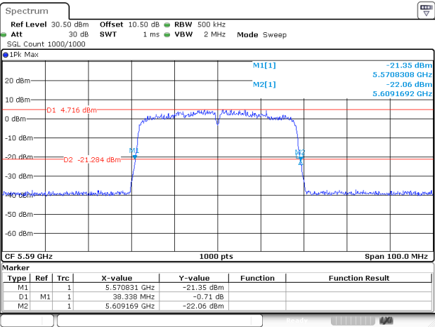
802.11ac40_5590MHz_Chain 1
