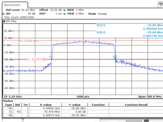
802.11ac80_5530MHz_Chain 2
