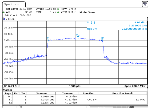
802.11ac80_5290MHz_Chain 0
