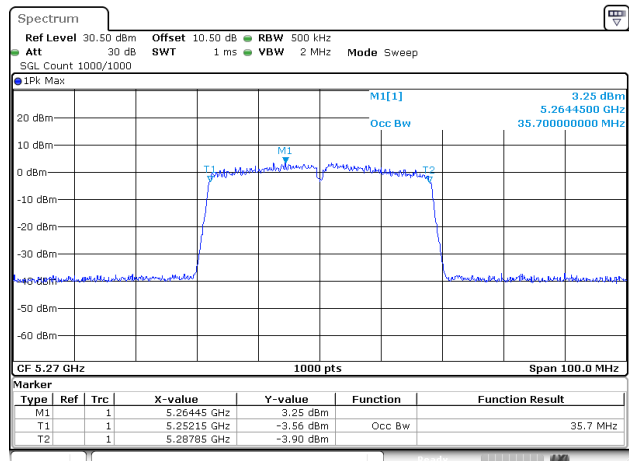
802.11ac40_5270MHz_Chain 2
