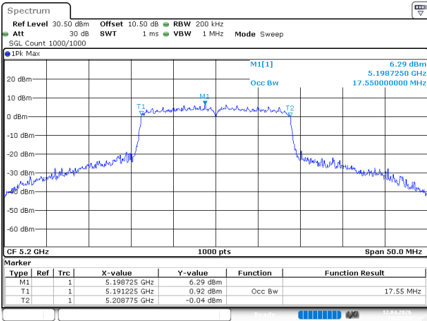
802.11ac20_5200MHz_Chain 2
