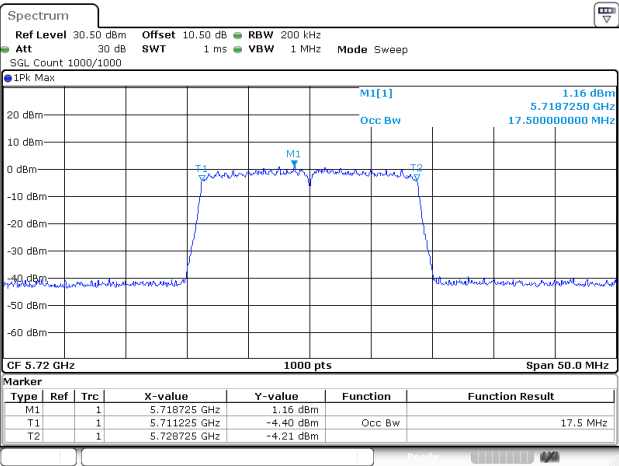
802.11ac20_5720MHz_Chain 2
