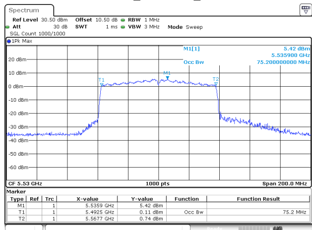
802.11ac80_5530MHz_Chain 1
