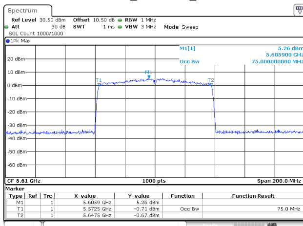
802.11ac80_5610MHz_Chain 1
