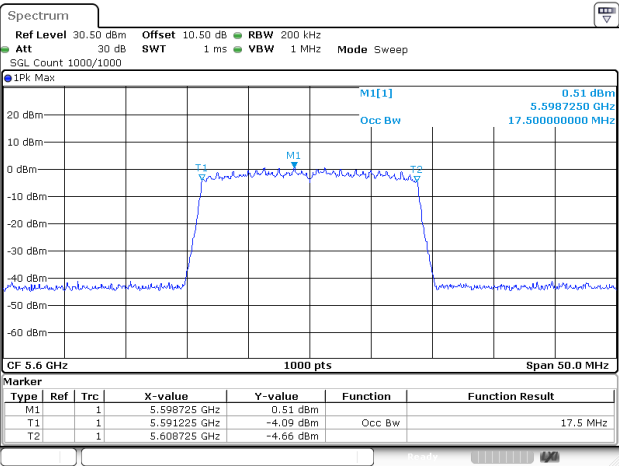
802.11ac20_5600MHz_Chain 1
