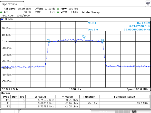
802.11ac40_5710MHz_Chain 0
