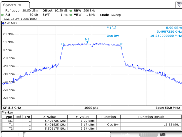
802.11a_5500MHz_Chain 2
