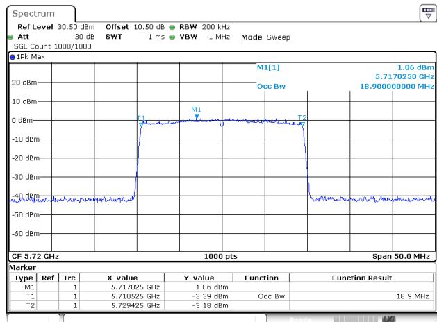
802.11be20_5720MHz_RU_Full_Chain 2
