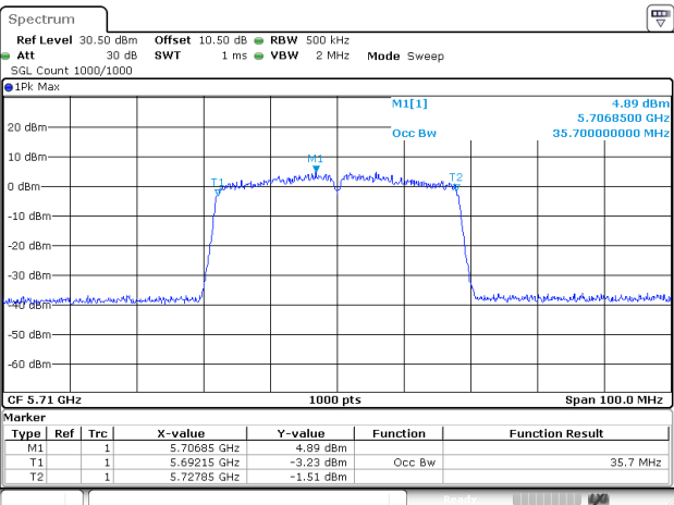
802.11ac40_5710MHz_Chain 2
