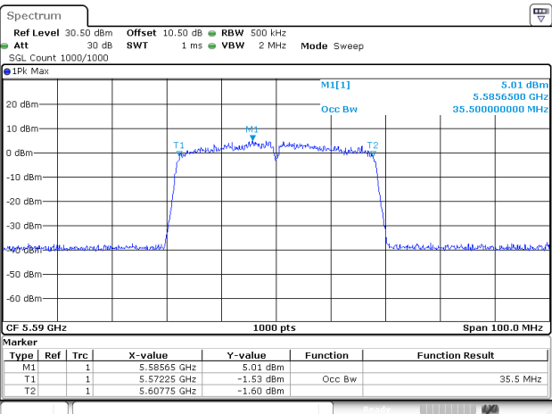
802.11ac40_5590MHz_Chain 1
