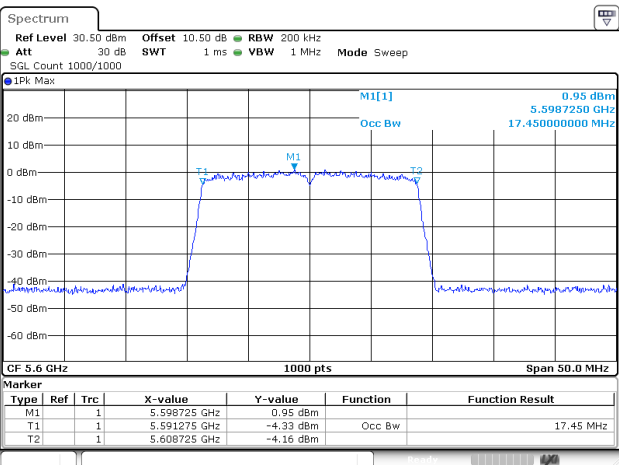
802.11ac20_5600MHz_Chain 0
