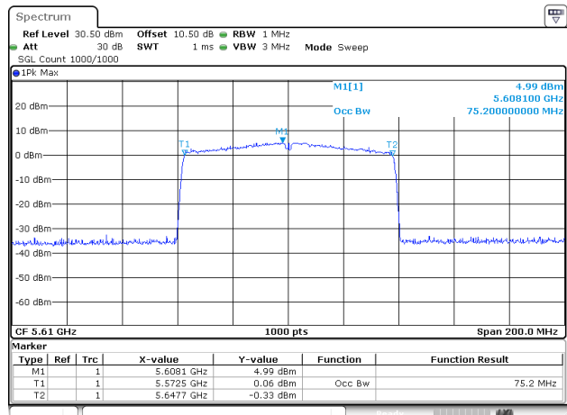
802.11ac80_5610MHz_Chain 0
