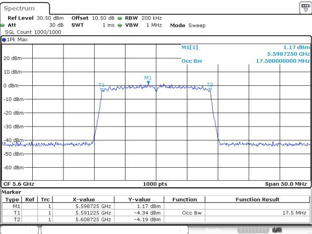
802.11ac20_5600MHz_Chain 2
