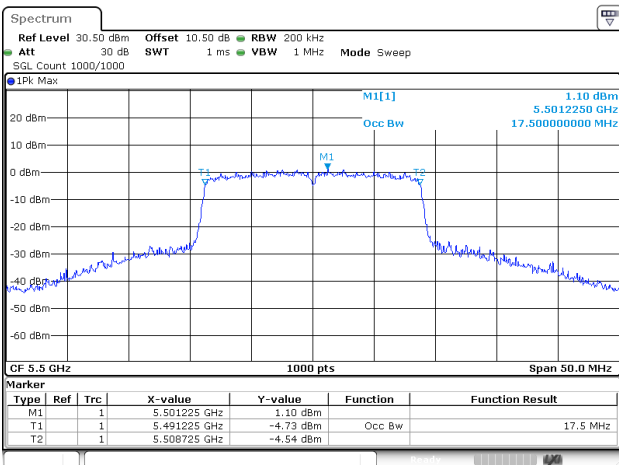
802.11ac20_5500MHz_Chain 0
