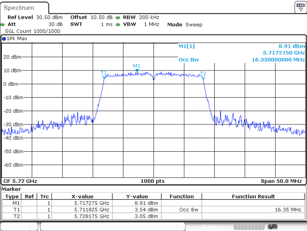
802.11a_5720MHz_Chain 2
