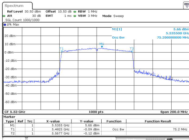
802.11ac80_5530MHz_Chain 0
