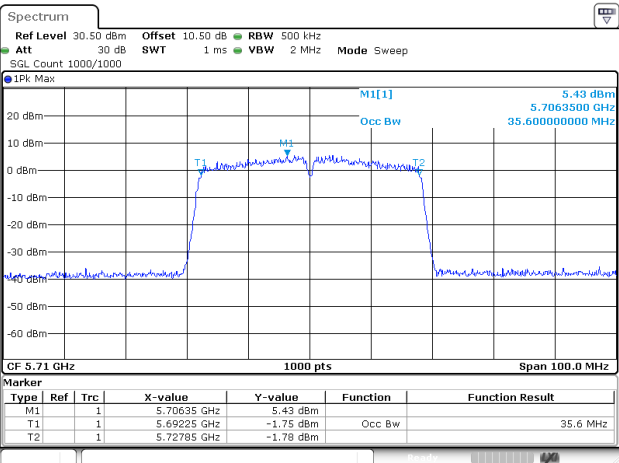
802.11ac40_5710MHz_Chain 1
