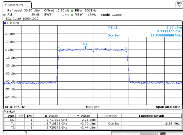
802.11be20_5720MHz_RU_Full_Chain 1
