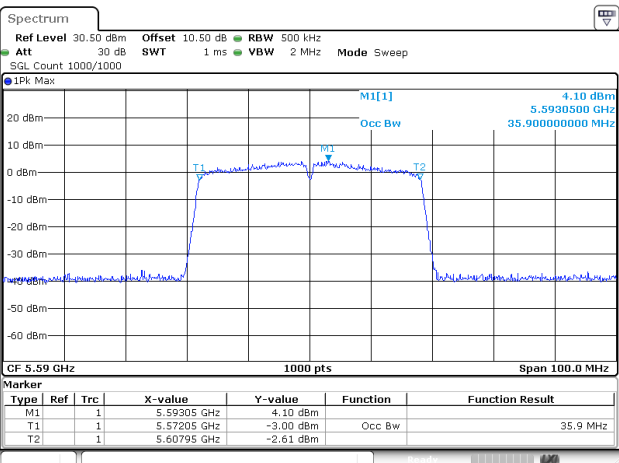
802.11ac40_5590MHz_Chain 0
