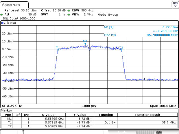
802.11ac40_5590MHz_Chain 2
