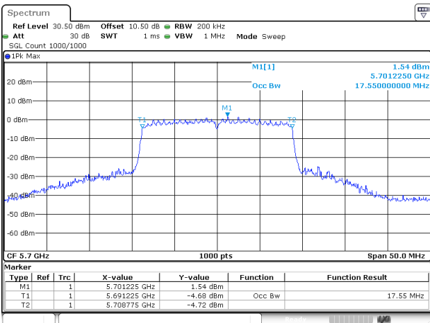
802.11ac20_5700MHz_Chain 1
