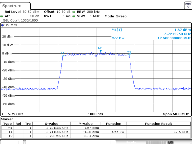
802.11ac20_5720MHz_Chain 1
