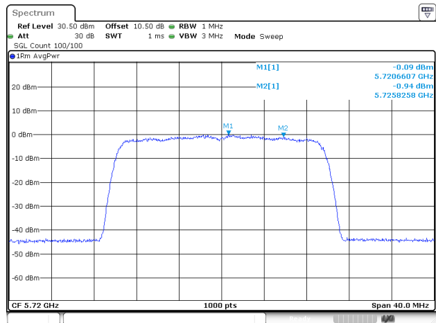
802.11be20_5720MHz_RU_Full_Chain 0
