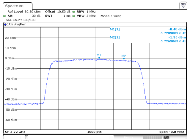
802.11be20_5720MHz_RU_Full_Chain 2
