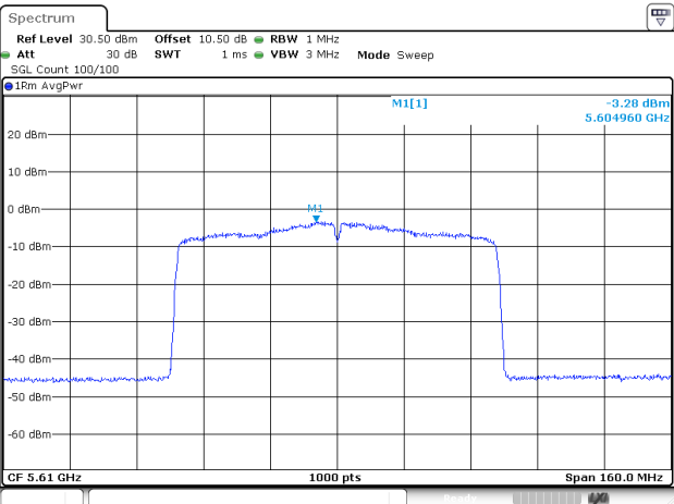
802.11ac80_5610MHz_Chain 2
