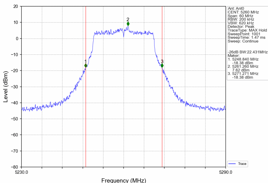
802.11n(HT20)_LCH_5260MHz_Ant0_NTNV
