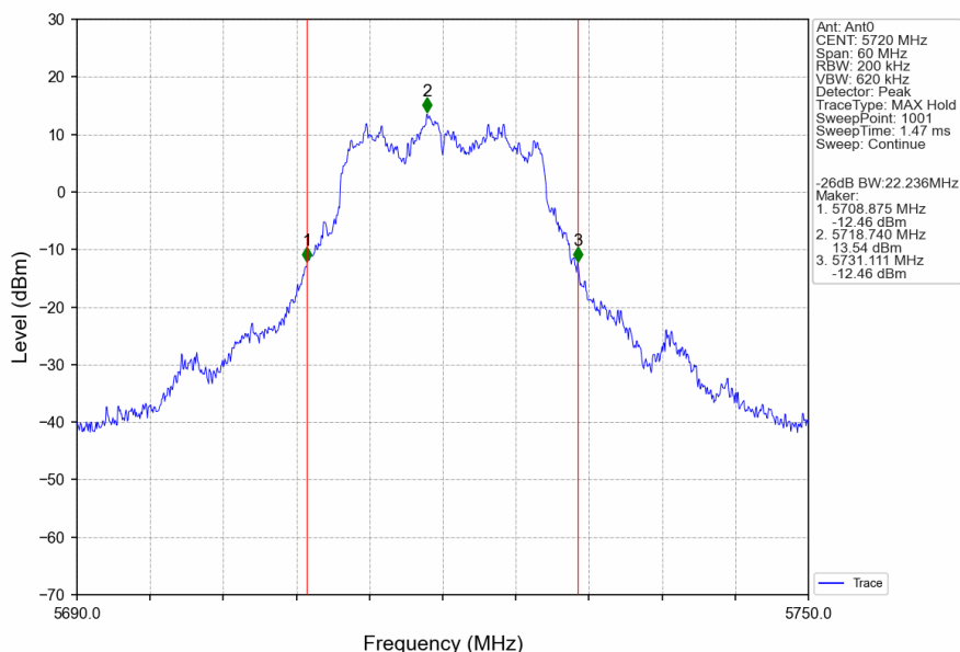
802.11a_HCH_5720MHz_Ant0_NTNV
