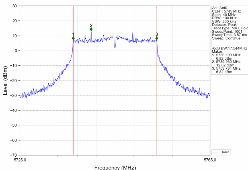
802.11n(HT20)_LCH_5745MHz_Ant0_NTNV
