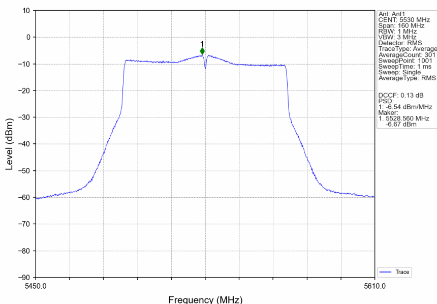
802.11ac(VHT80)_LCH_5530MHz_Ant1_NTNV
