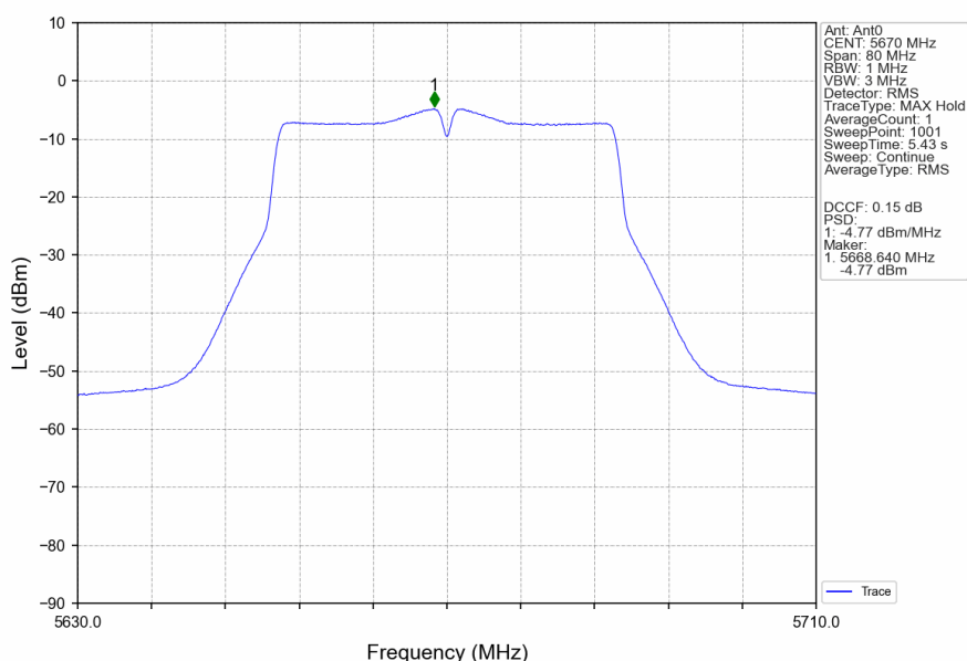
802.11n(HT40)_HCH_5670MHz_Ant0_NTNV
