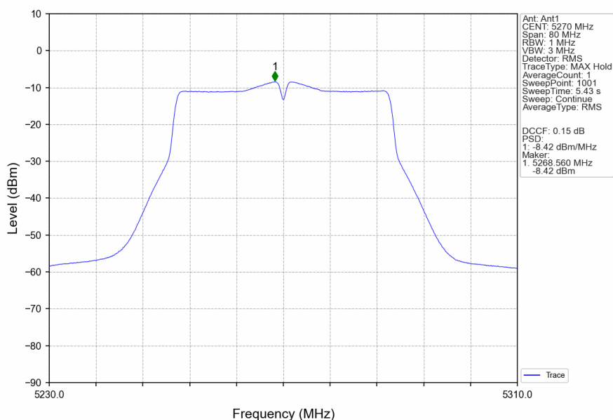
802.11n(HT40)_LCH_5270MHz_MIMO_NTNV
