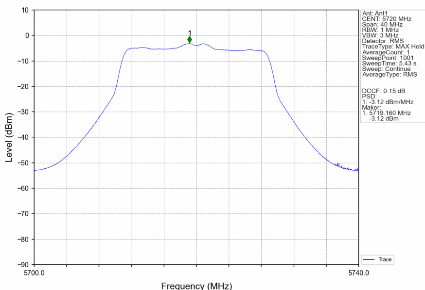
802.11ac(VHT20)_HCH_5720MHz_Ant1_NTNV
