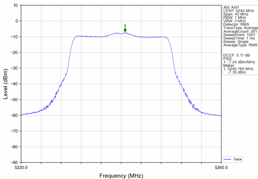
802.11be(EHT20)_HCH_5240MHz_SU_ / _Ant1_NTNV
