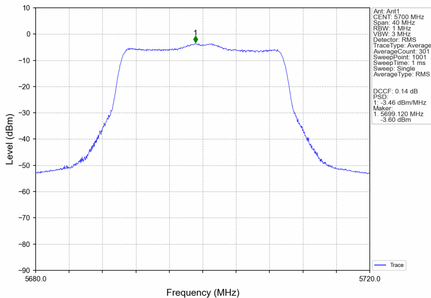
802.11be(EHT20)_HCH_5700MHz_SU_ / _Ant1_NTNV
