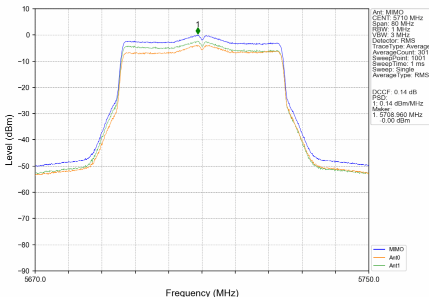
802.11be(EHT40)_HCH_5710MHz_SU_ / _MIMO_NTNV
