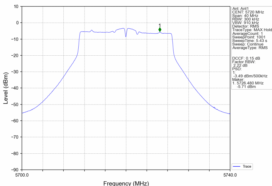
802.11ac(VHT20)_HCH_5720MHz_Ant1_NTNV
