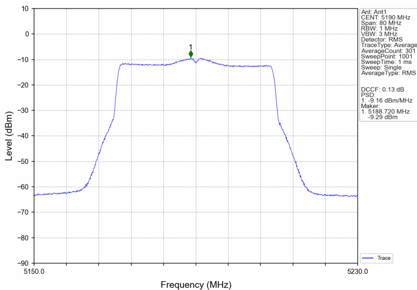
802.11be(EHT40)_LCH_5190MHz_SU_ / _Ant1_NTNV
