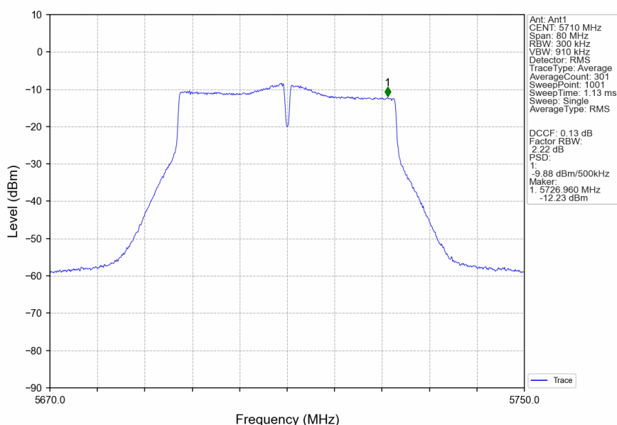
802.11n(HT40)_HCH_5710MHz_Ant1_NTNV
