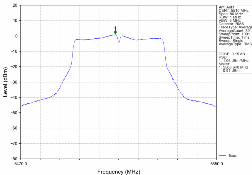
802.11n(HT40)_LCH_5510MHz_Ant1_NTNV
