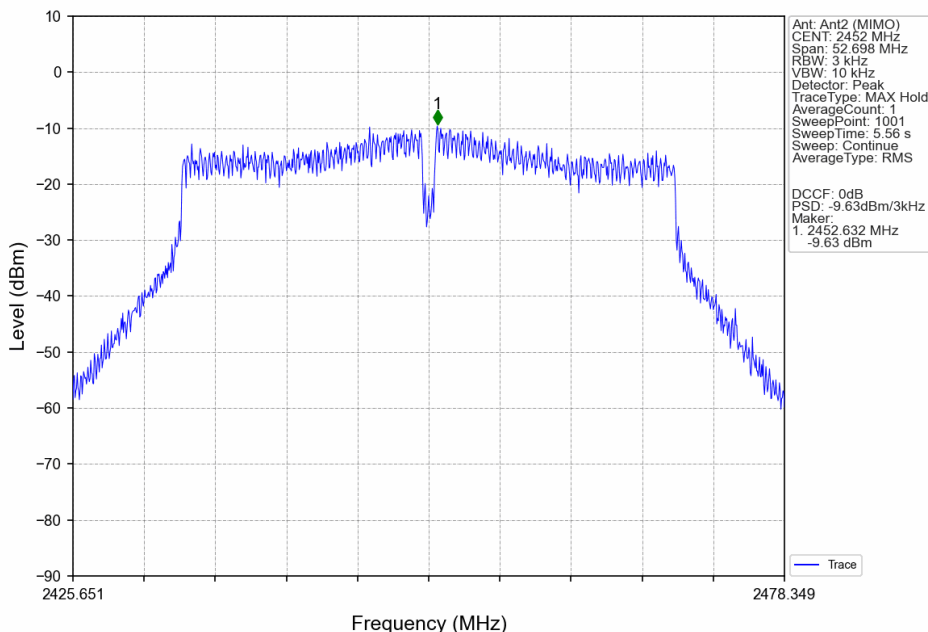
802.11n(HT40)_HCH_2452MHz_MIMO_NTNV
