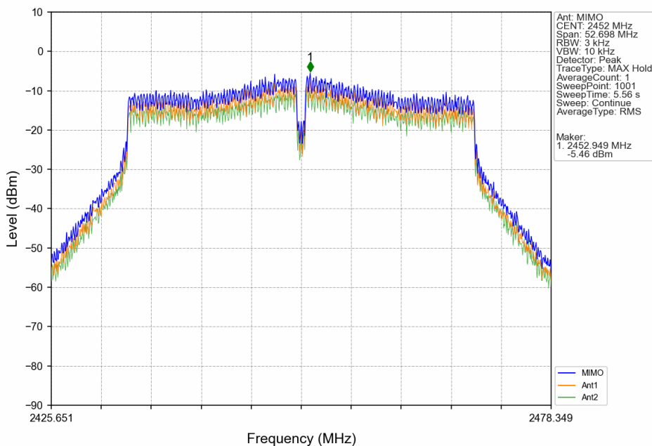
802.11n(HT40)_HCH_2452MHz_MIMO_NTNV
