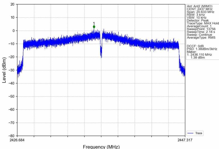
802.11be(EHT20)_MCH_2437MHz_SU_/_MIMO_NTNV
