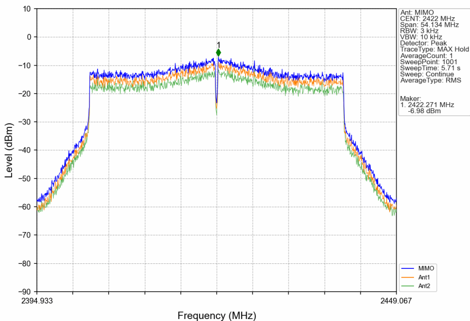
802.11be(EHT40)_LCH_2422MHz_SU_/_MIMO_NTNV
