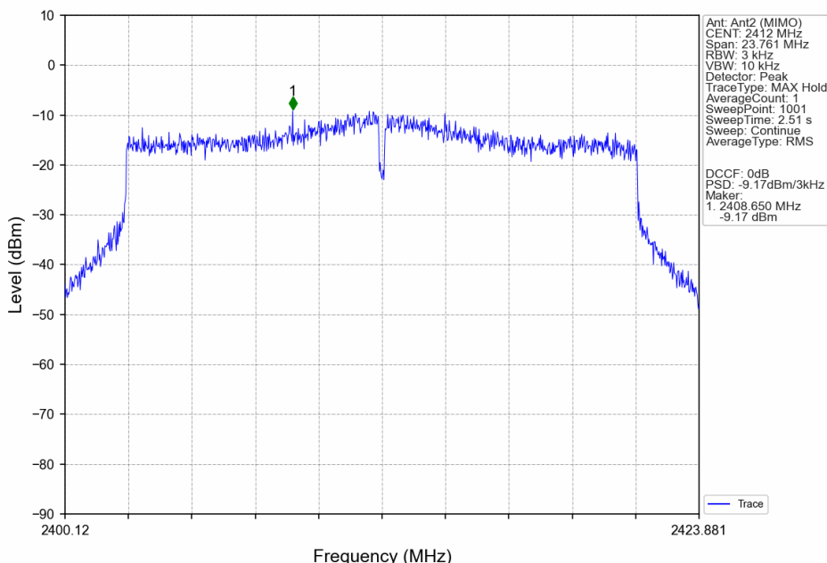
802.11be(EHT20)_LCH_2412MHz_SU_/_Ant2 (MIMO)_NTNV
