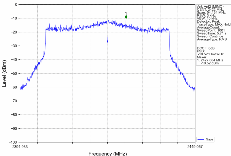
802.11be(EHT40)_LCH_2422MHz_SU_/_MIMO_NTNV
