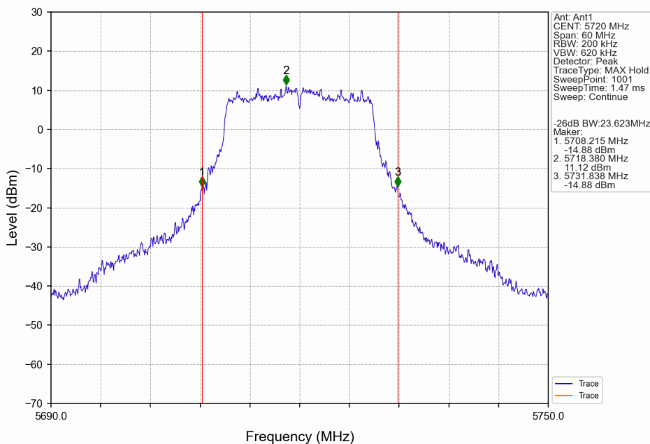
802.11ac(VHT20)_HCH_5720MHz_Ant1_NTNV
