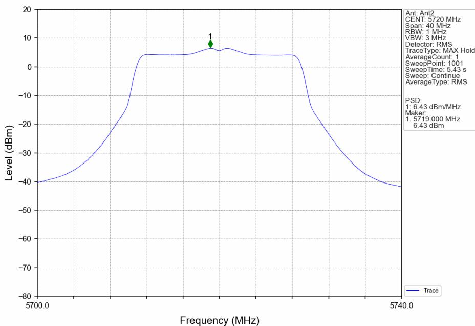
802.11n(HT20)_HCH_5720MHz_MIMO_NTNV
