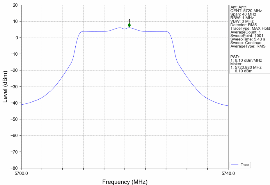
802.11n(HT20)_HCH_5720MHz_Ant1_NTNV
