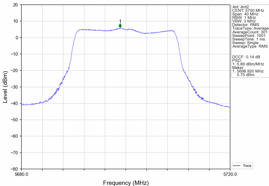
802.11be(EHT20)_HCH_5700MHz_SU_ / _MIMO_NTNV
