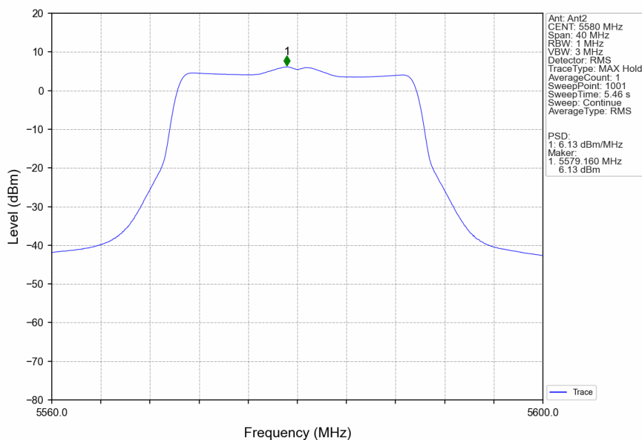
802.11be(EHT20)_MCH_5580MHz_SU_/_Ant2_NTNV
