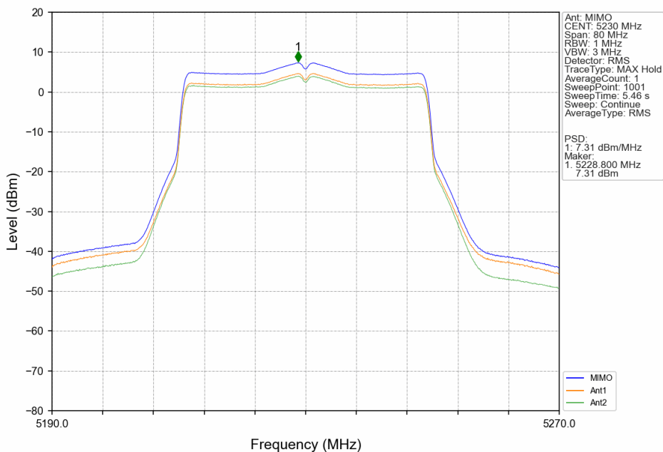
802.11be(EHT40)_HCH_5230MHz_SU_ / _MIMO_NTNV
