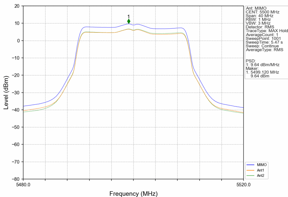
802.11be(EHT20)_LCH_5500MHz_SU_/_MIMO_NTNV
