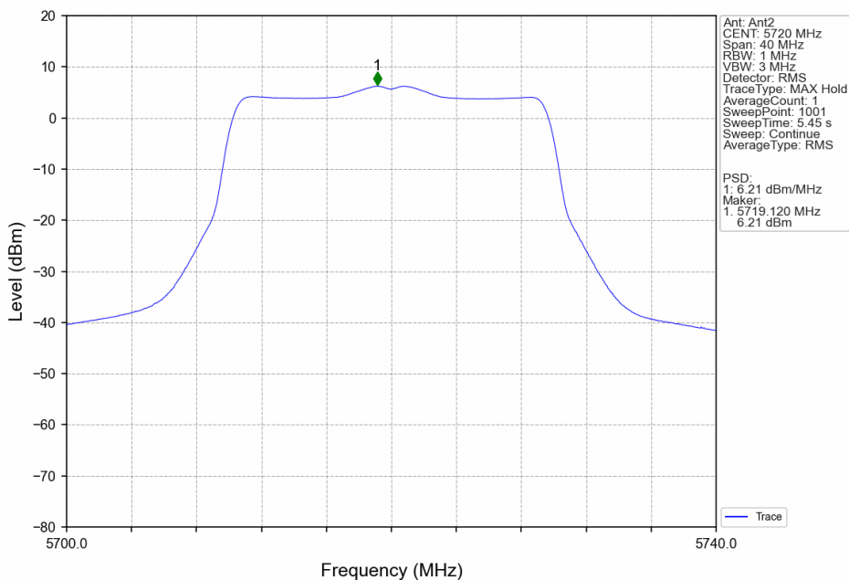
802.11be(EHT20)_HCH_5720MHz_SU_ / _Ant2_NTNV
