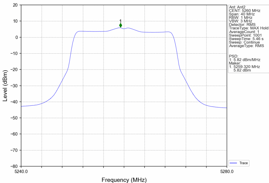
802.11be(EHT20)_LCH_5260MHz_SU_/_Ant2_NTNV
