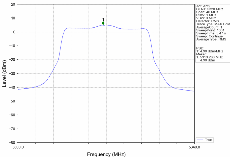
802.11be(EHT20)_HCH_5320MHz_SU_ / _Ant2_NTNV
