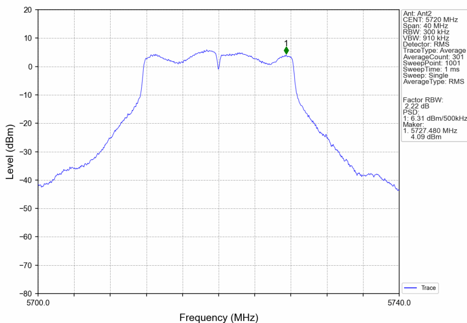
802.11a_HCH_5720MHz_Ant2_NTNV
