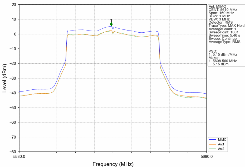
802.11be(EHT80)_HCH_5610MHz_SU_ / _MIMO_NTNV
