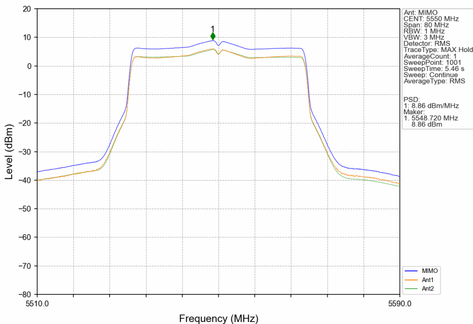
802.11be(EHT40)_MCH_5550MHz_SU_/_MIMO_NTNV
