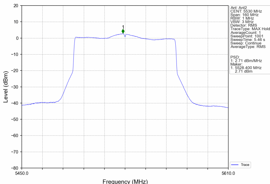
802.11be(EHT80)_LCH_5530MHz_SU_/_Ant2_NTNV
