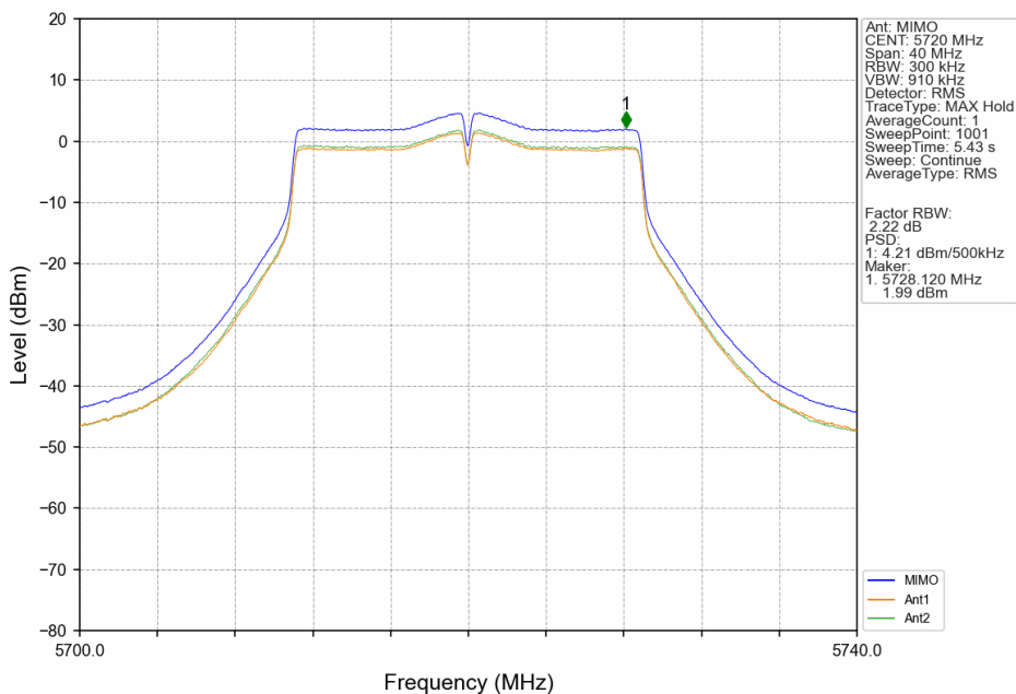
802.11n(HT20)_HCH_5720MHz_MIMO_NTNV
