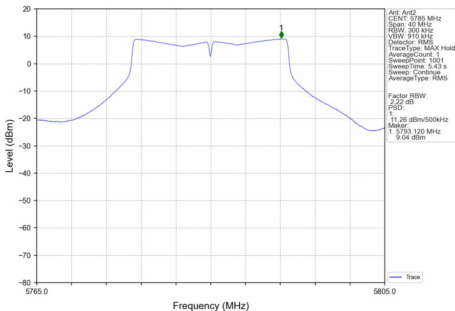
802.11n(HT20)_MCH_5785MHz_MIMO_NTNV
