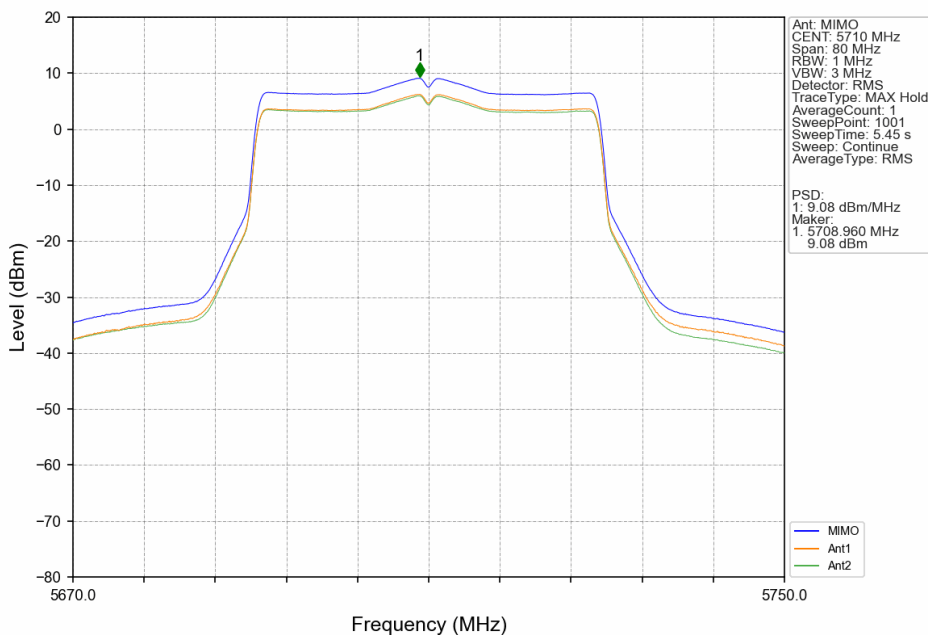
802.11be(EHT40)_HCH_5710MHz_SU_ / _MIMO_NTNV
