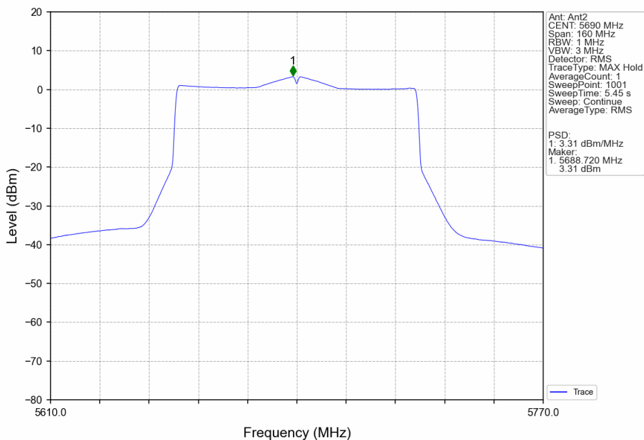
802.11be(EHT80)_HCH_5690MHz_SU_ / _Ant2_NTNV
