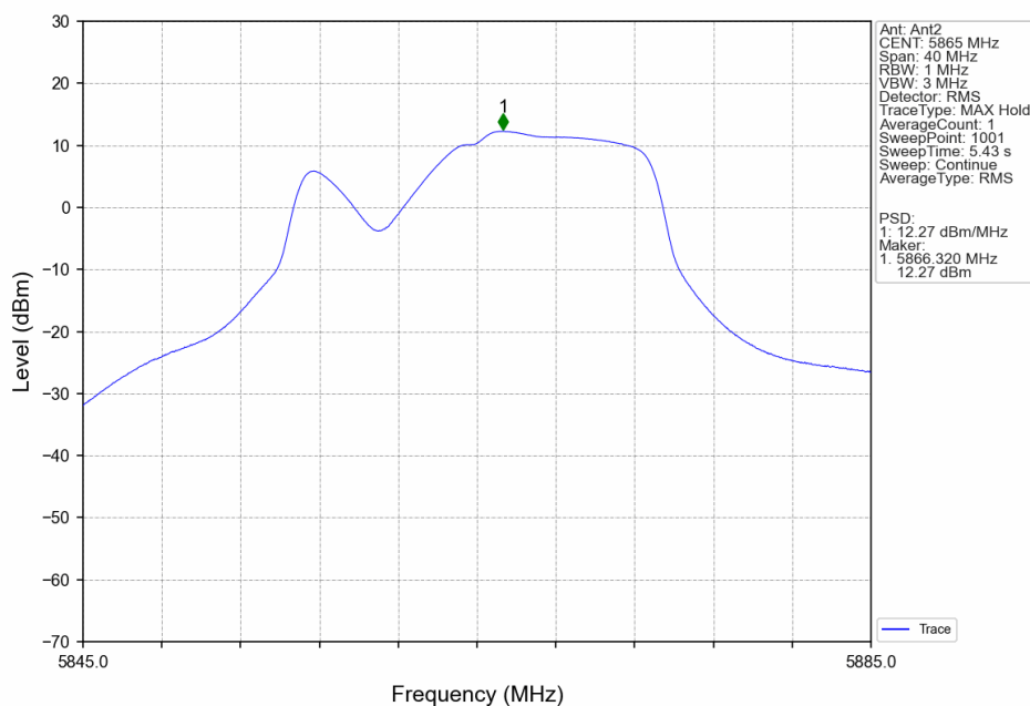
802.11n(HT20)_LCH_5865MHz_Ant2_NTNV
