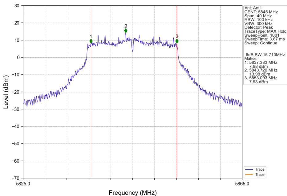
802.11a_HCH_5845MHz_Ant1_NTNV
