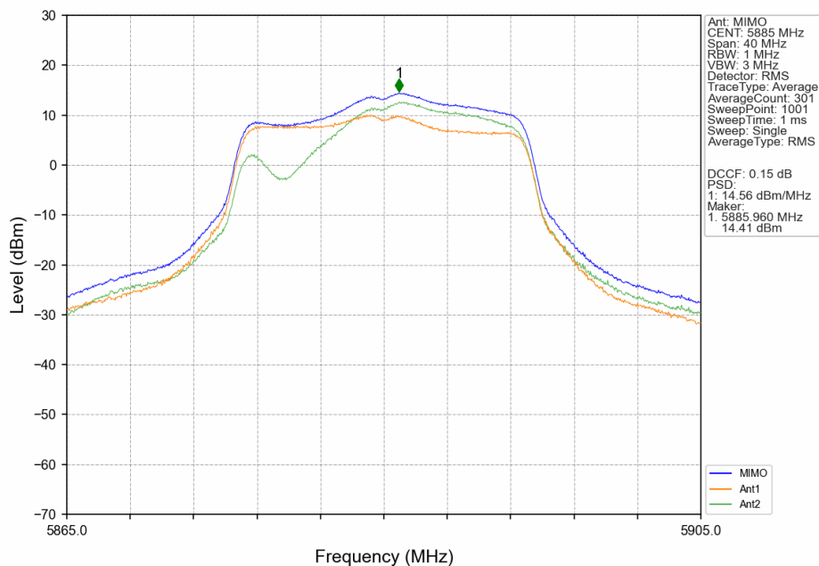
802.11n(HT20)_HCH_5885MHz_MIMO_NTNV
