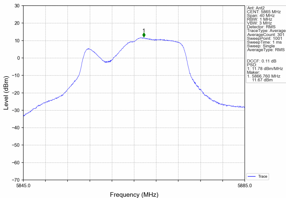
802.11ac(VHT20)_LCH_5865MHz_MIMO_NTNV
