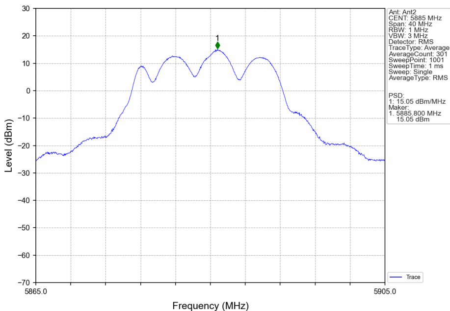
802.11a_HCH_5885MHz_Ant2_NTNV
