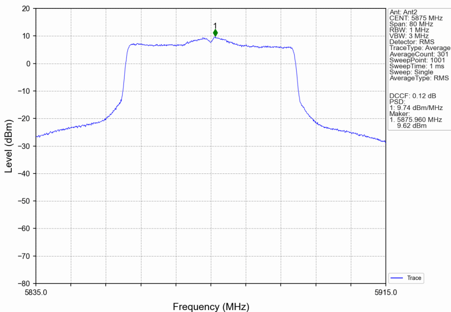
802.11be(EHT40)_MCH_5875MHz_SU_ / _Ant2_NTNV
