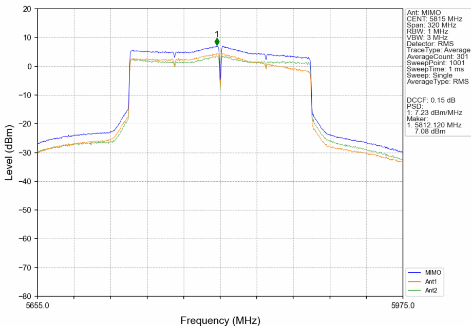
802.11be(EHT160)_HCH_5815MHz_SU_ / _MIMO_NTNV
