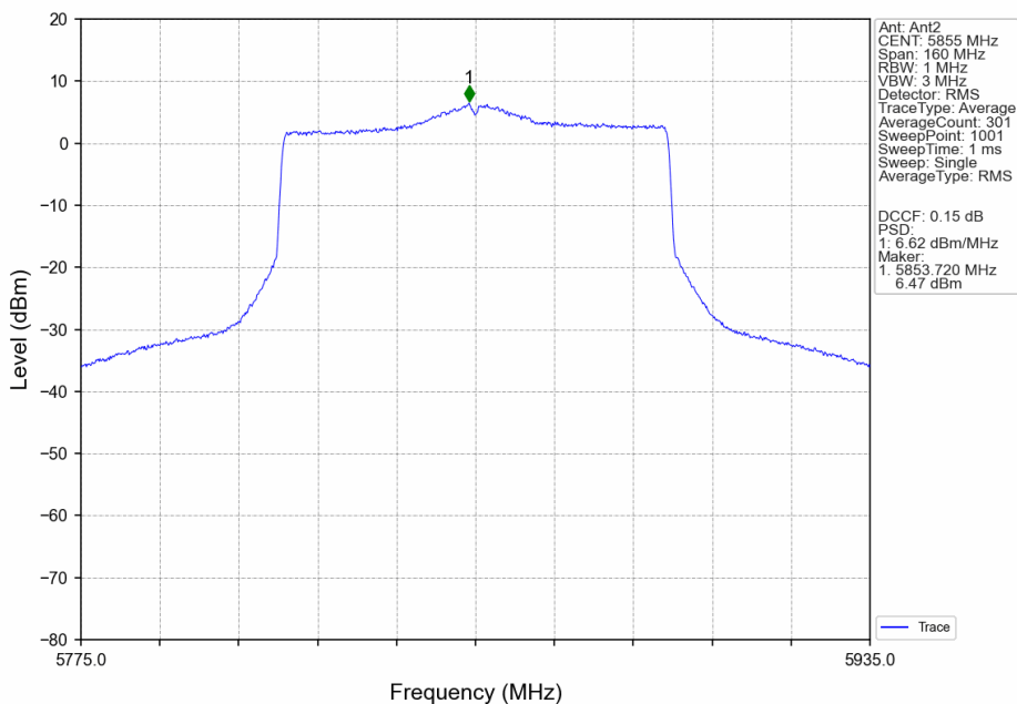
802.11be(EHT80)_HCH_5855MHz_SU_ / _Ant2_NTNV
