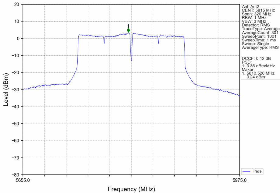
802.11ac(VHT160)_HCH_5815MHz_MIMO_NTNV
