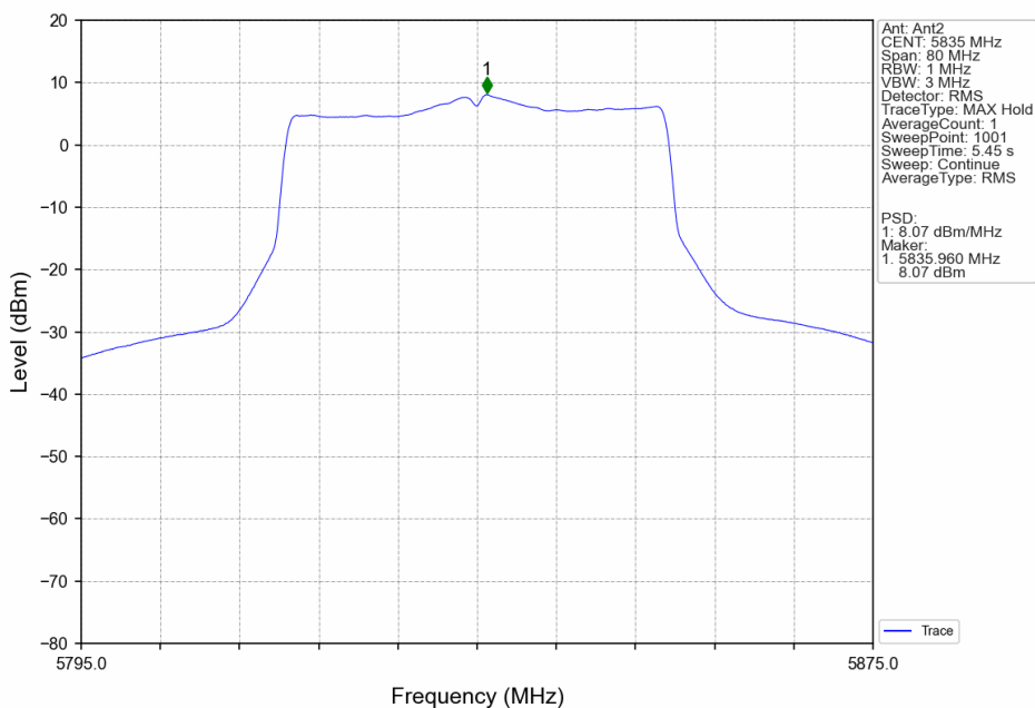
802.11be(EHT40)_HCH_5835MHz_SU_ / _MIMO_NTNV
