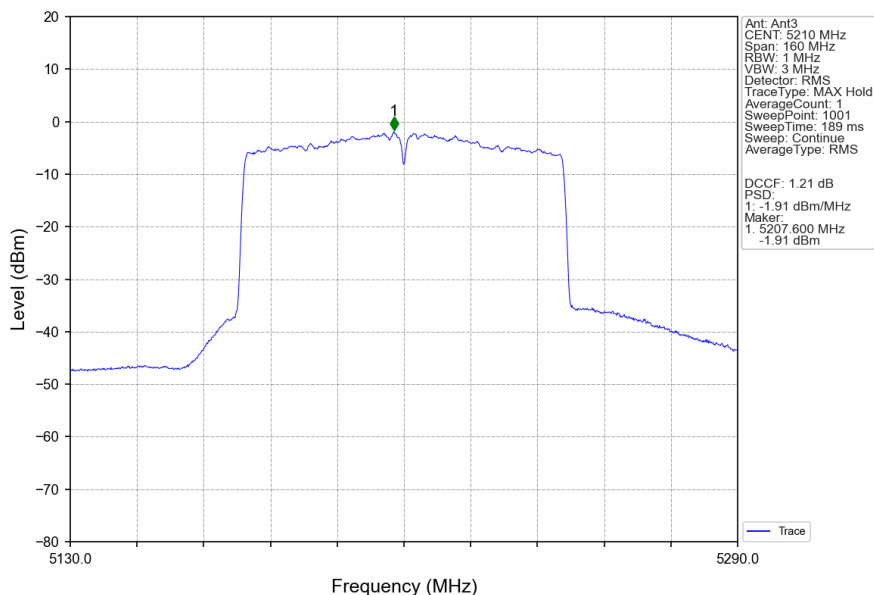
802.11ac(VHT80)_MCH_5210MHz_MIMO_NTNV
