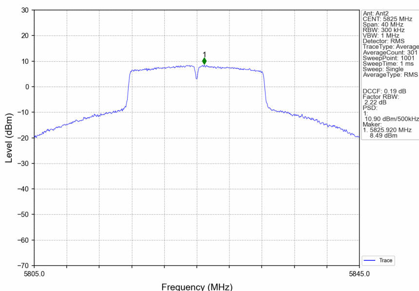
802.11a_HCH_5825MHz_Ant2_NTNV
