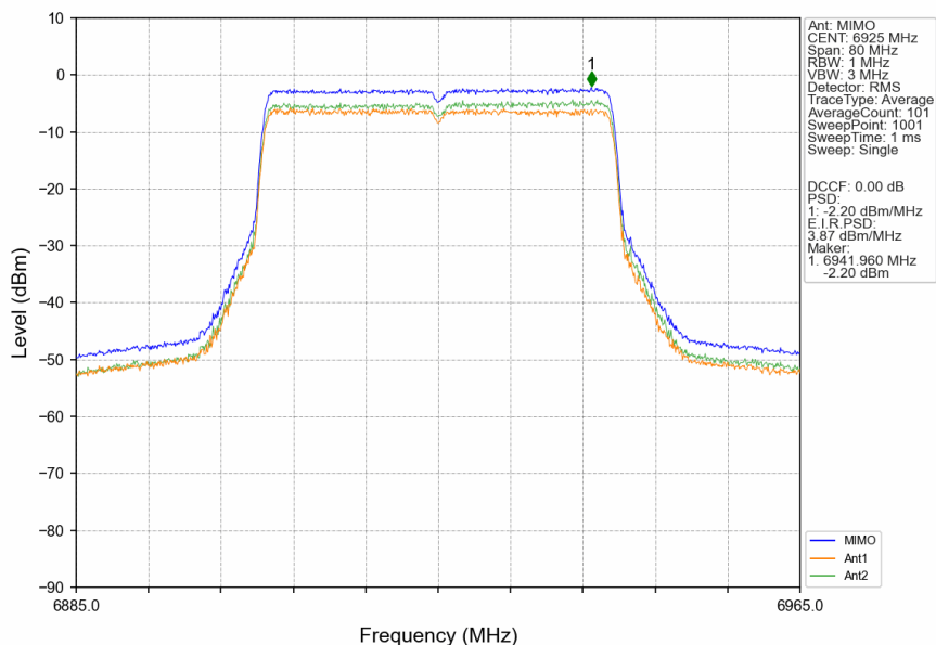
802.11be(EHT40)_LCH_6925MHz_RU484_Left_MIMO_NTNV
