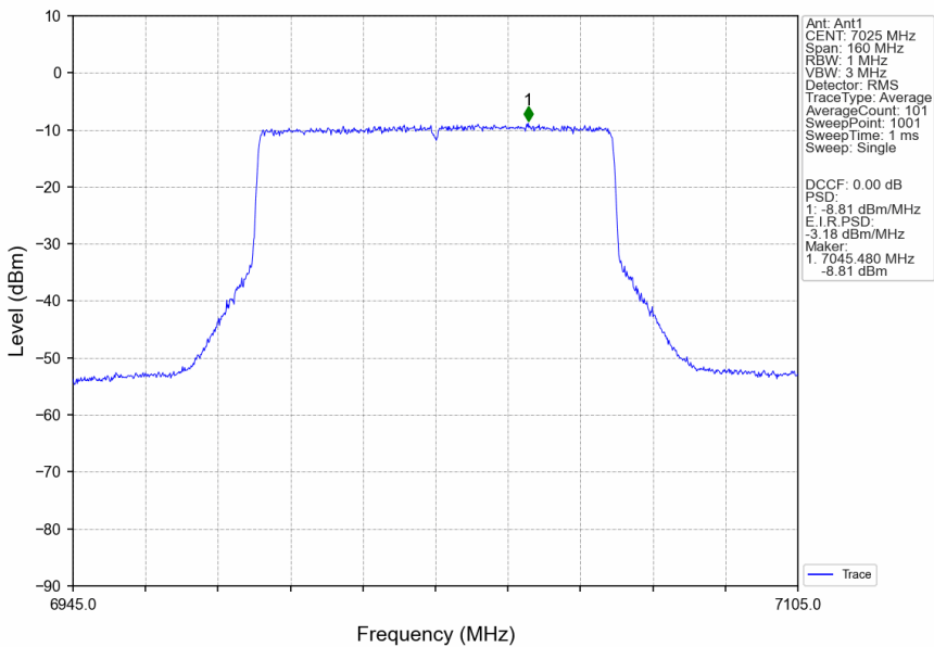
802.11be(EHT80)_HCH_7025MHz_RU996_Left_Ant1_NTNV
