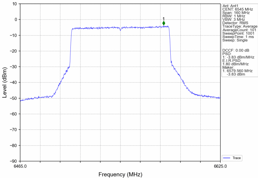
802.11be(EHT80)_HCH_6545MHz_RU996_Left_Ant1_NTNV
