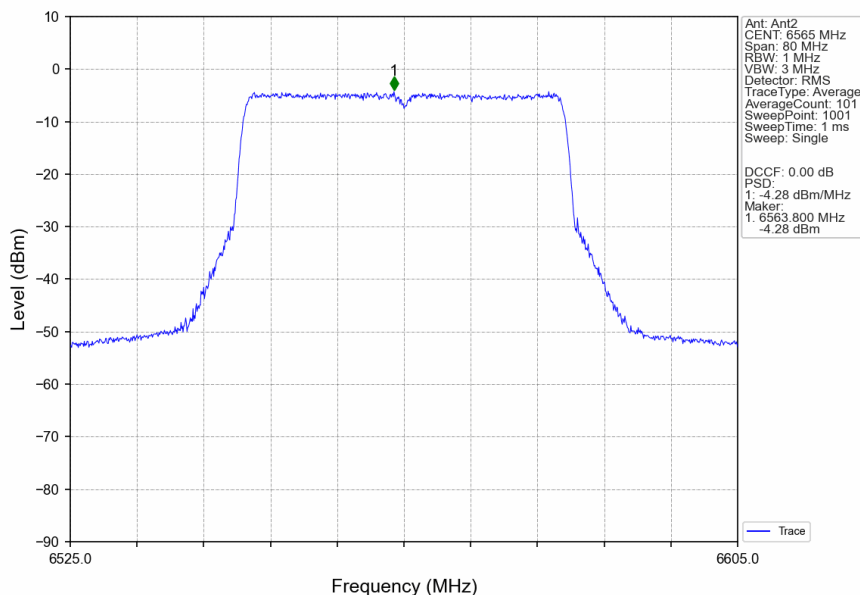
802.11ax(HEW40)_LCH_6565MHz_RU484_Left_Ant2_NTNV
