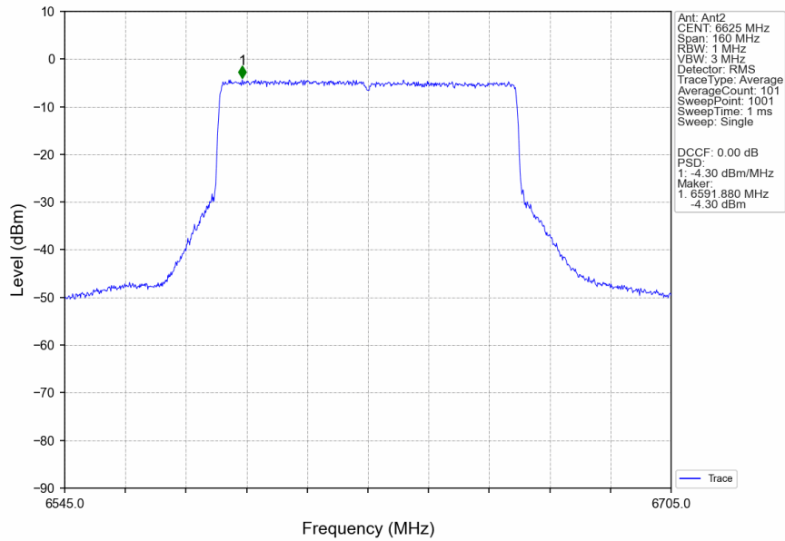
802.11ax(HEW80)_LCH_6625MHz_RU996_Left_Ant2_NTNV
