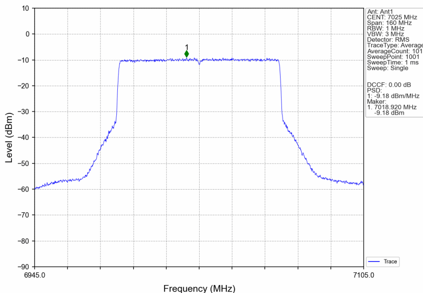
802.11ax(HEW80)_HCH_7025MHz_RU996_Left_Ant1_NTNV
