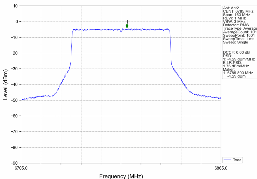
802.11ax(HEW80)_HCH_6785MHz_RU996_Left_Ant2_NTNV
