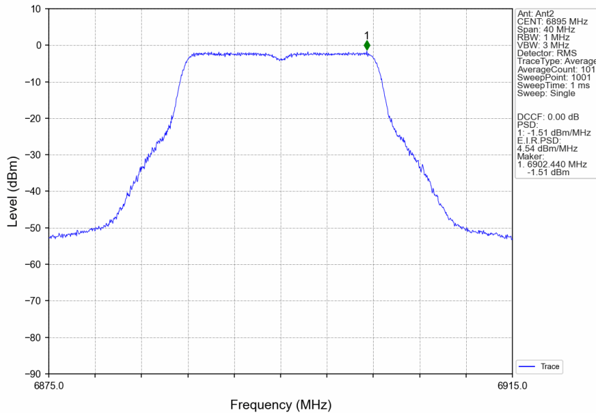
802.11a_LCH_6895MHz_Ant2_NTNV
