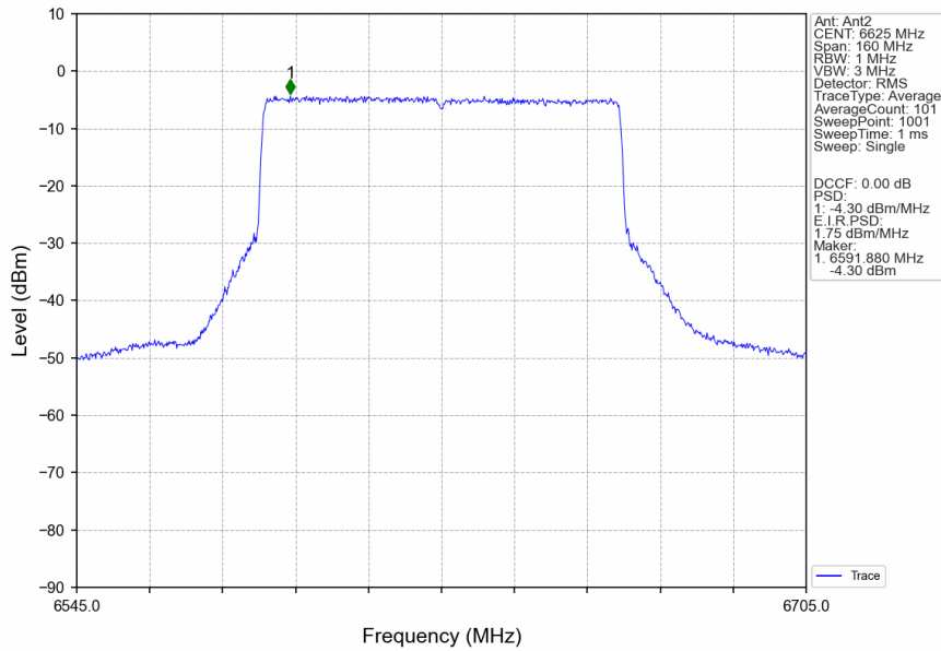
802.11ax(HEW80)_LCH_6625MHz_RU996_Left_Ant2_NTNV
