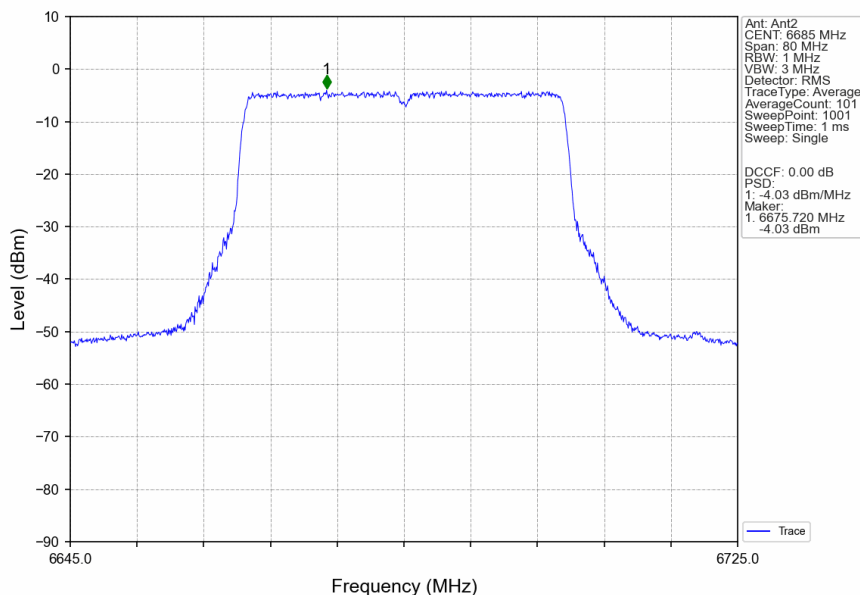
802.11ax(HEW40)_MCH_6685MHz_RU484_Left_Ant2_NTNV
