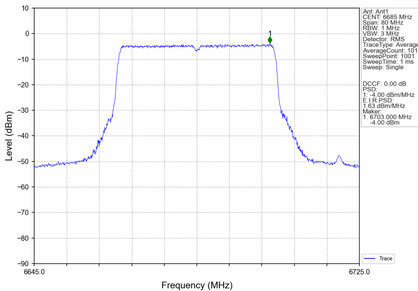
802.11ax(HEW40)_MCH_6685MHz_RU484_Left_Ant1_NTNV
