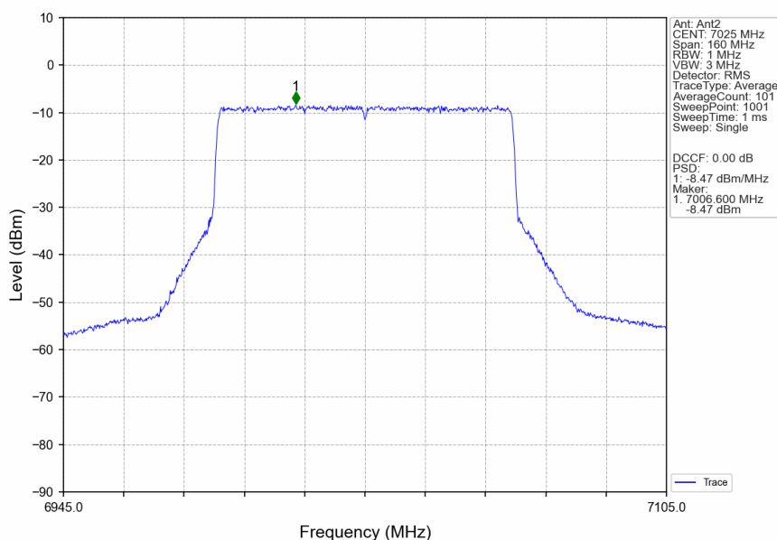
802.11ax(HEW80)_HCH_7025MHz_RU996_Left_Ant2_NTNV
