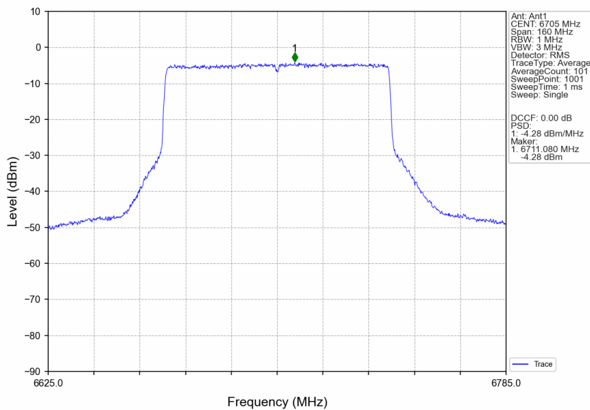
802.11ax(HEW80)_MCH_6705MHz_RU996_Left_Ant1_NTNV
