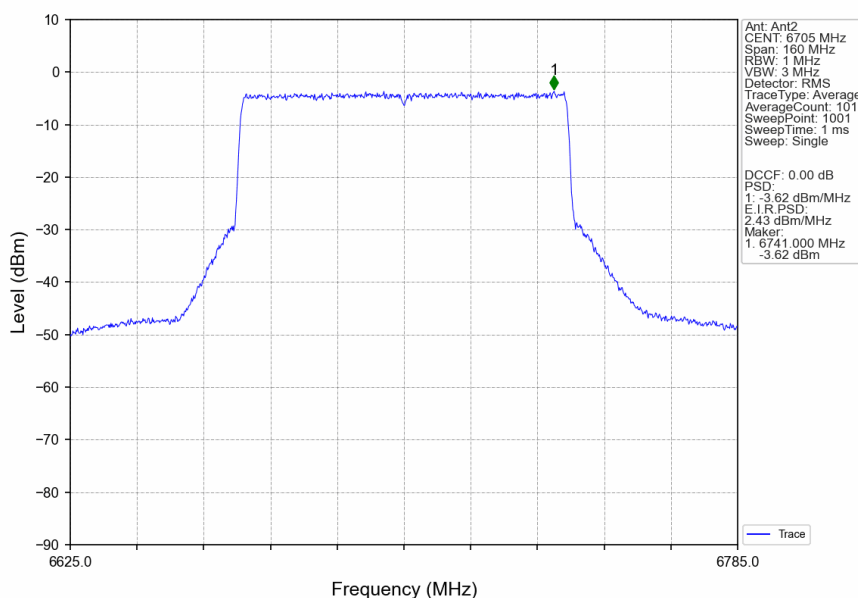
802.11ax(HEW80)_MCH_6705MHz_RU996_Left_Ant2_NTNV
