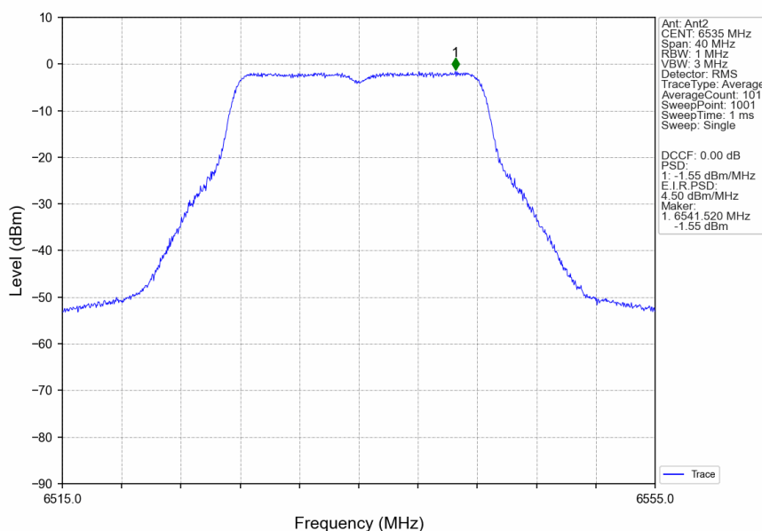
802.11a_LCH_6535MHz_Ant2_NTNV
