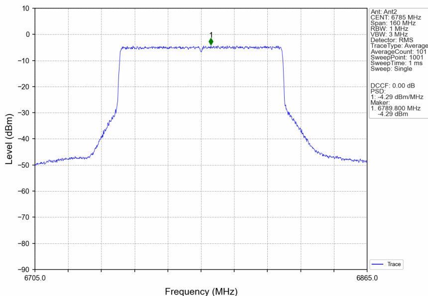
802.11ax(HEW80)_HCH_6785MHz_RU996_Left_Ant2_NTNV
