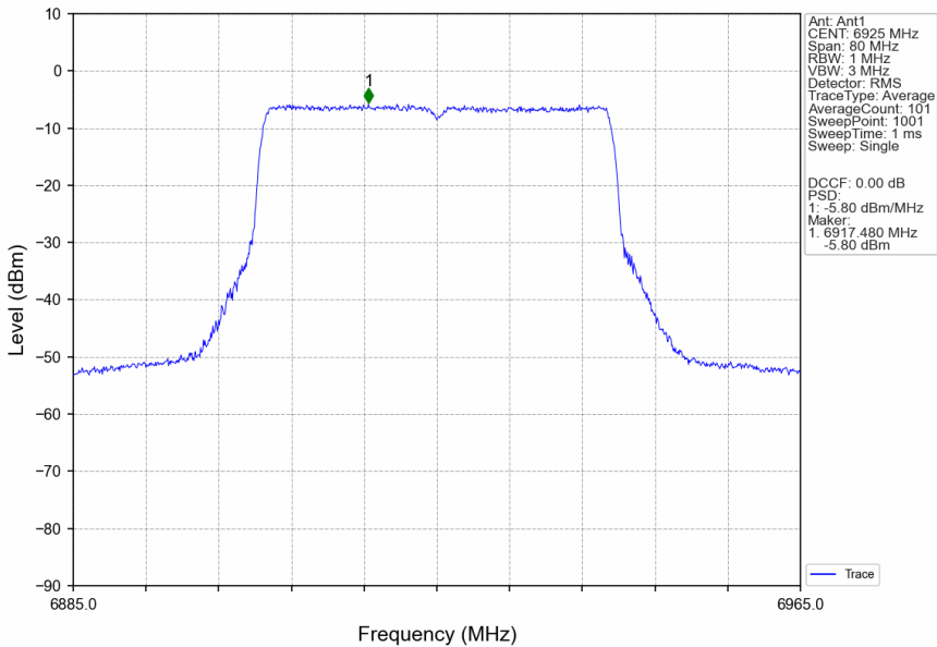
802.11ax(HEW40)_LCH_6925MHz_RU484_Left_Ant1_NTNV
