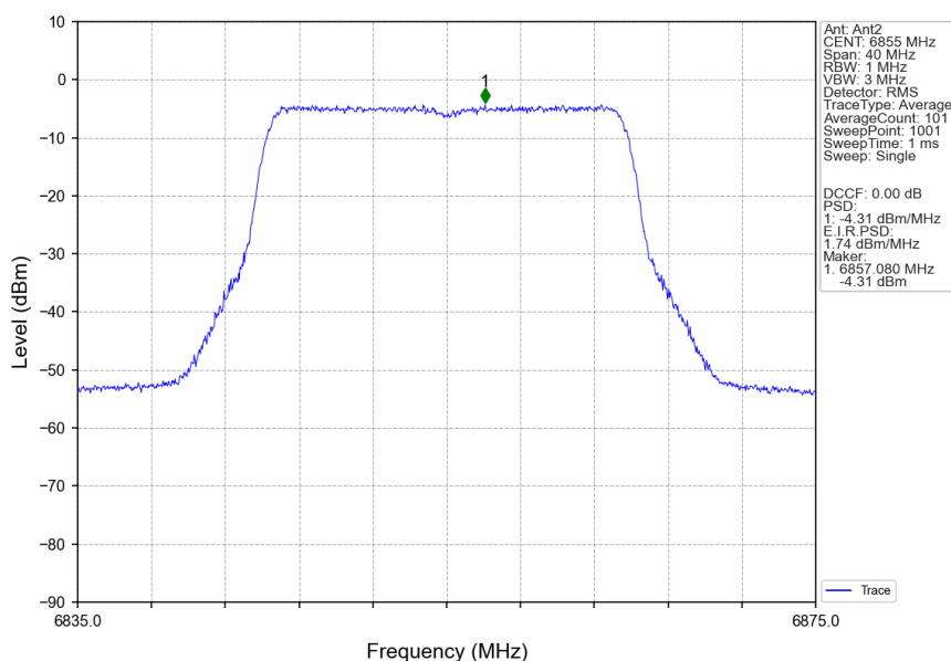
802.11ax(HEW20)_HCH_6855MHz_RU242_Left_Ant2_NTNV
