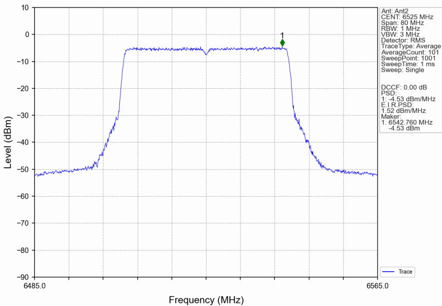
802.11ax(HEW40)_HCH_6525MHz_RU484_Left_Ant2_NTNV
