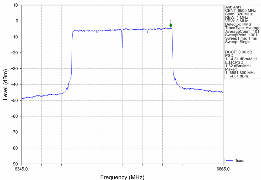
802.11ax(HEW160)_HCH_6505MHz_2xRU996_Left_Ant1_NTNV
