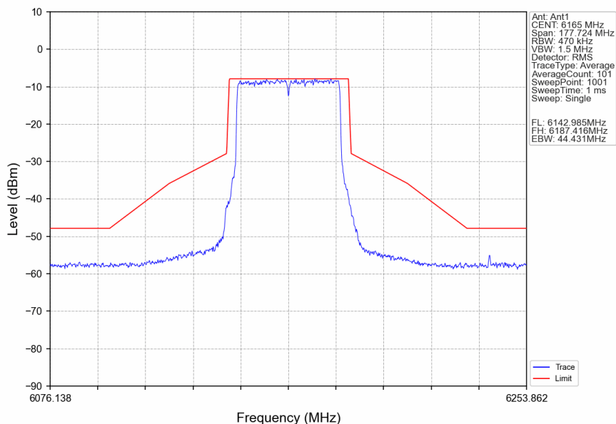
802.11ax(HEW40)_MCH_6165MHz_RU484_Left_Ant1_NTNV
