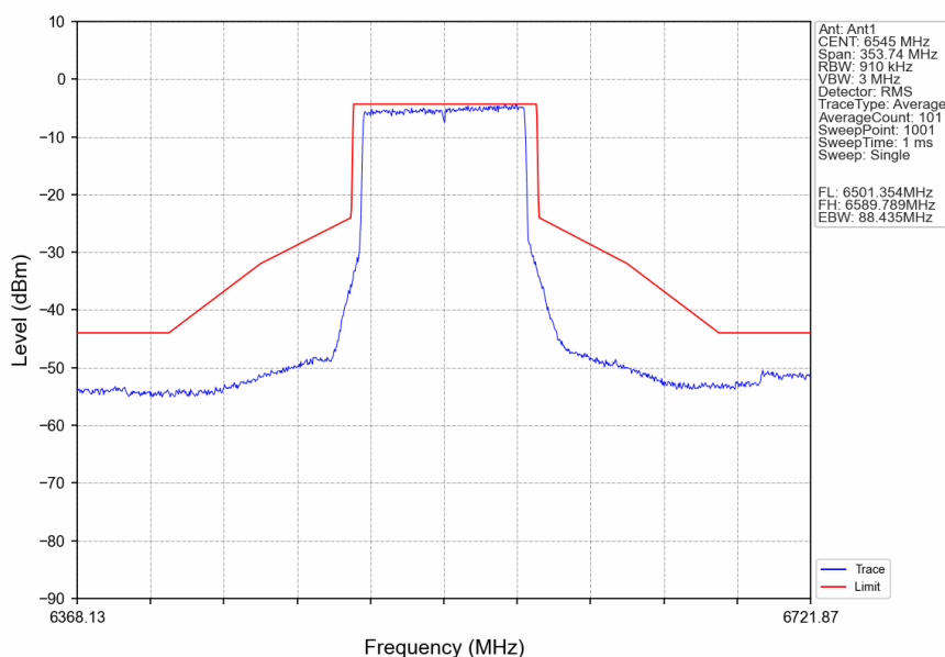
802.11ax(HEW80)_HCH_6545MHz_RU996_Left_Ant1_NTNV
