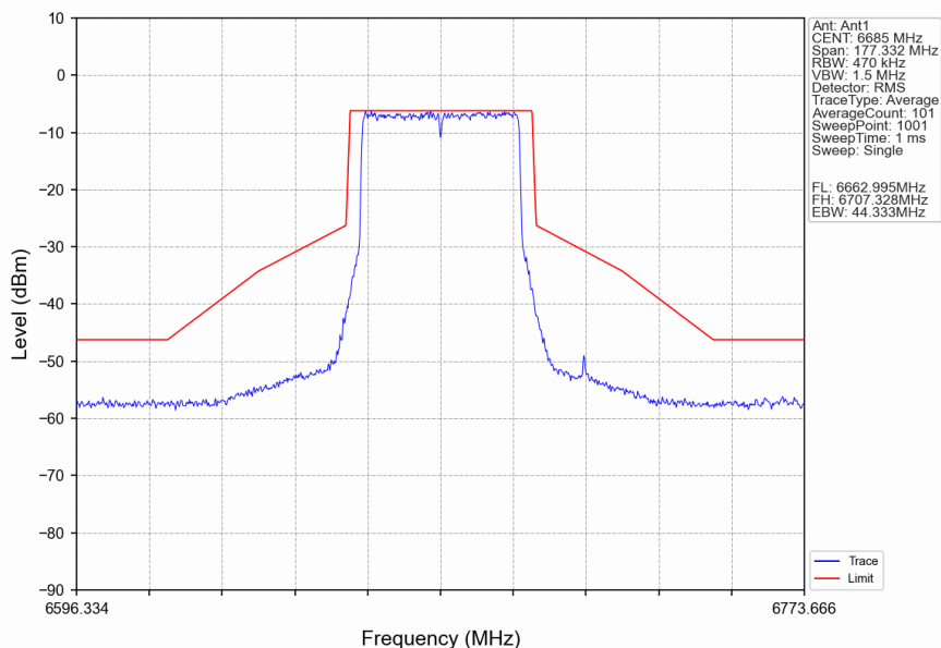
802.11ax(HEW40)_MCH_6685MHz_RU484_Left_Ant1_NTNV
