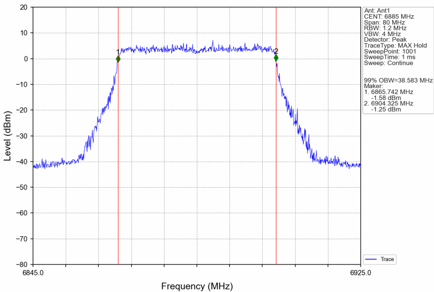
802.11be(EHT40)_HCH_6885MHz_RU484_Left_Ant1_NTNV
