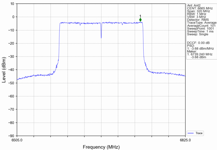
802.11be(EHT160)_MCH_6665MHz_2xRU996_Left_Ant2_NTNV
