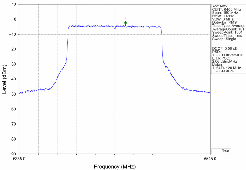
802.11ax(HEW80)_LCH_6465MHz_RU996_Left_Ant2_NTNV
