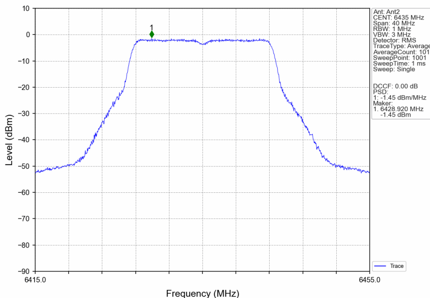
802.11a_LCH_6435MHz_Ant2_NTNV
