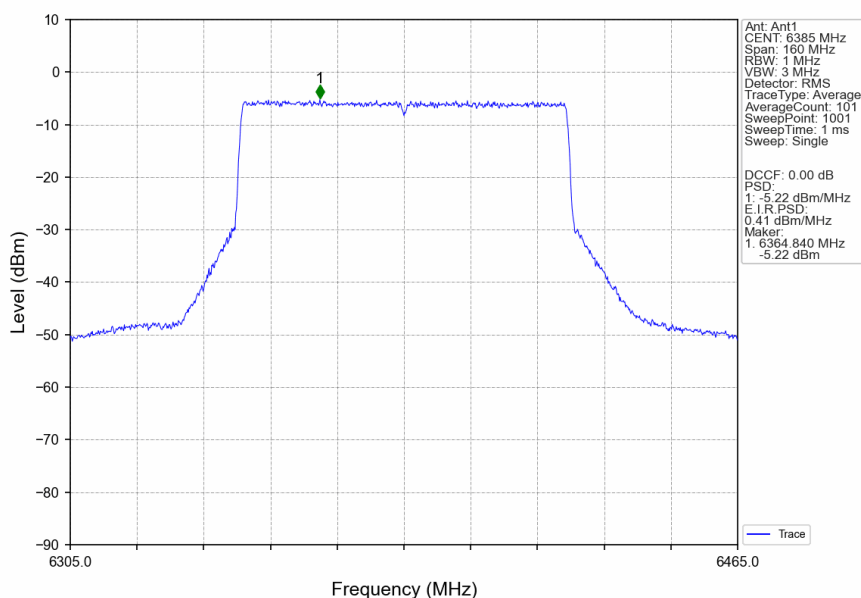
802.11ax(HEW80)_HCH_6385MHz_RU996_Left_Ant1_NTNV
