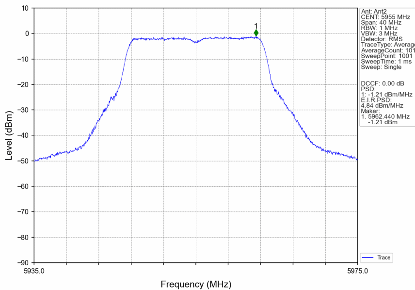
802.11a_LCH_5955MHz_Ant2_NTNV
