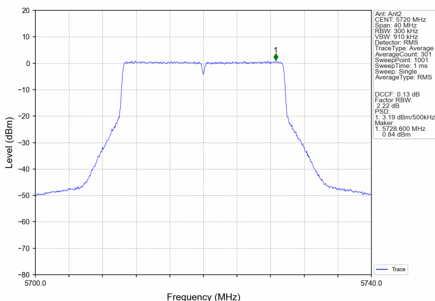
802.11be(EHT20)_HCH_5720MHz_SU_ / _Ant2_NTNV
