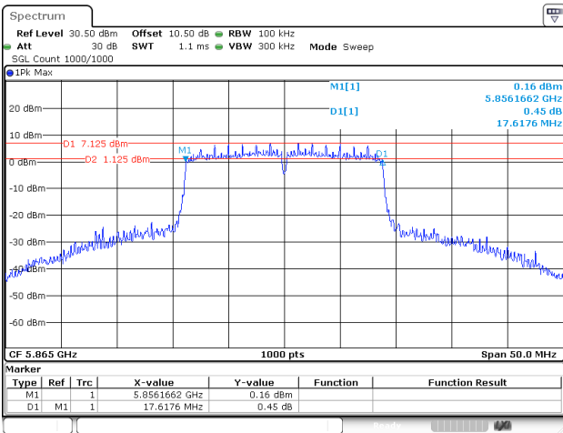
802.11ac20_5865MHz_Chain 2
