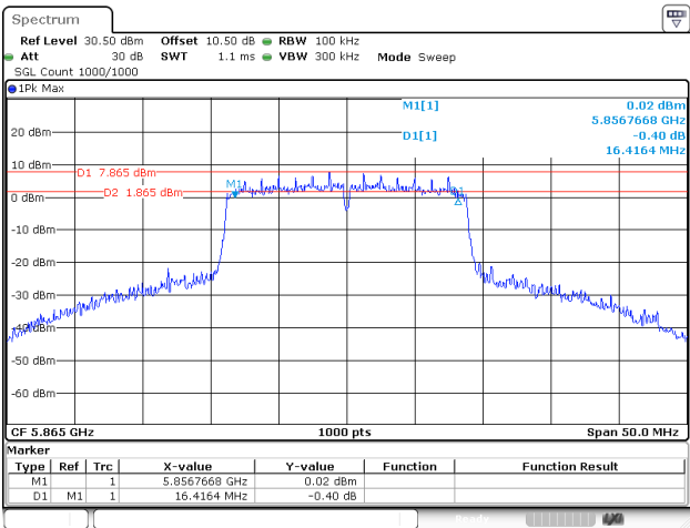
802.11ac20_5865MHz_Chain 0
