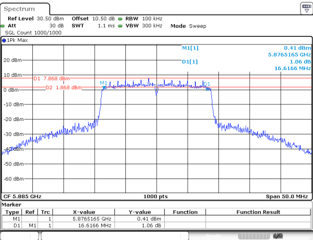
802.11ac20_5885MHz_Chain 0
