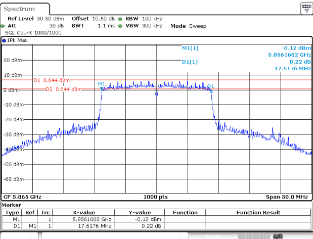
802.11ac20_5865MHz_Chain 1
