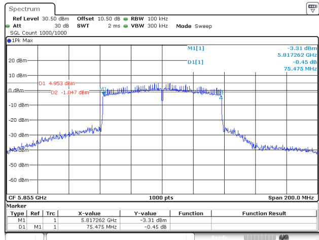
802.11ac80_5855MHz_Chain 1
