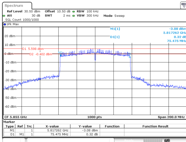
802.11ac80_5855MHz_Chain 2
