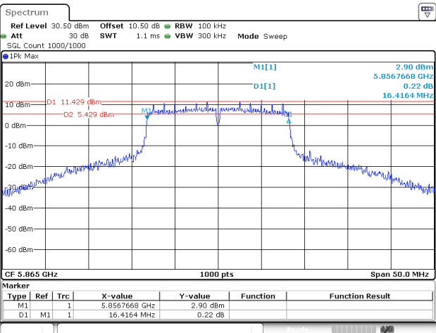
802.11a_5865MHz_Chain 2
