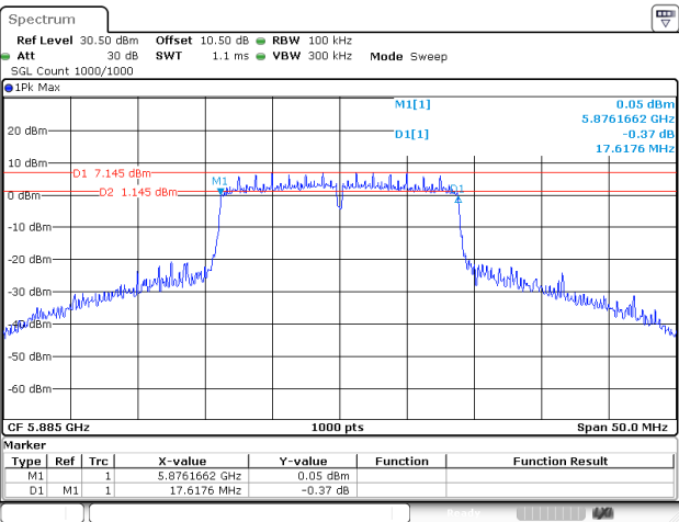
802.11ac20_5885MHz_Chain 2
