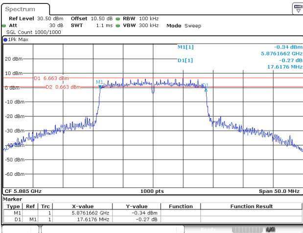
802.11ac20_5885MHz_Chain 1
