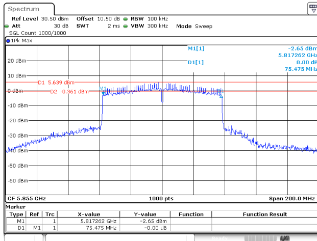
802.11ac80_5855MHz_Chain 0
