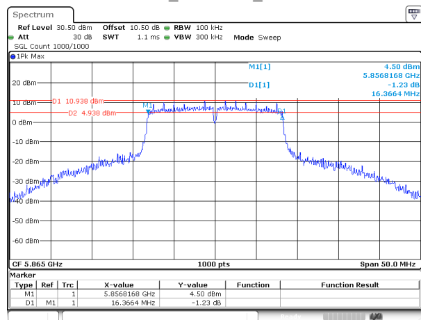
802.11a_5865MHz_Chain 1
