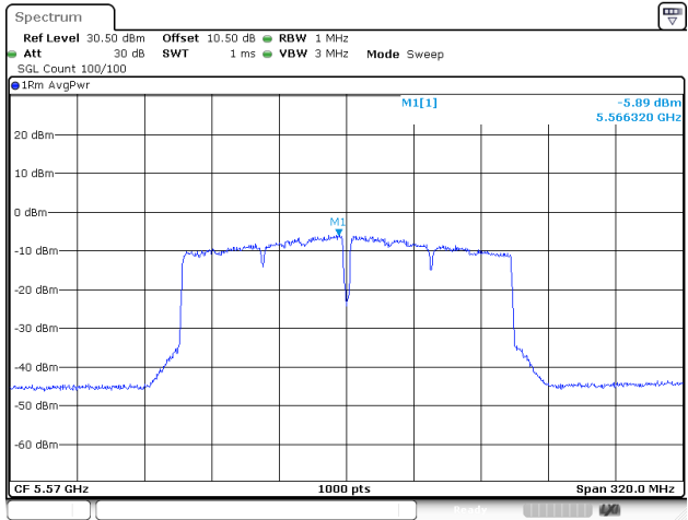
802.11ac160_5570MHz_Chain 0
