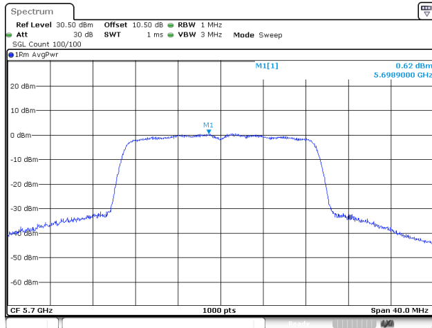
802.11ac20_5700MHz_Chain 1
