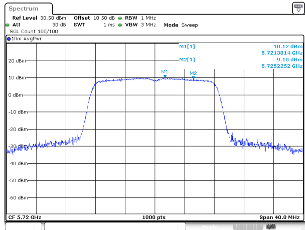
802.11a_5720MHz_Chain 0
