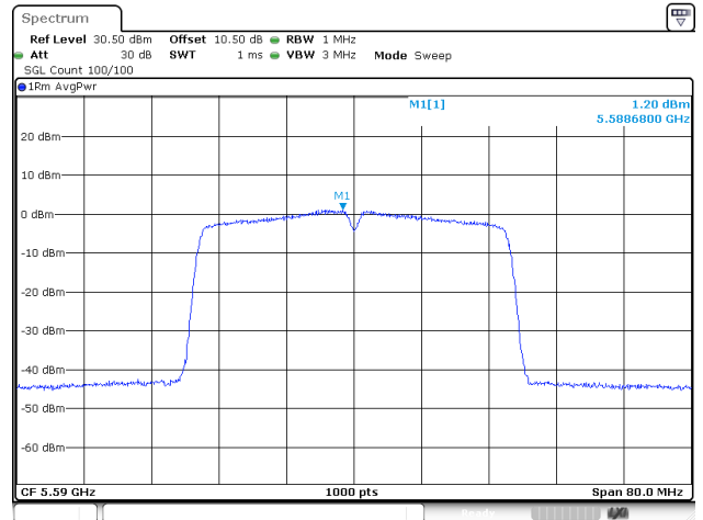
802.11ac40_5590MHz_Chain 0
