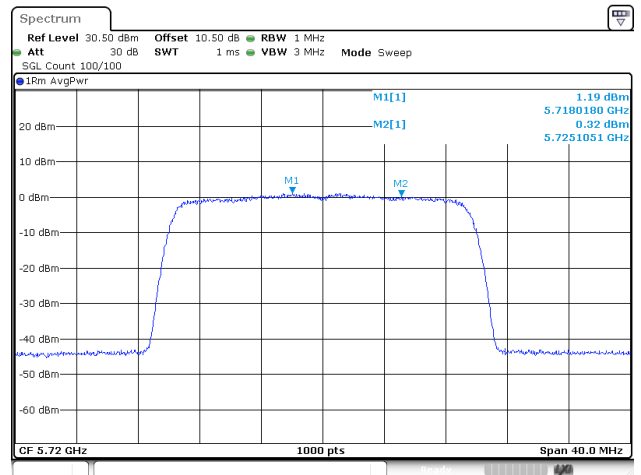
802.11be20_5720MHz_RU_Full_Chain 0
