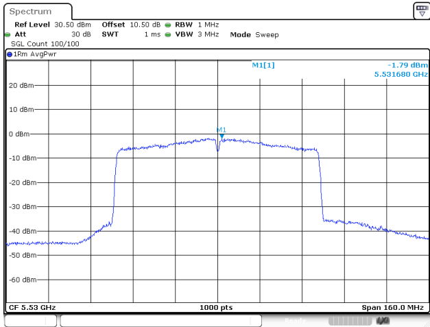
802.11ac80_5530MHz_Chain 0
