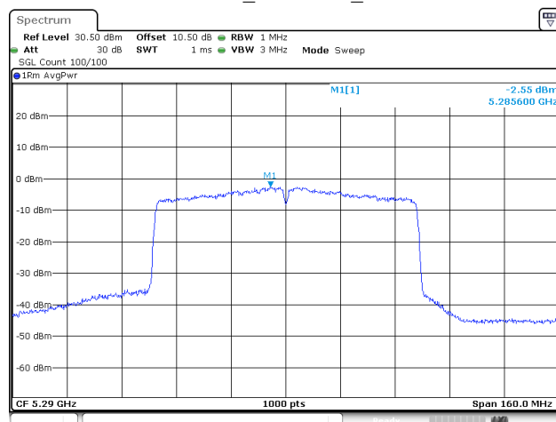
802.11ac80_5290MHz_Chain 0
