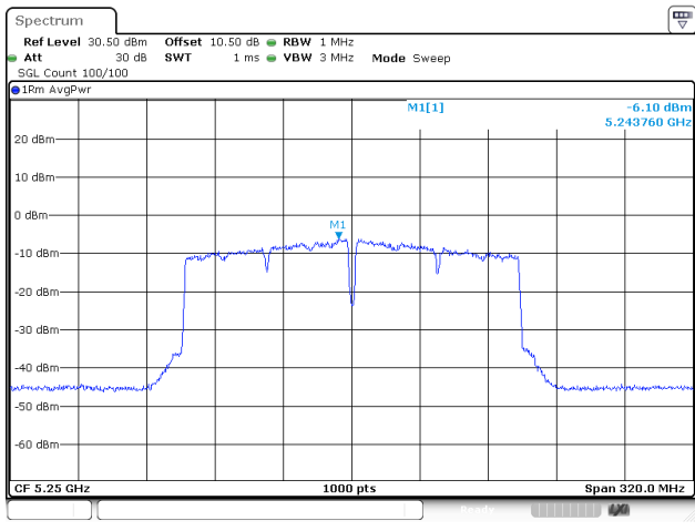
802.11ac160_5250MHz_Chain 2
