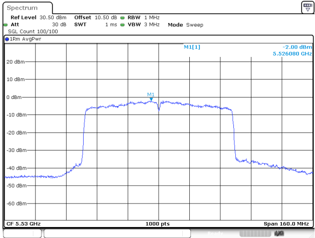
802.11ac80_5530MHz_Chain 1
