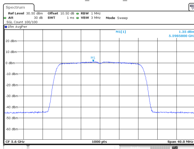
802.11ac20_5600MHz_Chain 0
