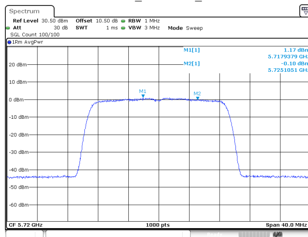
802.11ac20_5720MHz_Chain 0
