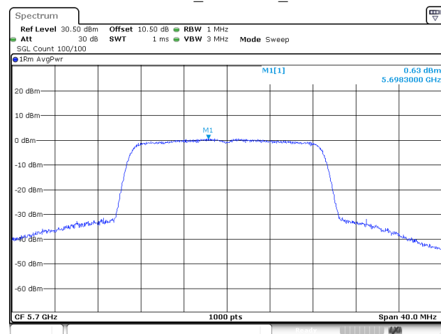
802.11ac20_5700MHz_Chain 0
