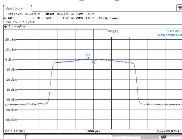
802.11ac40_5270MHz_Chain 2
