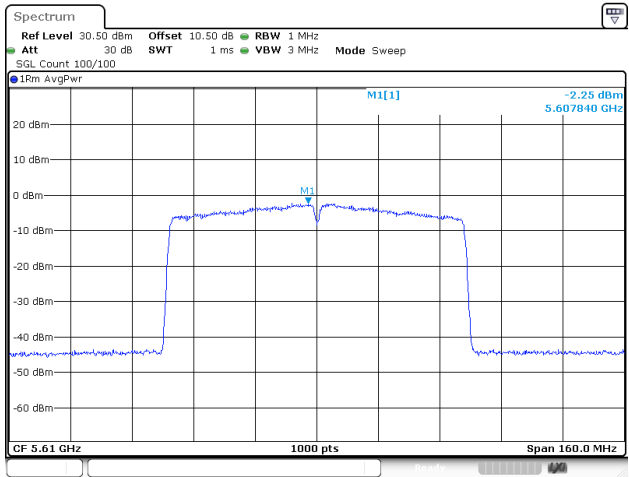
802.11ac80_5610MHz_Chain 2
