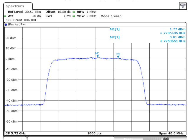
802.11be20_5720MHz_RU_Full_Chain 2
