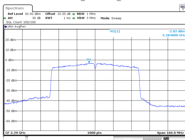
802.11ac80_5290MHz_Chain 2
