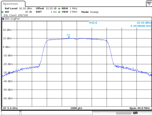
802.11a_5500MHz_Chain 2
