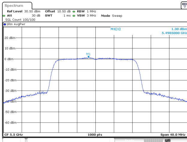
802.11ac20_5500MHz_Chain 2
