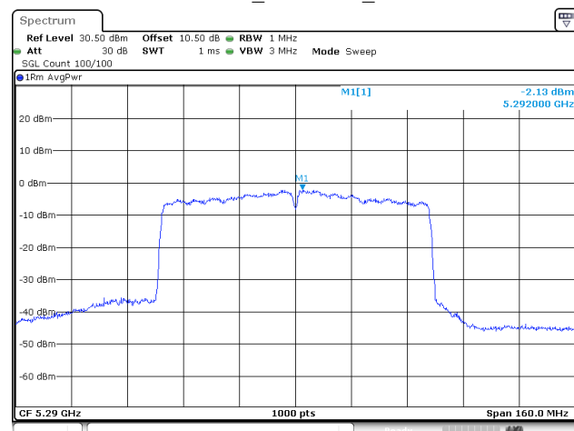
802.11ac80_5290MHz_Chain 1
