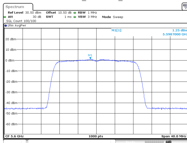
802.11ac20_5600MHz_Chain 1
