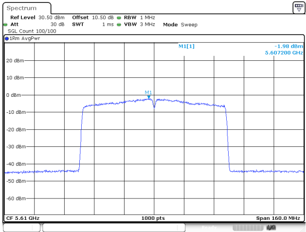
802.11ac80_5610MHz_Chain 0
