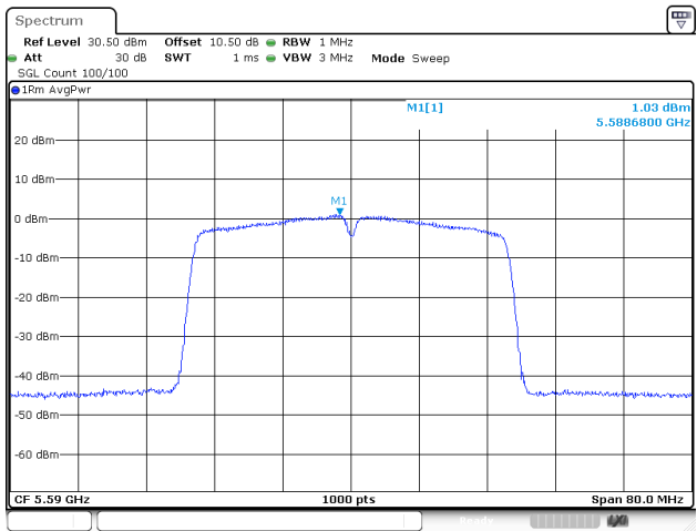
802.11ac40_5590MHz_Chain 2
