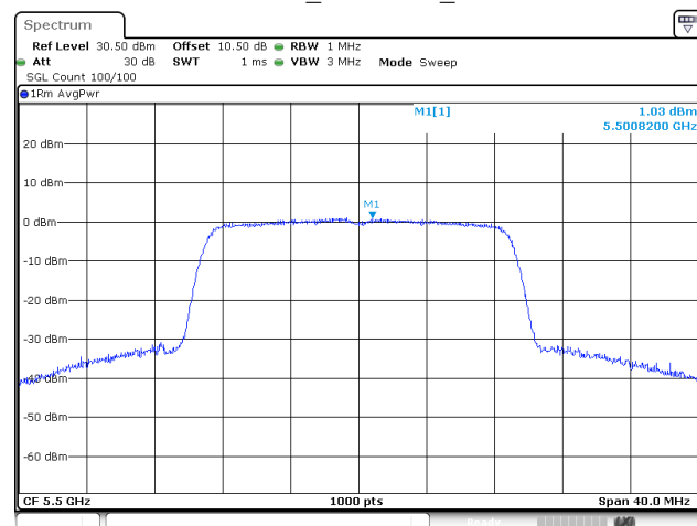
802.11ac20_5500MHz_Chain 1
