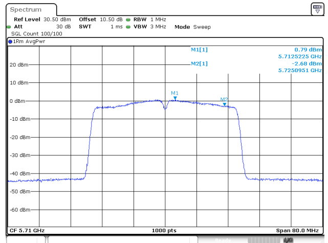
802.11ac40_5710MHz_Chain 0
