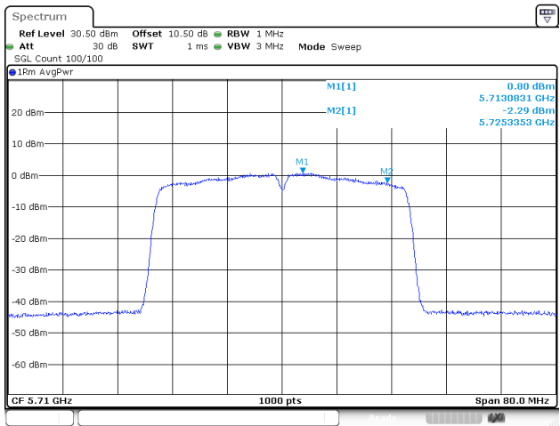
802.11ac40_5710MHz_Chain 2
