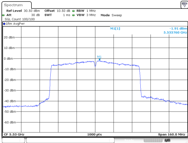
802.11ac80_5530MHz_Chain 2
