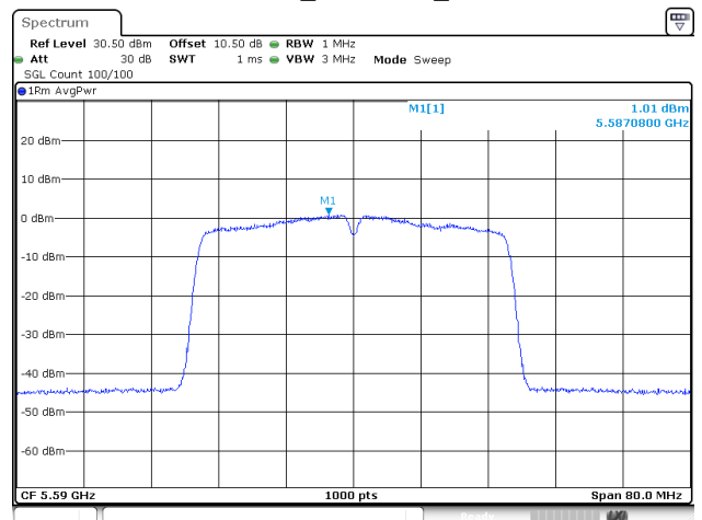
802.11ac40_5590MHz_Chain 1
