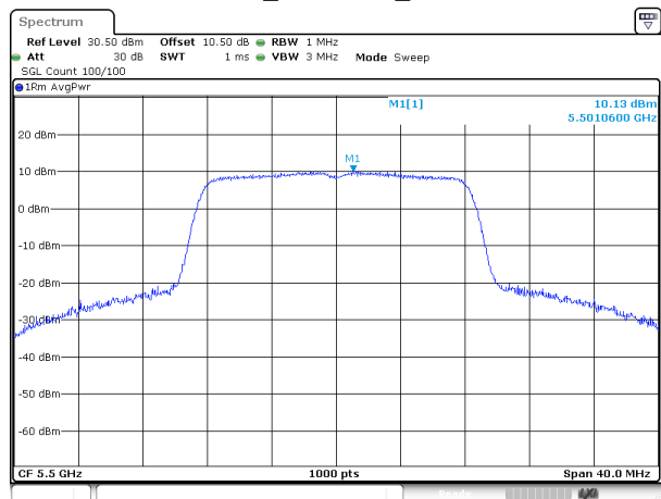
802.11a_5500MHz_Chain 1
