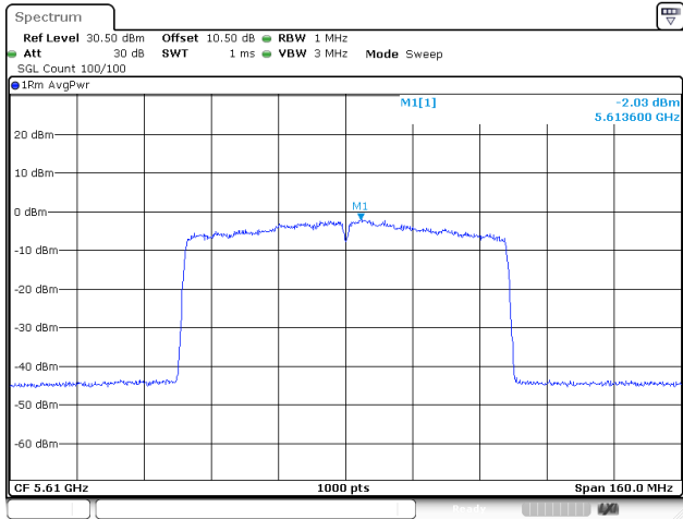
802.11ac80_5610MHz_Chain 1
