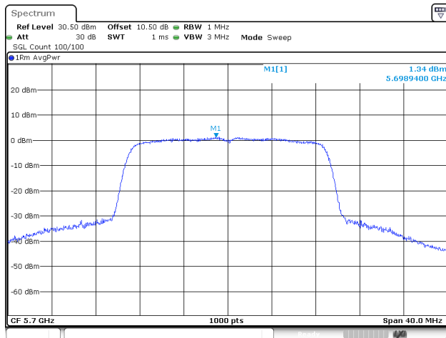
802.11ac20_5700MHz_Chain 2
