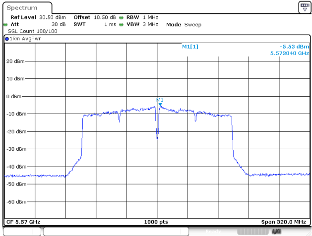
802.11ac160_5570MHz_Chain 2
