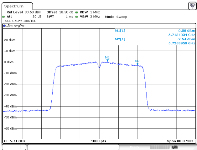
802.11ac40_5710MHz_Chain 1
