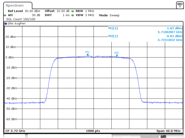
802.11ac20_5720MHz_Chain 2
