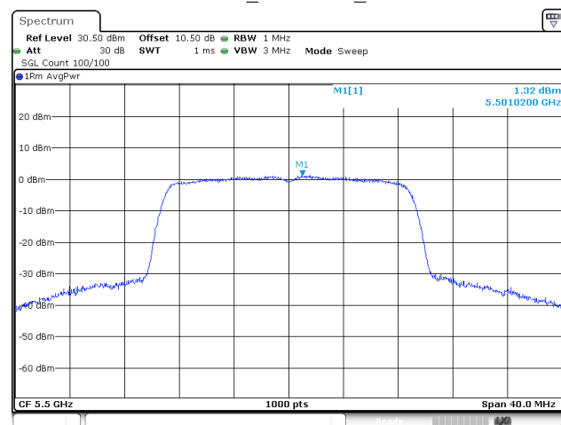
802.11ac20_5500MHz_Chain 0
