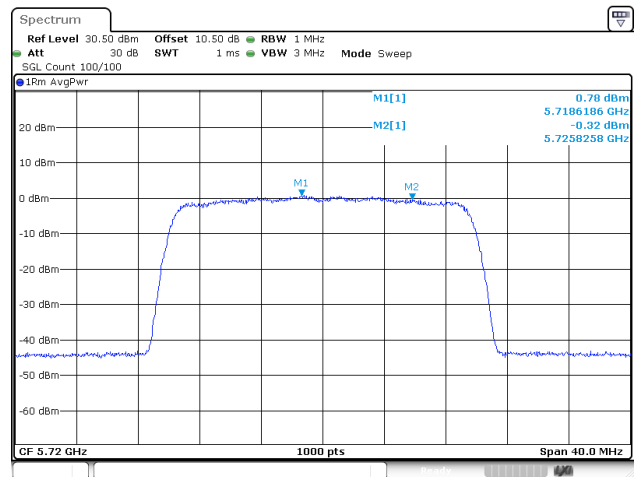
802.11be20_5720MHz_RU_Full_Chain 1
