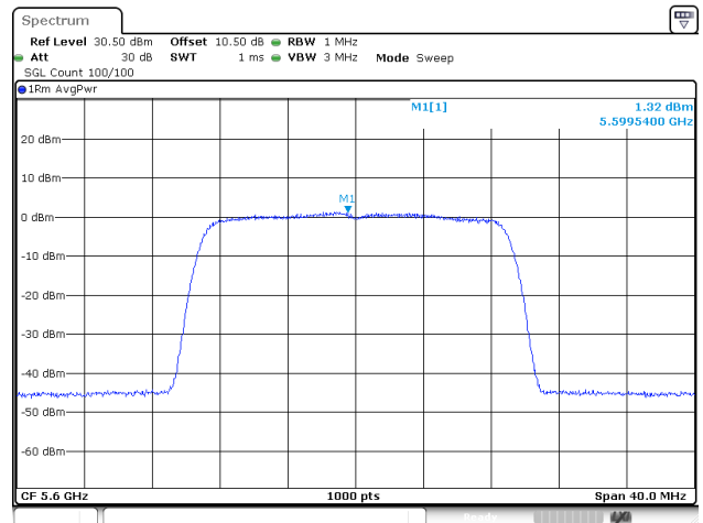
802.11ac20_5600MHz_Chain 2
