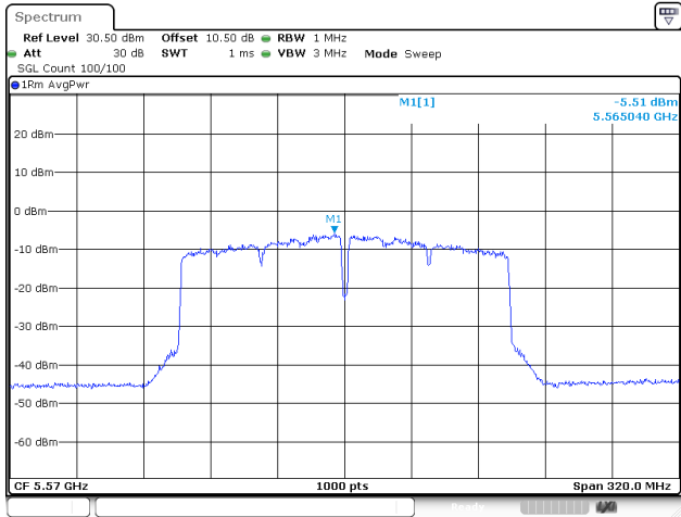
802.11ac160_5570MHz_Chain 1
