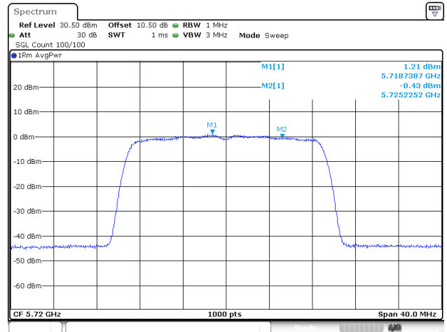
802.11ac20_5720MHz_Chain 1
