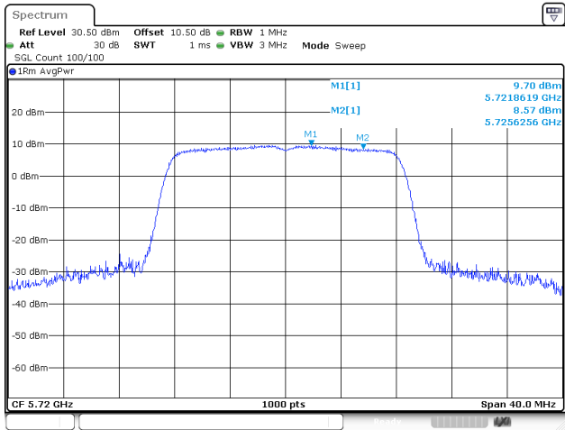
802.11a_5720MHz_Chain 1
