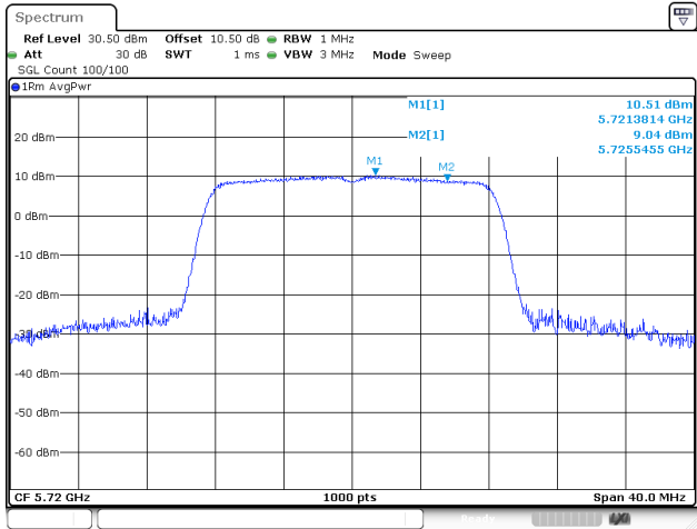
802.11a_5720MHz_Chain 2
