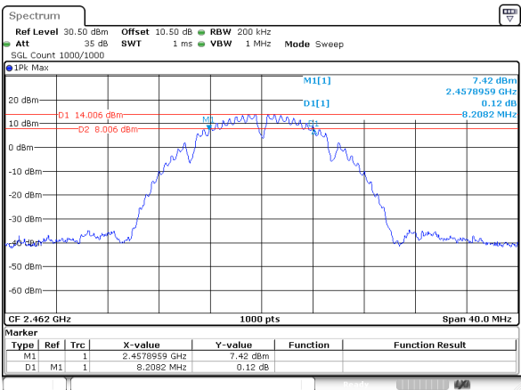
802.11b_2462MHz_Chain 1
