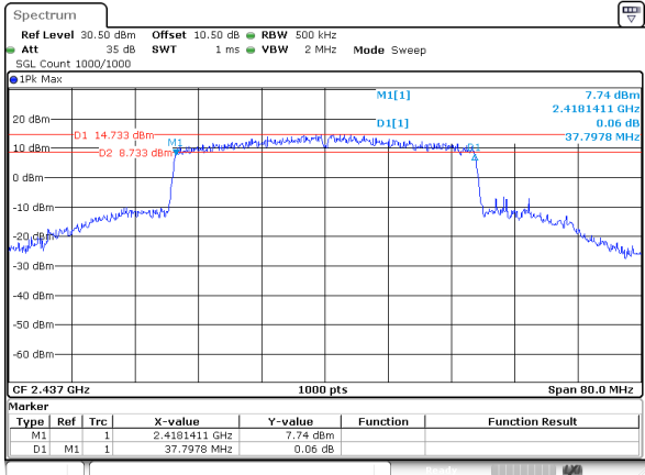
802.11be40_RU_Full_2437MHz_Chain 1
