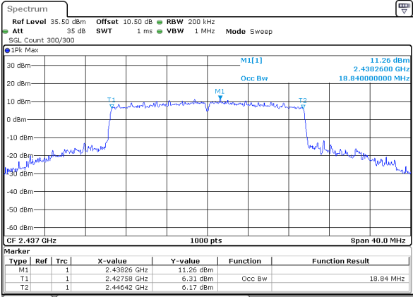
802.11be20_RU_Full_2437MHz_Chain 0
