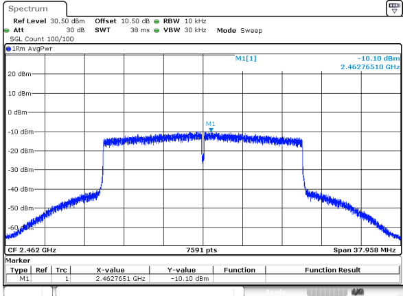
802.11be20_RU_Full_2462MHz_Chain 0
