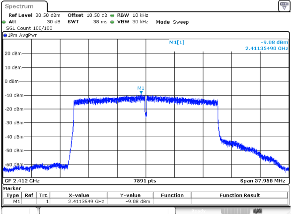
802.11be20_RU_Full_2412MHz_Chain 1
