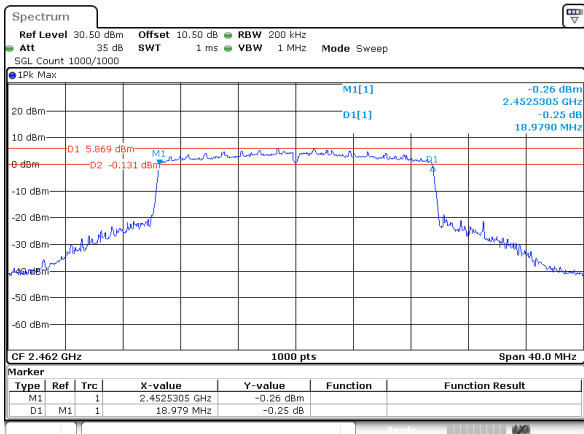
802.11be20_RU_Full_2462MHz_Chain 0
