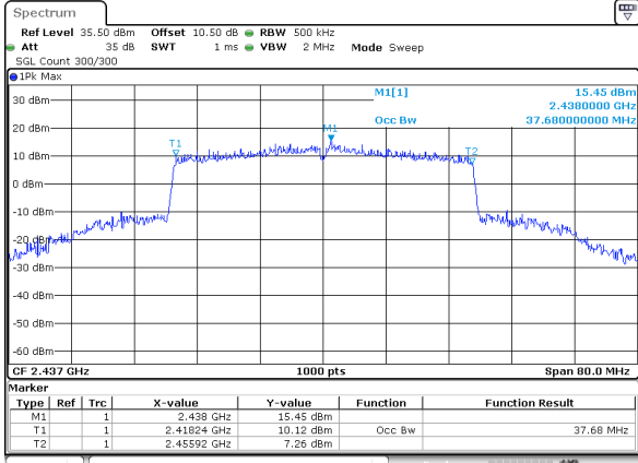
802.11be40_RU_Full_2437MHz_Chain 1
