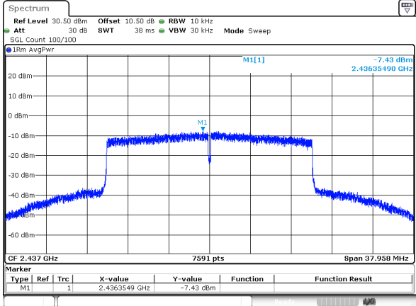
802.11be20_RU_Full_2437MHz_Chain 1
