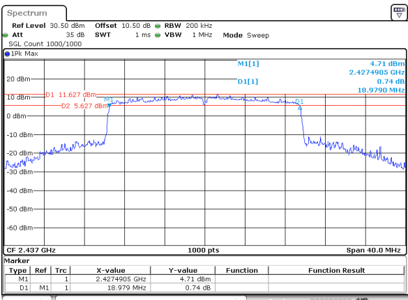
802.11be20_RU_Full_2437MHz_Chain 0
