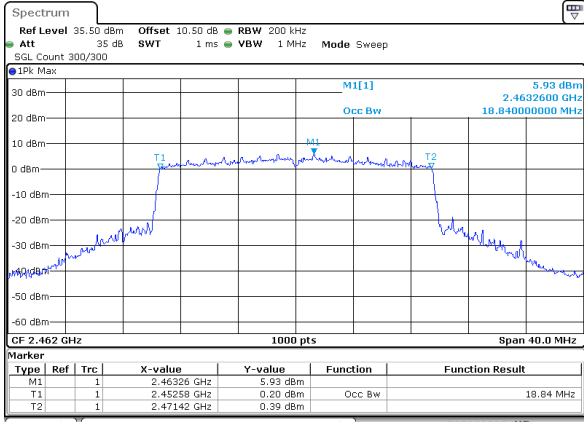
802.11be20_RU_Full_2462MHz_Chain 0
