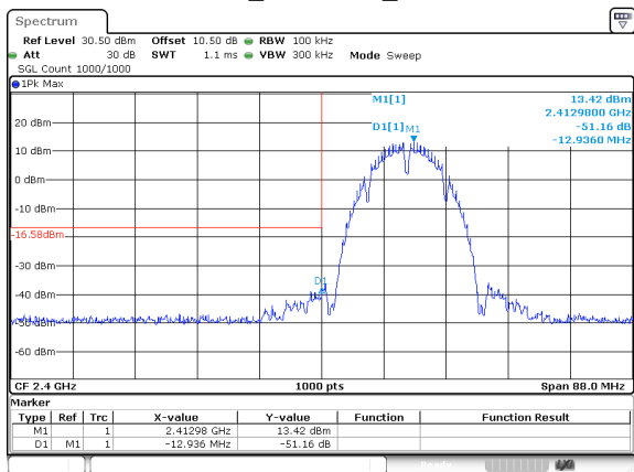
802.11b_2412MHz_Chain 1
