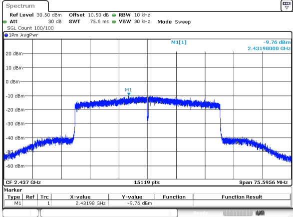
802.11be40_RU_Full_2437MHz_Chain 1
