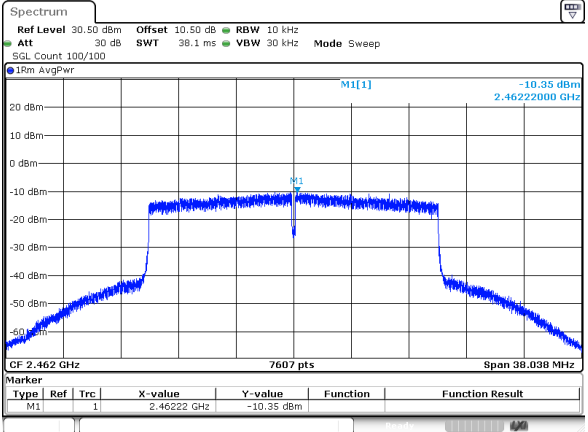
802.11be20_RU_Full_2462MHz_Chain 1
