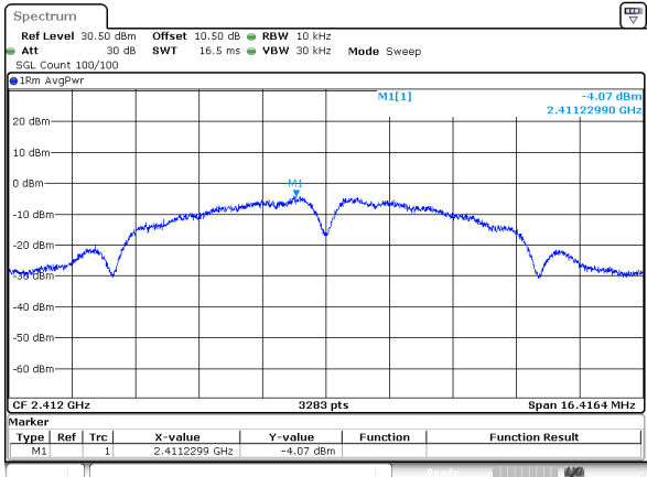
802.11b_2412MHz_Chain 0
