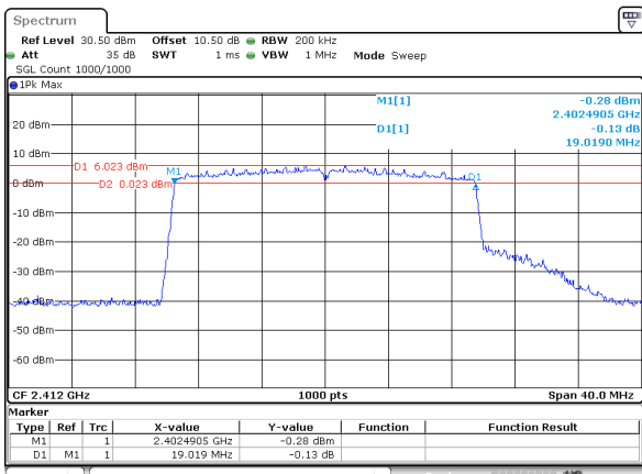
802.11be20_RU_Full_2412MHz_Chain 0
