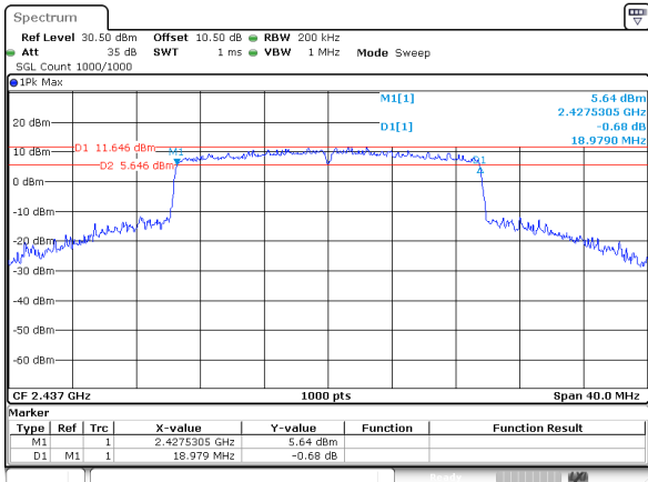
802.11be20_RU_Full_2437MHz_Chain 1
