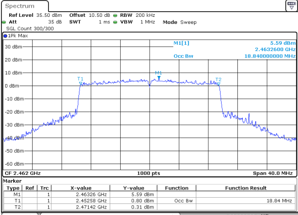
802.11be20_RU_Full_2462MHz_Chain 1
