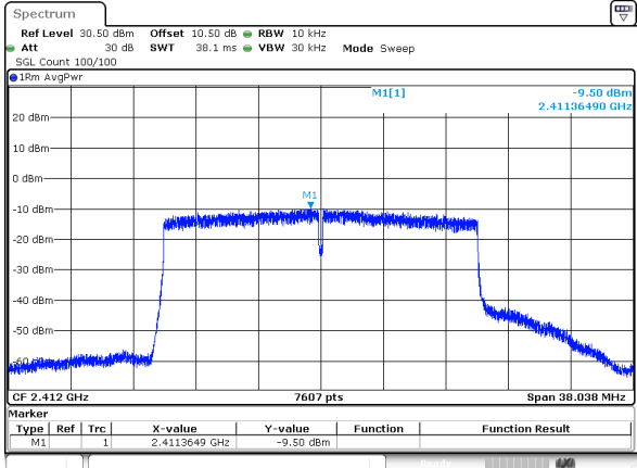
802.11be20_RU_Full_2412MHz_Chain 0
