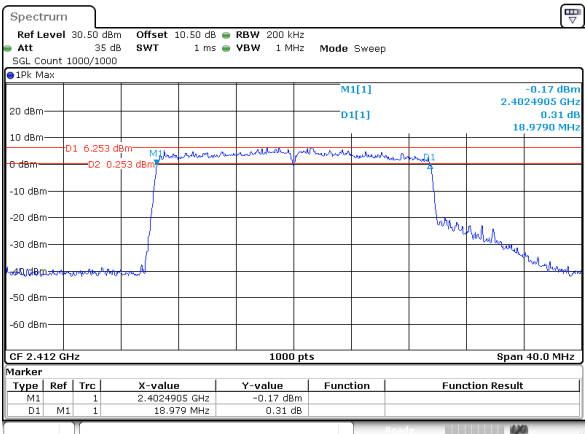
802.11be20_RU_Full_2412MHz_Chain 1
