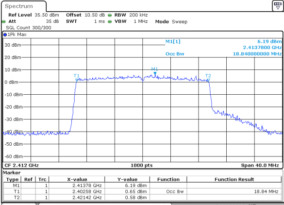
802.11be20_RU_Full_2412MHz_Chain 1
