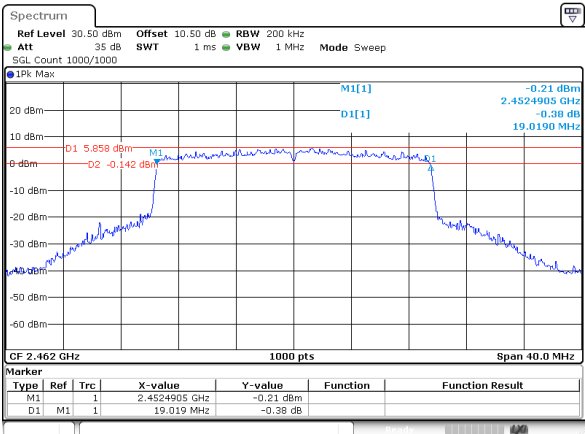
802.11be20_RU_Full_2462MHz_Chain 1
