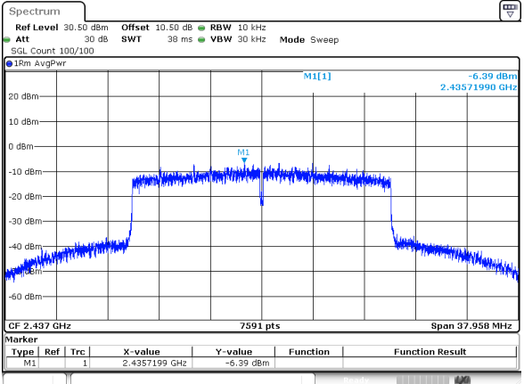
802.11be20_RU_Full_2437MHz_Chain 0
