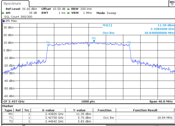
802.11be20_RU_Full_2437MHz_Chain 1
