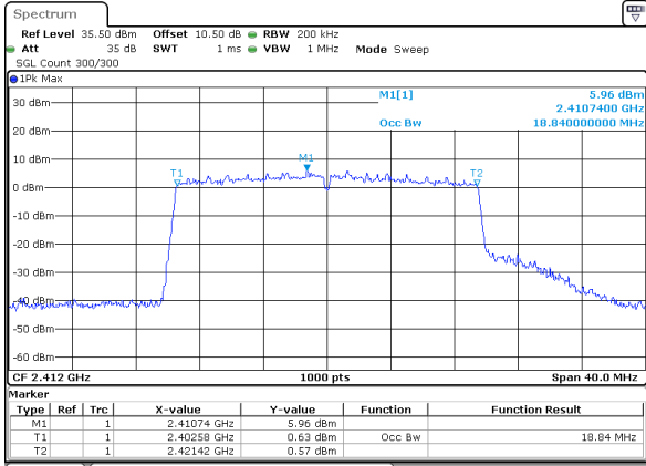
802.11be20_RU_Full_2412MHz_Chain 0
