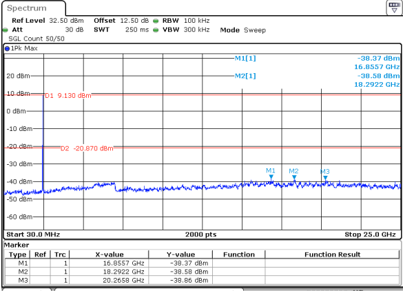
802.11be20_2462MHz_Chain 1
