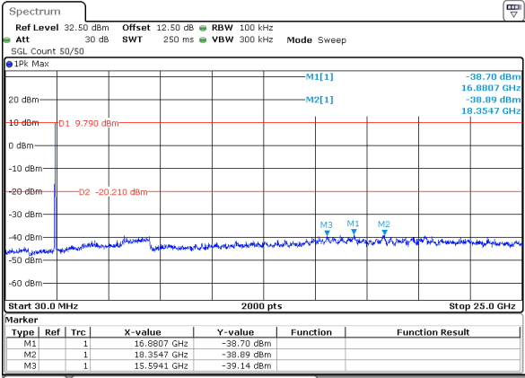
802.11be20_2437MHz_Chain 0
