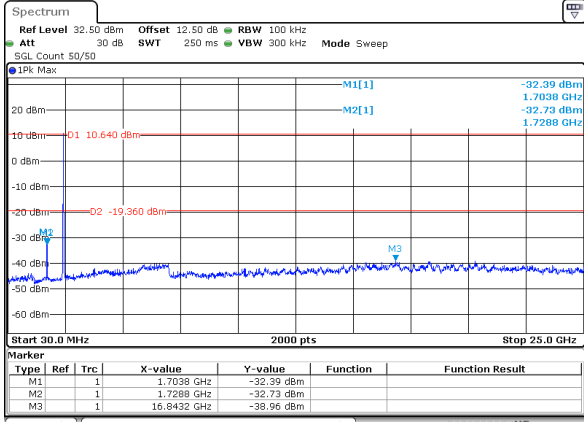
802.11be20_2437MHz_Chain 1
