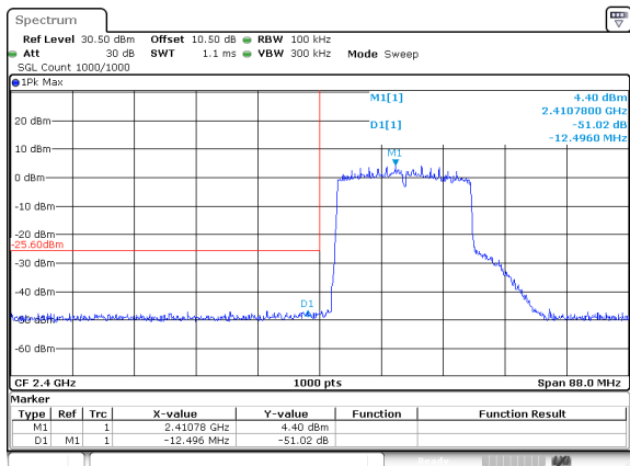
802.11be20_2412MHz_Chain 1
