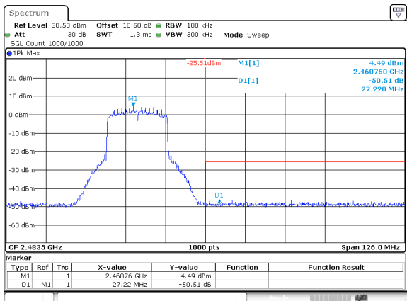
802.11be20_2462MHz_Chain 1
