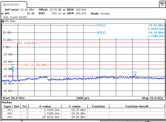
802.11be40_2452MHz_Chain 1
