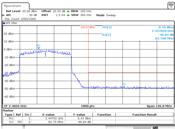
802.11be40_2452MHz_Chain 1
