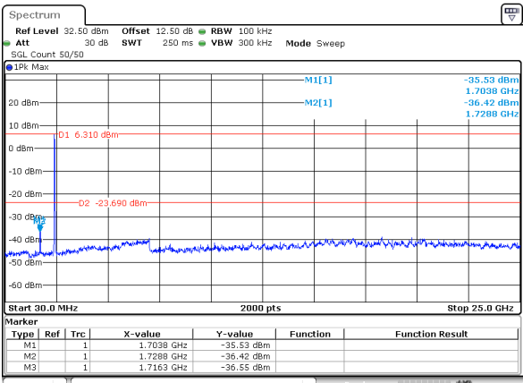
802.11be40_2422MHz_Chain 1
