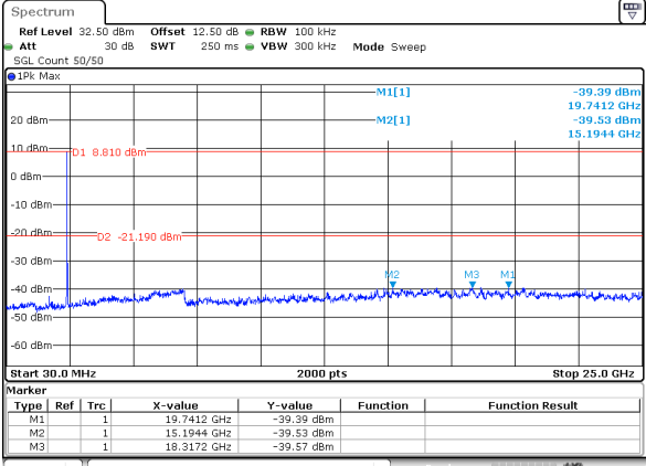
802.11be20_2412MHz_Chain 1
