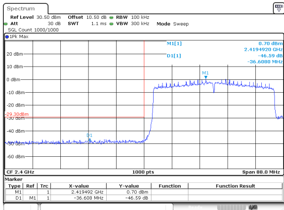
802.11be40_2422MHz_Chain 0
