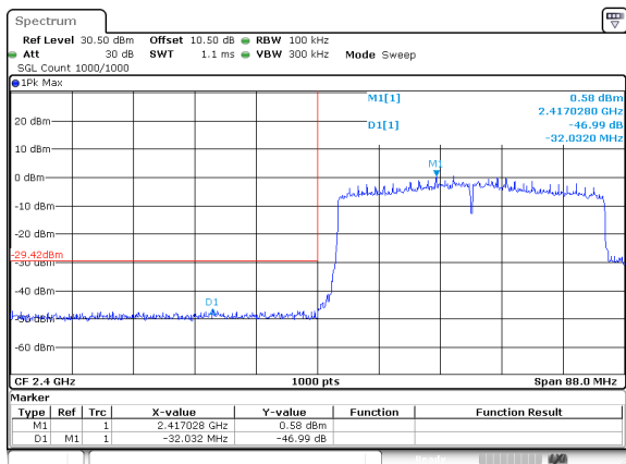
802.11be40_2422MHz_Chain 1
