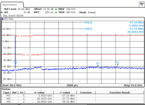
802.11be40_2437MHz_Chain 0
