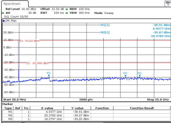
802.11be20_2412MHz_Chain 0
