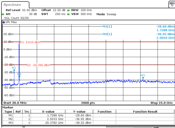
802.11be40_2437MHz_Chain 1
