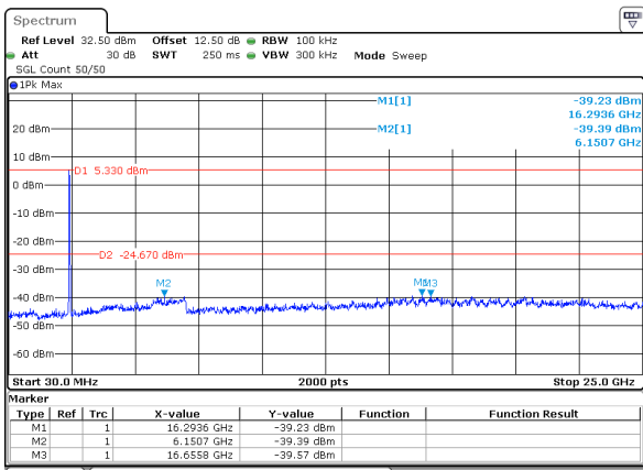
802.11be40_2422MHz_Chain 0
