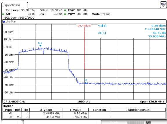
802.11be40_2452MHz_Chain 0
