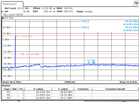
802.11be40_2452MHz_Chain 0
