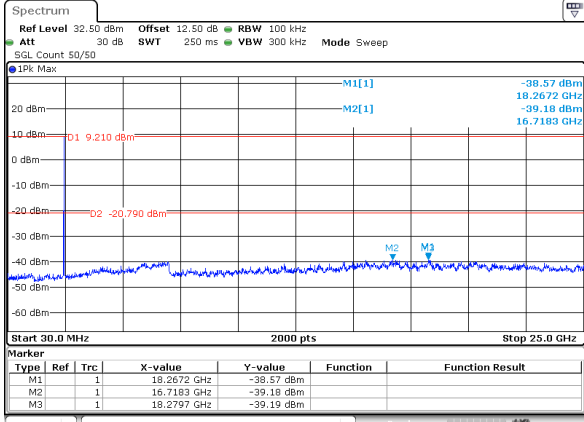
802.11be20_2462MHz_Chain 0
