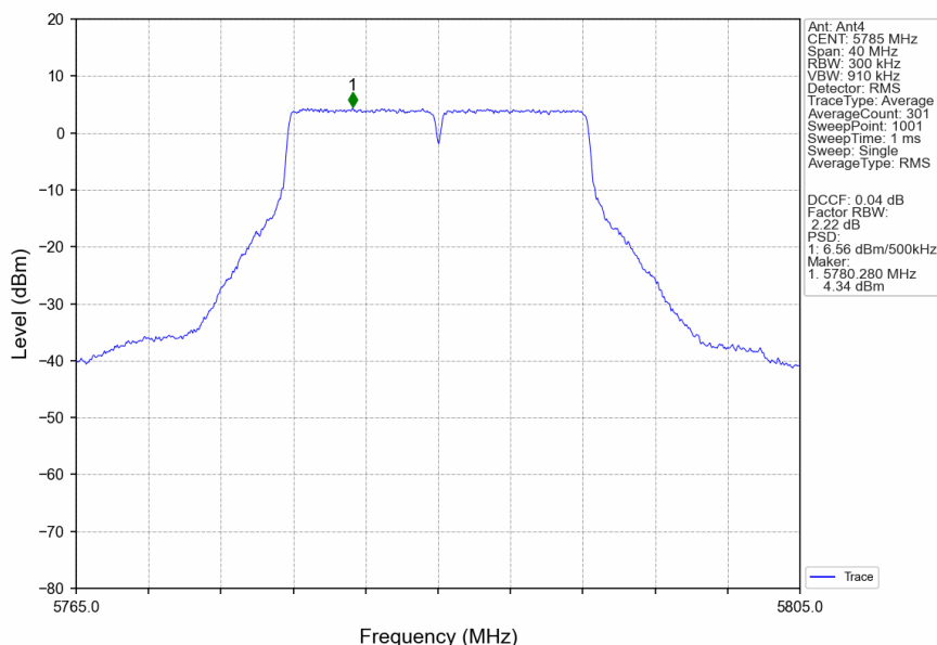
802.11a_MCH_5785MHz_Ant4_NTNV
