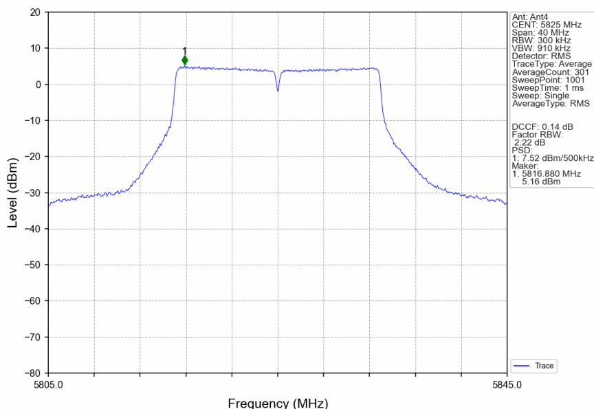
802.11n(HT20)_HCH_5825MHz_Ant4_NTNV
