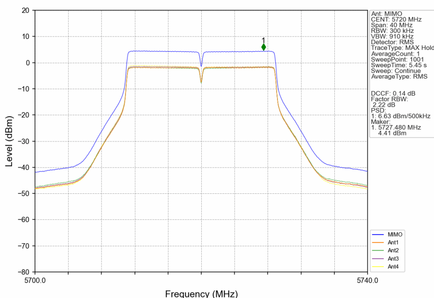
802.11n(HT20)_HCH_5720MHz_MIMO_NTNV
