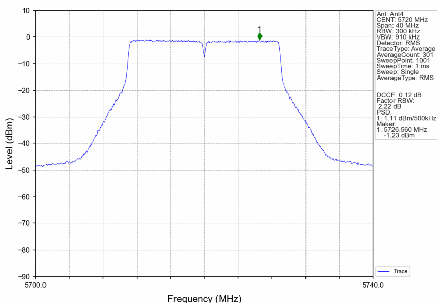
802.11ac(VHT20)_HCH_5720MHz_Ant4_NTNV
