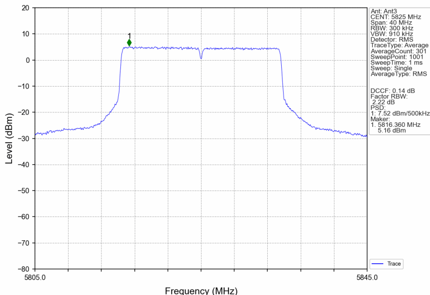
802.11be(EHT20)_HCH_5825MHz_SU_ / _Ant3_NTNV
