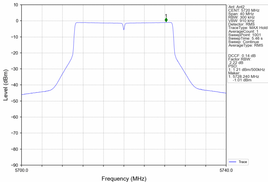
802.11be(EHT20)_HCH_5720MHz_SU_ / _Ant2_NTNV
