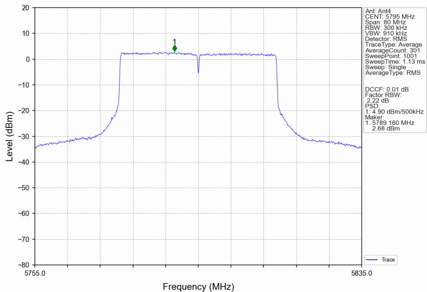
802.11be(EHT40)_HCH_5795MHz_SU_ / _Ant4_NTNV
