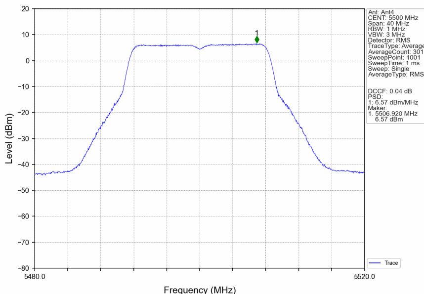
802.11a_LCH_5500MHz_Ant4_NTNV
