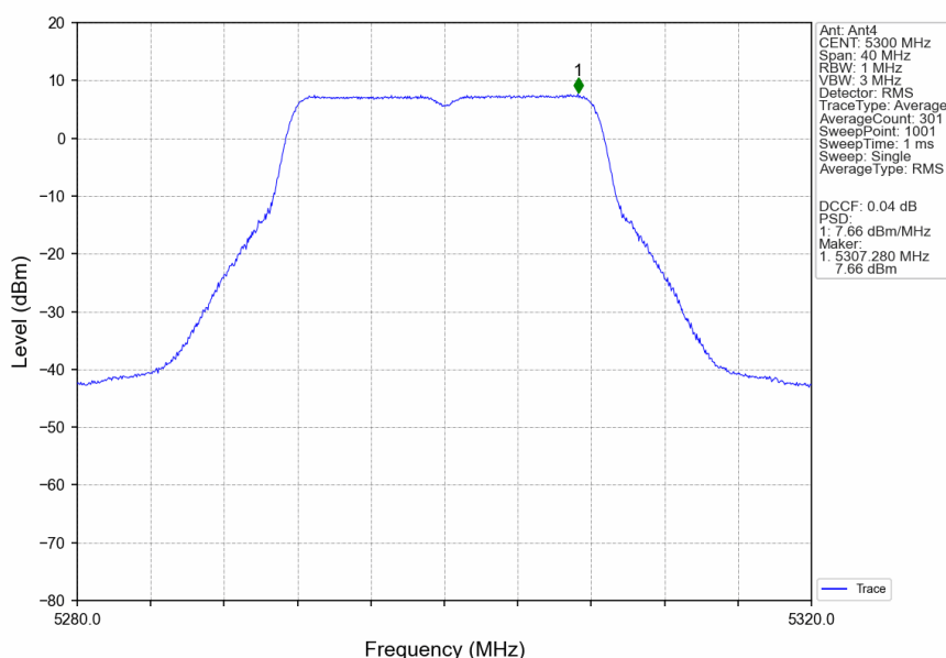
802.11a_MCH_5300MHz_Ant4_NTNV
