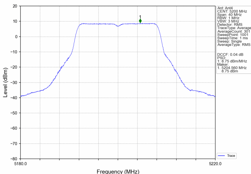
802.11a_MCH_5200MHz_Ant4_NTNV
