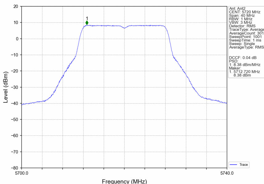
802.11a_HCH_5720MHz_Ant2_NTNV
