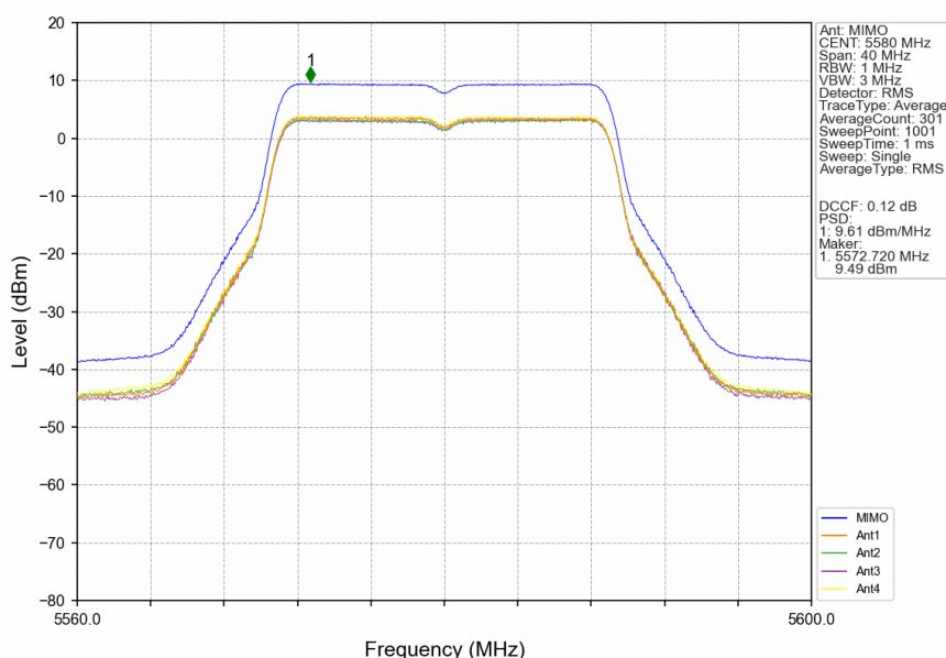
802.11n(HT20)_MCH_5580MHz_MIMO_NTNV
