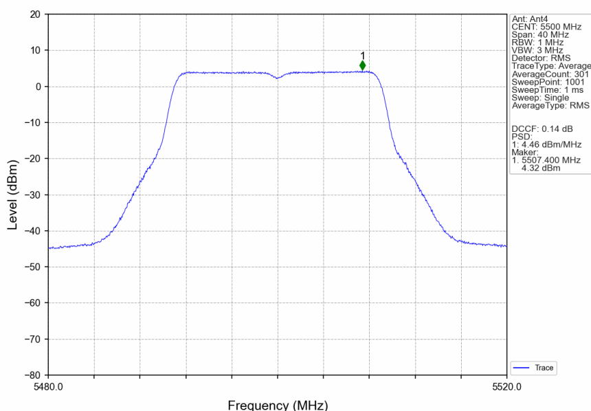
802.11n(HT20)_LCH_5500MHz_Ant4_NTNV
