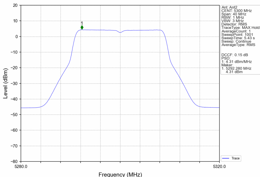
802.11n(HT20)_MCH_5300MHz_Ant2_NTNV
