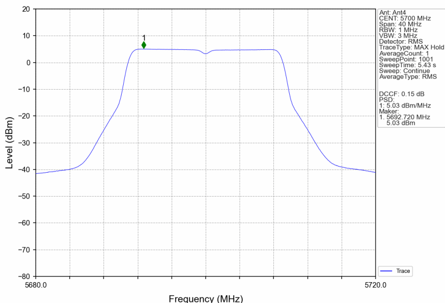
802.11n(HT20)_HCH_5700MHz_Ant4_NTNV
