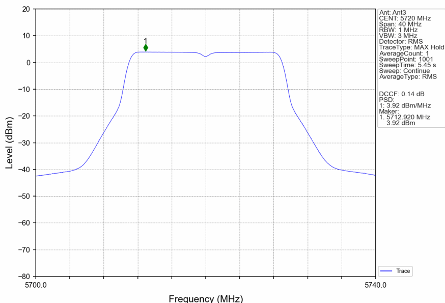
802.11n(HT20)_HCH_5720MHz_Ant3_NTNV
