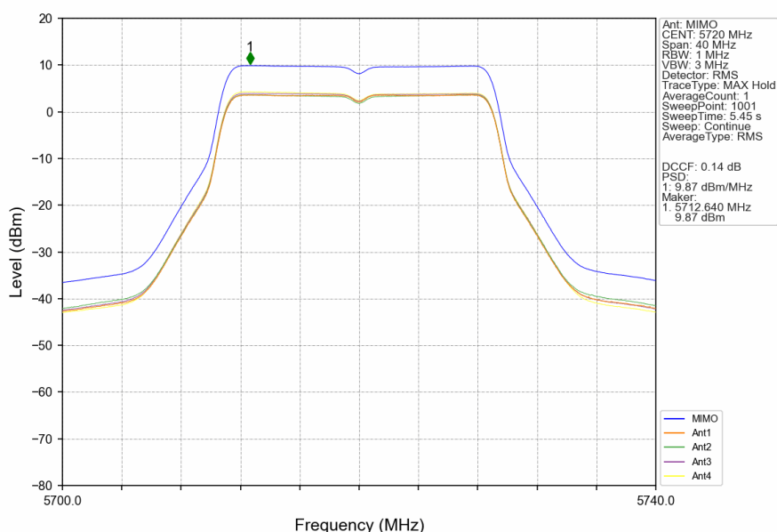
802.11n(HT20)_HCH_5720MHz_MIMO_NTNV
