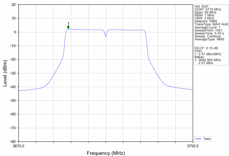
802.11n(HT40)_HCH_5710MHz_Ant1_NTNV
