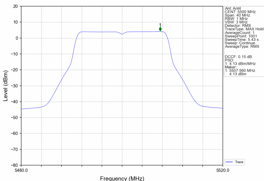
802.11ac(VHT20)_LCH_5500MHz_Ant4_NTNV
