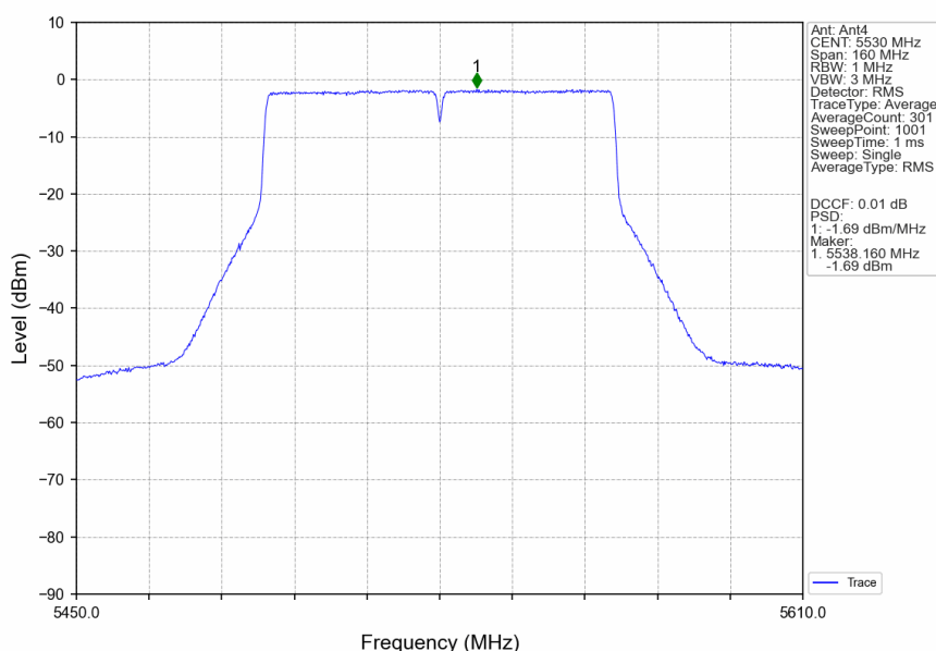
802.11ac(VHT80)_LCH_5530MHz_Ant4_NTNV
