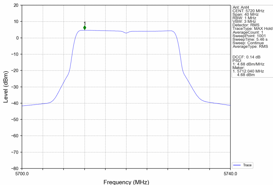
802.11be(EHT20)_HCH_5720MHz_SU_/_MIMO_NTNV
