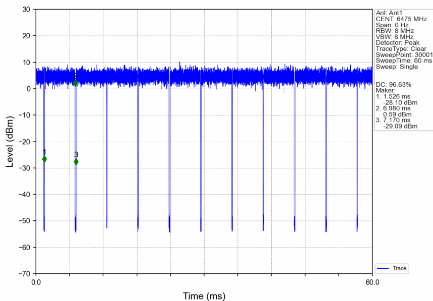
802.11be(EHT20)_MCH_6475MHz_RU242_Left_Ant1_NTNV
