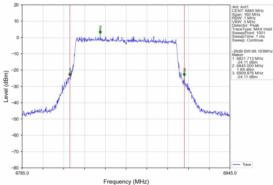
802.11ax(HEW80)_HCH_6865MHz_RU996_Left_Ant1_NTNV
