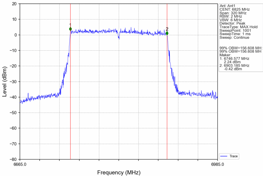
802.11ax(HEW160)_HCH_6825MHz_2xRU996_Left_Ant1_NTNV
