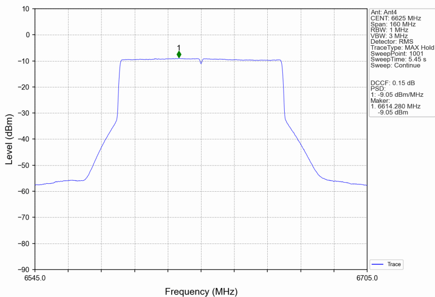
802.11ax(HEW80)_LCH_6625MHz_RU996_Left_Ant4_NTNV
