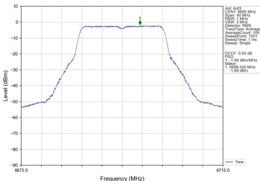
802.11a_MCH_6695MHz_Ant3_NTNV
