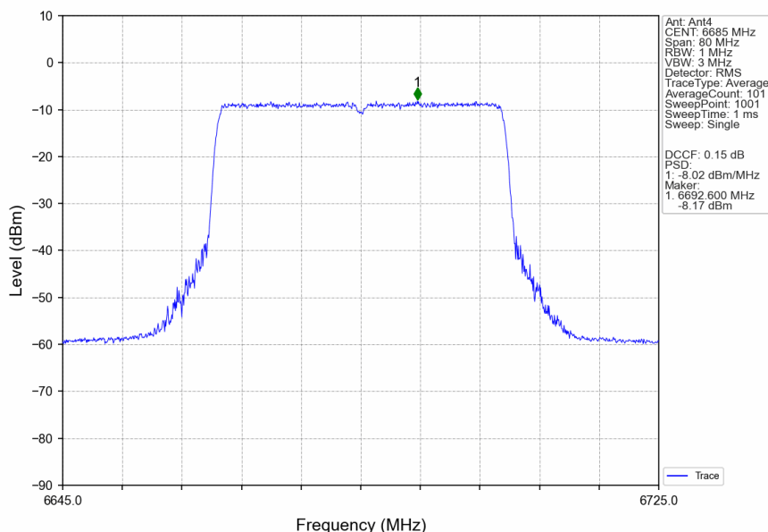
802.11ax(HEW40)_MCH_6685MHz_RU484_Left_Ant4_NTNV
