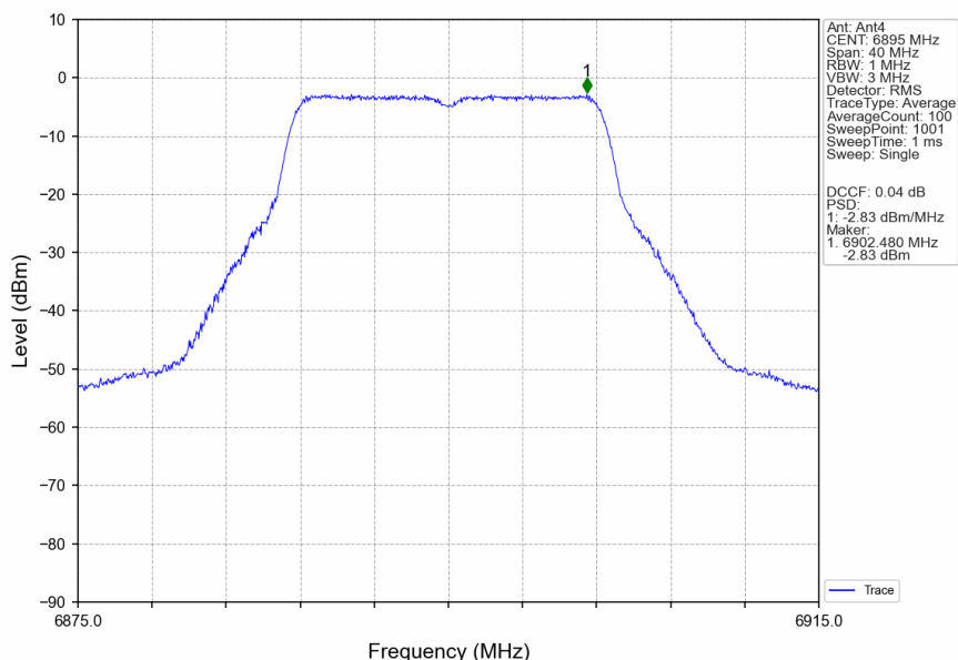
802.11a_LCH_6895MHz_Ant4_NTNV
