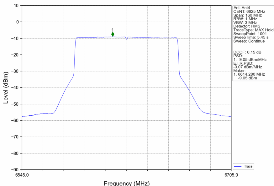
802.11ax(HEW80)_LCH_6625MHz_RU996_Left_Ant4_NTNV
