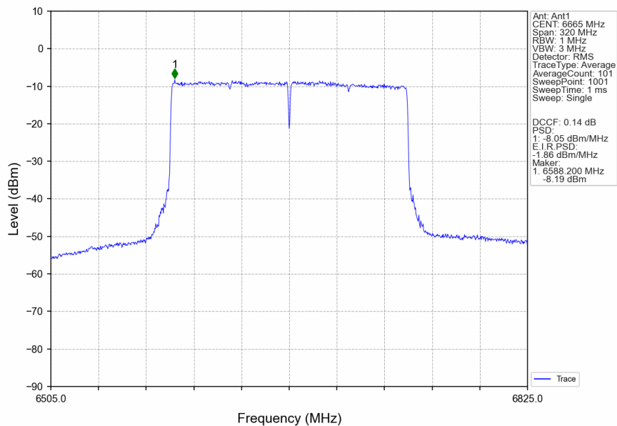
802.11ax(HEW160)_MCH_6665MHz_2xRU996_Left_Ant1_NTNV
