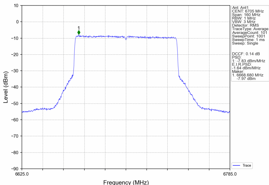
802.11ax(HEW80)_MCH_6705MHz_RU996_Left_Ant1_NTNV
