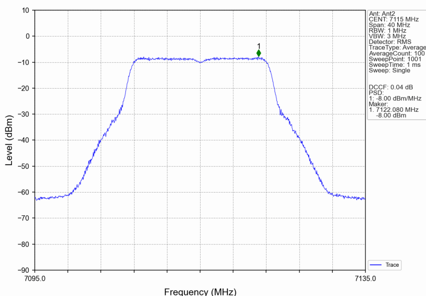
802.11a_HCH_7115MHz_Ant2_NTNV
