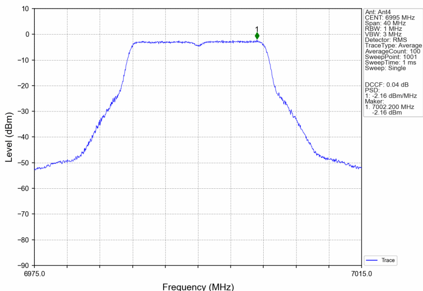
802.11a_MCH_6995MHz_Ant4_NTNV
