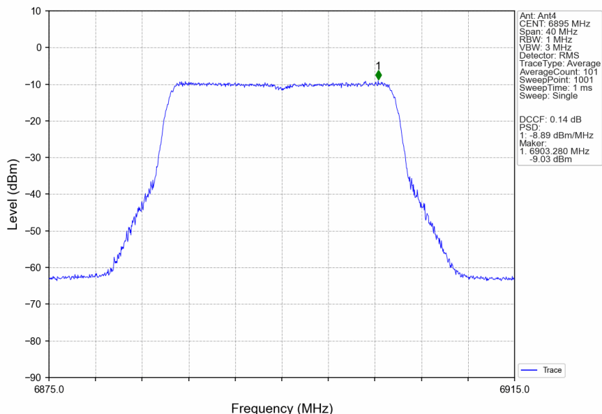
802.11ax(HEW20)_LCH_6895MHz_RU242_Left_Ant4_NTNV
