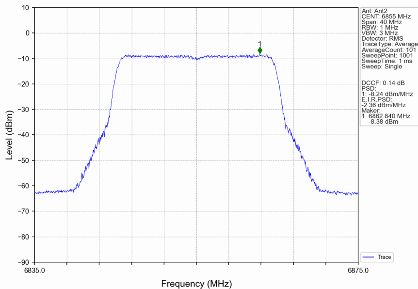
802.11ax(HEW20)_HCH_6855MHz_RU242_Left_Ant2_NTNV
