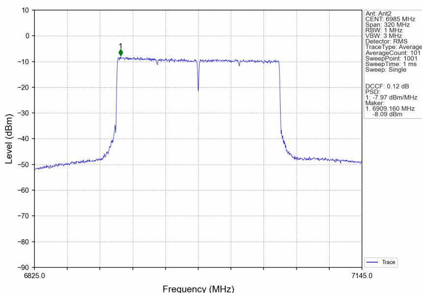
802.11ax(HEW160)_MCH_6985MHz_2xRU996_Left_Ant2_NTNV
