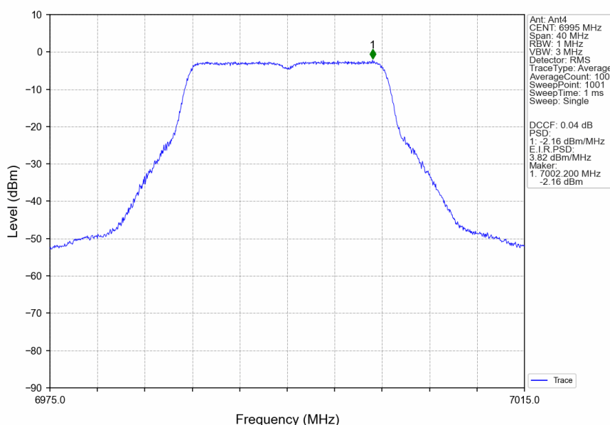
802.11a_MCH_6995MHz_Ant4_NTNV
