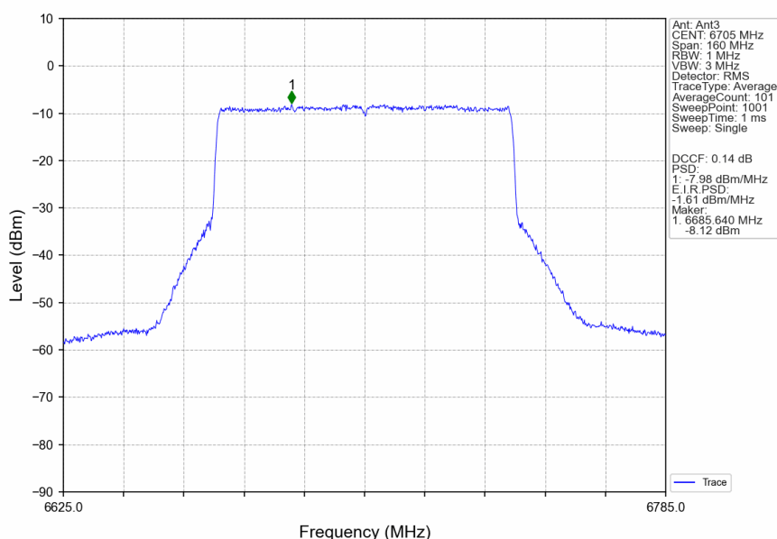
802.11ax(HEW80)_MCH_6705MHz_RU996_Left_Ant3_NTNV
